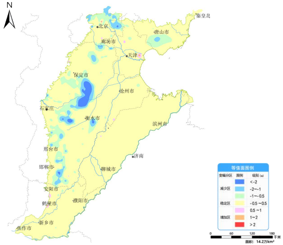
图 11 海河平原 1 月份与上月地下水埋深变幅图
