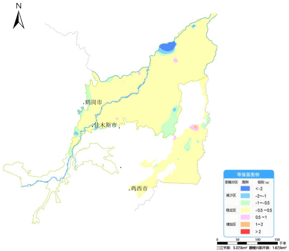
图3 三江平原及穆棱兴凯平原1月份与去年同期地下水埋深变幅图
