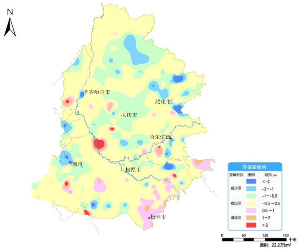
图6 松嫩平原1月份与去年同期地下水埋深变幅图
