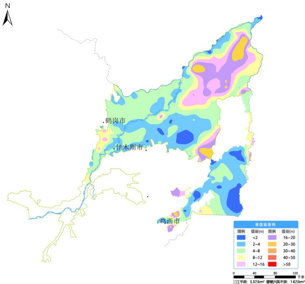
图 1 三江平原及穆棱兴凯平原 1 月份地下水埋深等值面图
