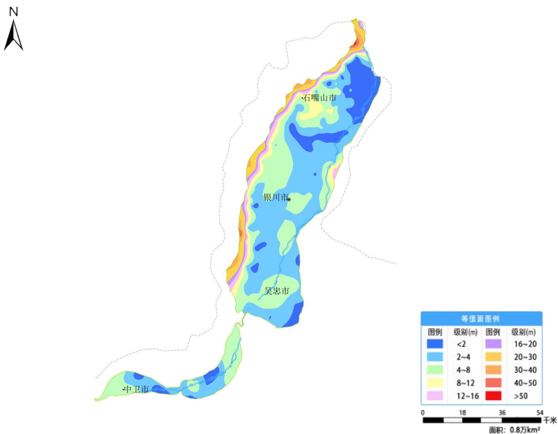
图 25 银川卫宁平原 1 月份地下水埋深等值面图
