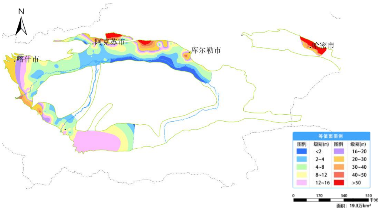
图 27 塔里木盆地监控区 1 月份地下水埋深等值面图
