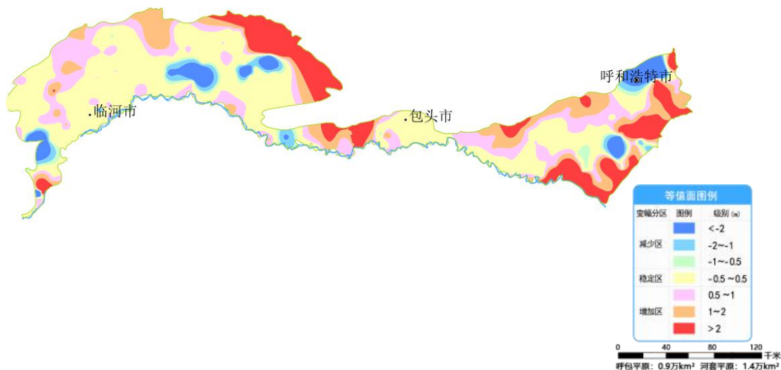
图 18 呼包平原及河套平原 1 月份与去年同期地下水埋深变幅图
