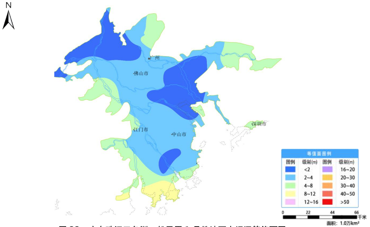
图 33 广东珠江三角洲一般平原 1 月份地下水埋深等值面图
