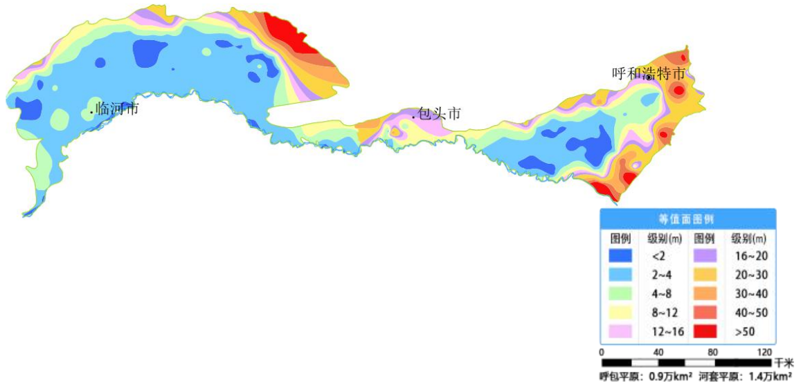
图 16 呼包平原及河套平原 1 月份地下水埋深等值面图
