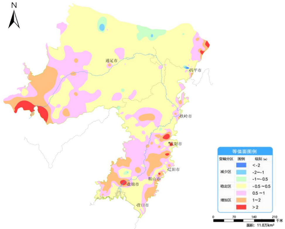
图 9 辽河平原 1 月份与去年同期地下水埋深变幅图
