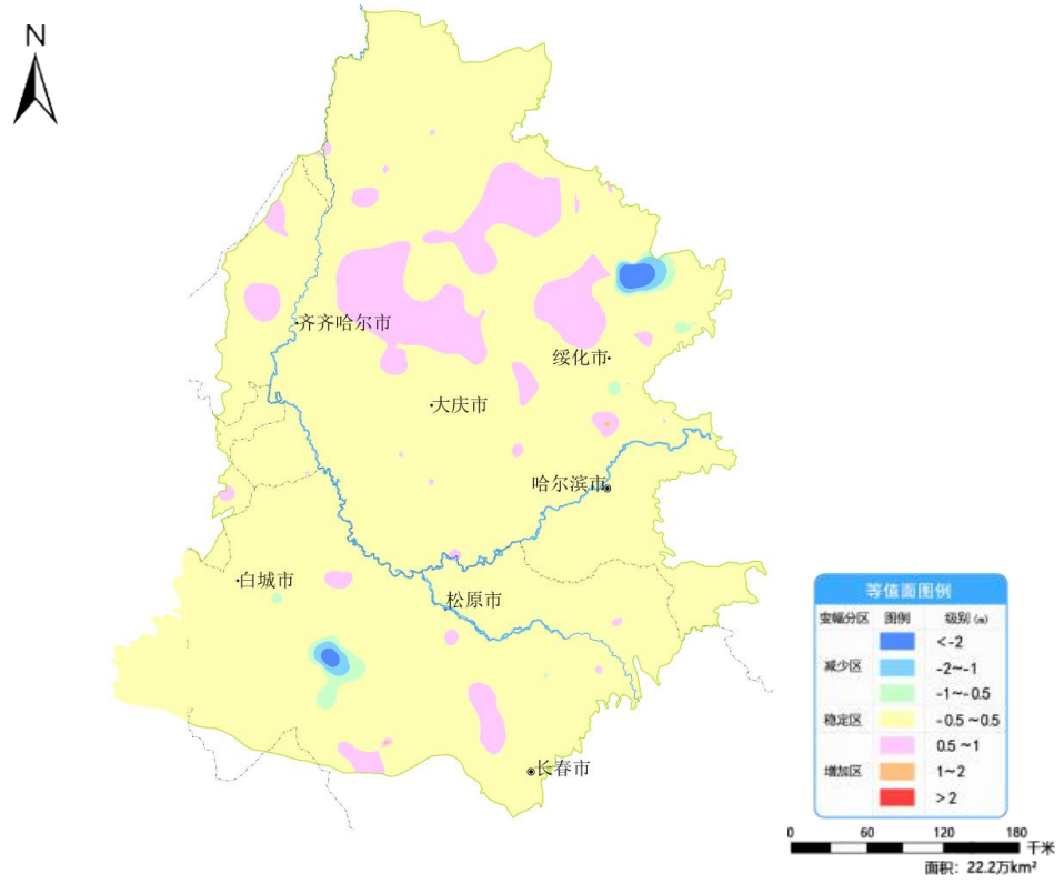
图5 松嫩平原1月份与上月地下水埋深变幅图
