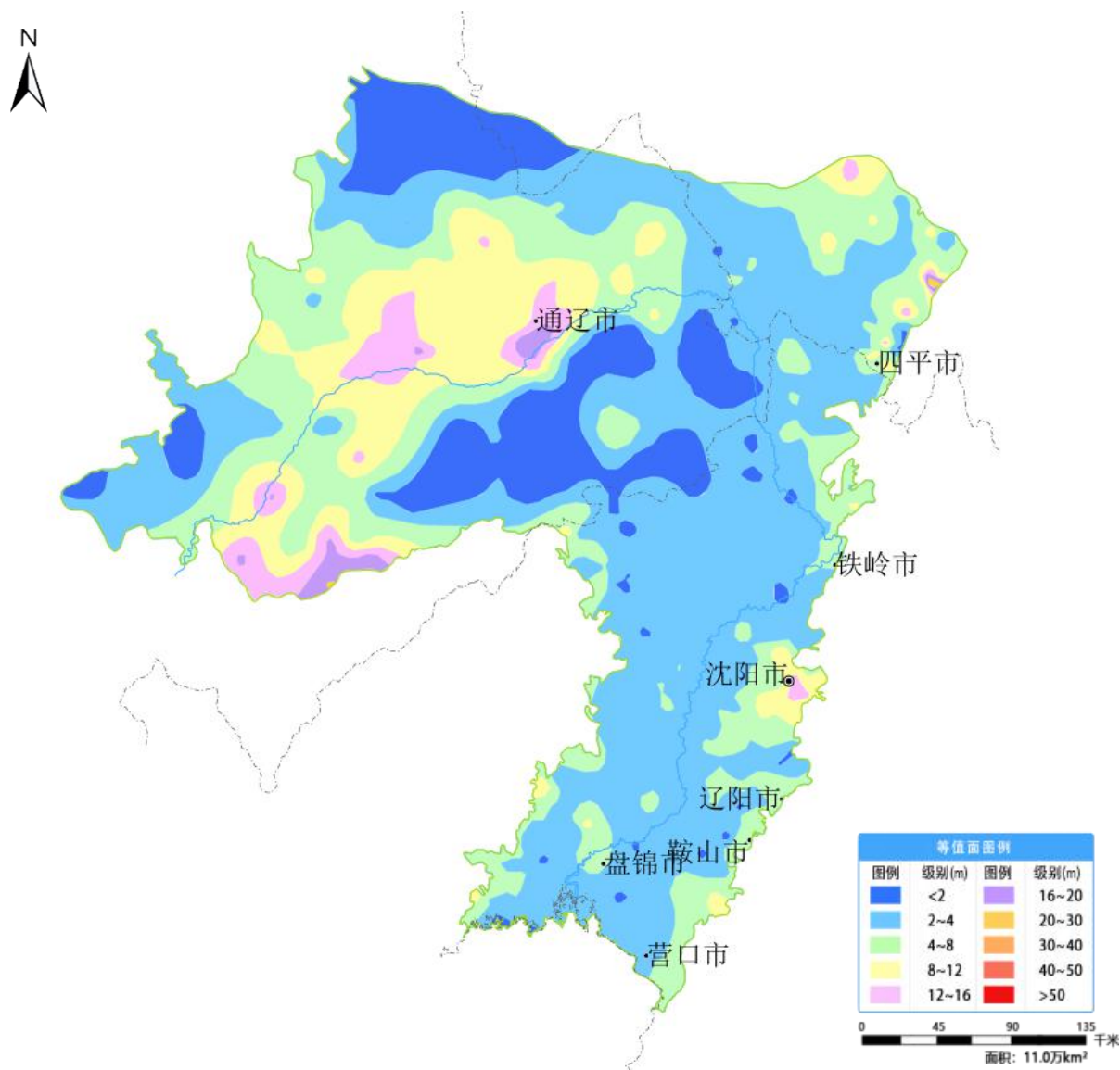
图 7 辽河平原 1 月份地下水埋深等值面图
