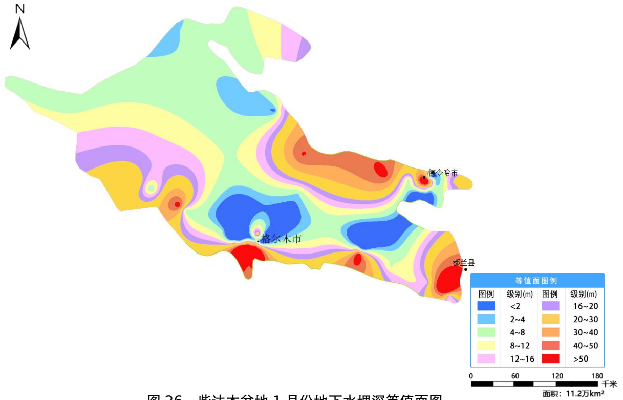
图 26 柴达木盆地 1 月份地下水埋深等值面图
