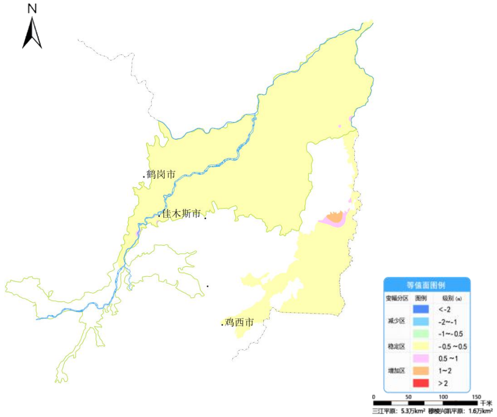
图2 三江平原及穆棱兴凯平原1月份与上月地下水埋深变幅图
