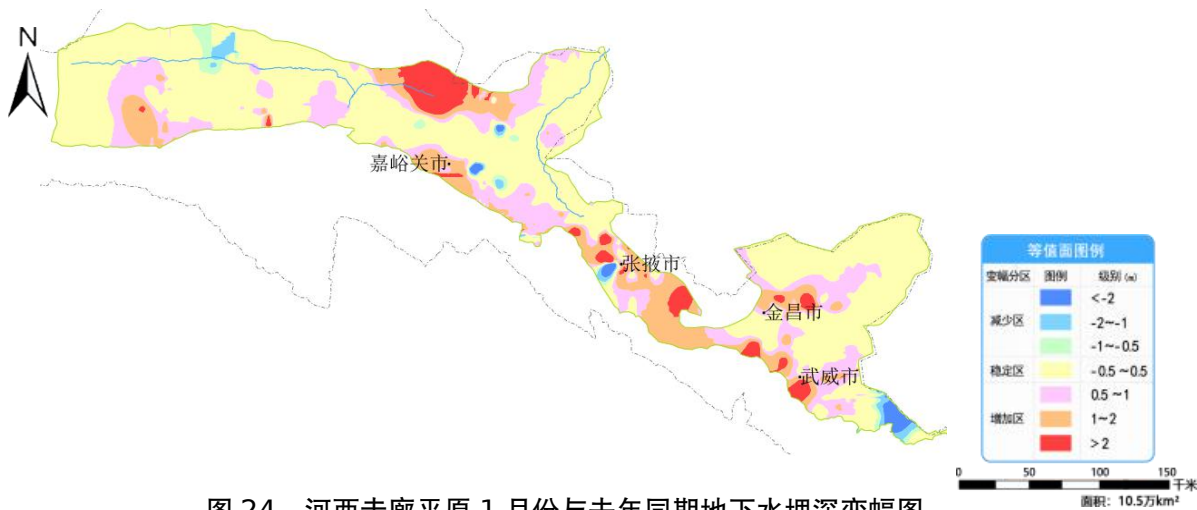
图 24 河西走廊平原 1 月份与去年同期地下水埋深变幅图
