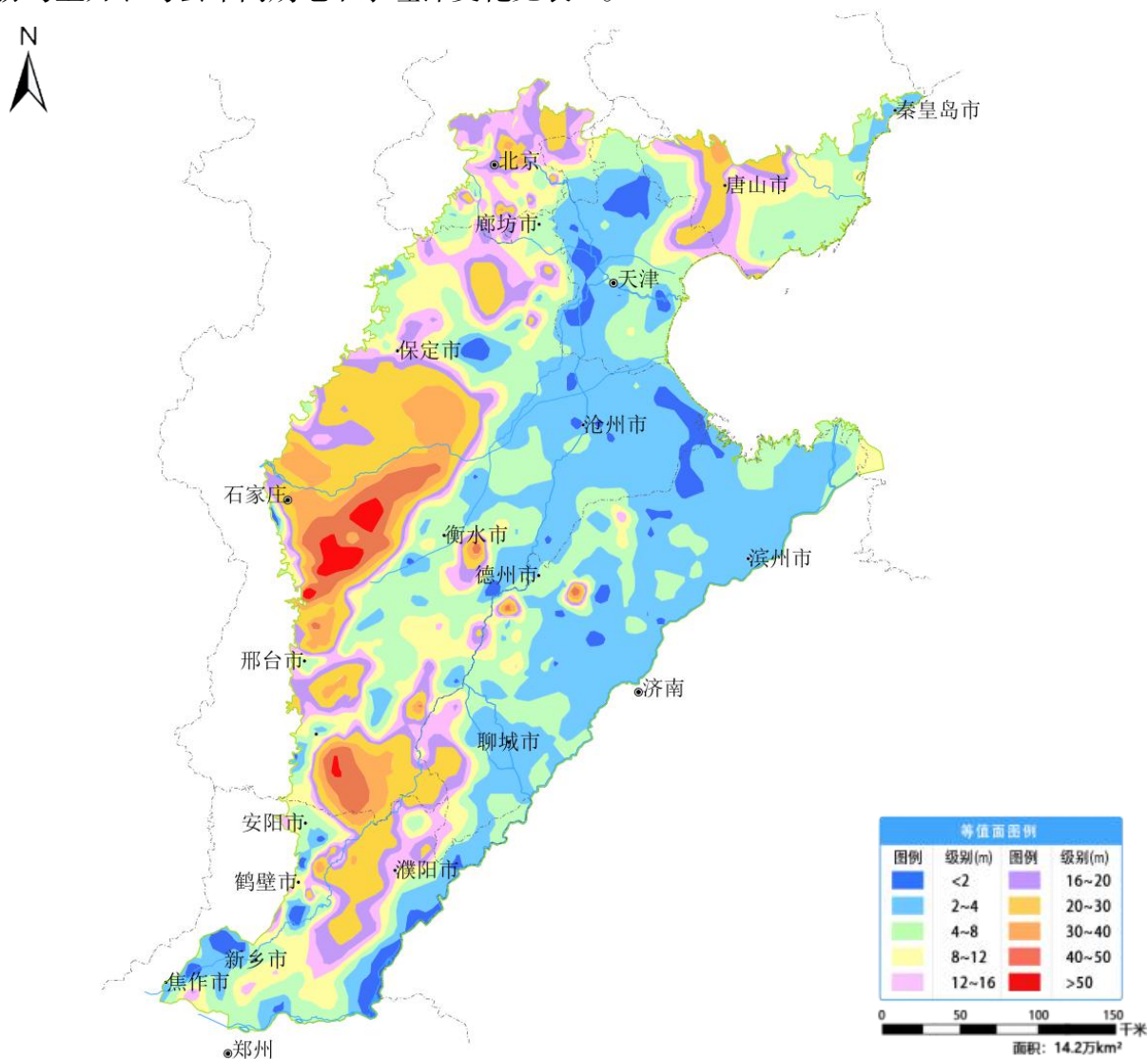
图 10 海河平原 1 月份地下水埋深等值面图
