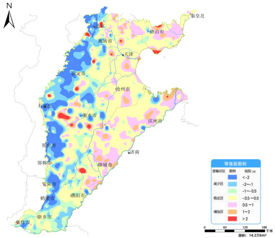
图 12 海河平原 1 月份与去年同期地下水埋深变幅图
