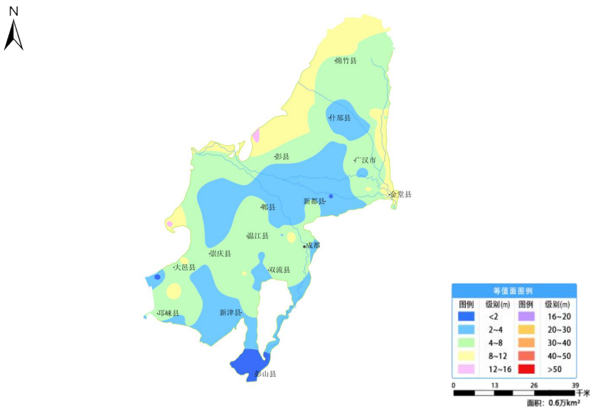
图 32 成都平原 1 月份地下水埋深等值面图
