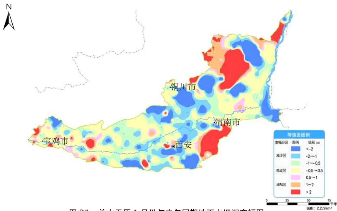
图 21 关中平原 1 月份与去年同期地下水埋深变幅图
