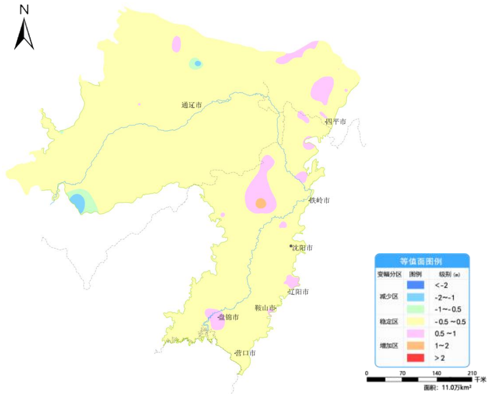
图 8 辽河平原 1 月份与上月地下水埋深变幅图
