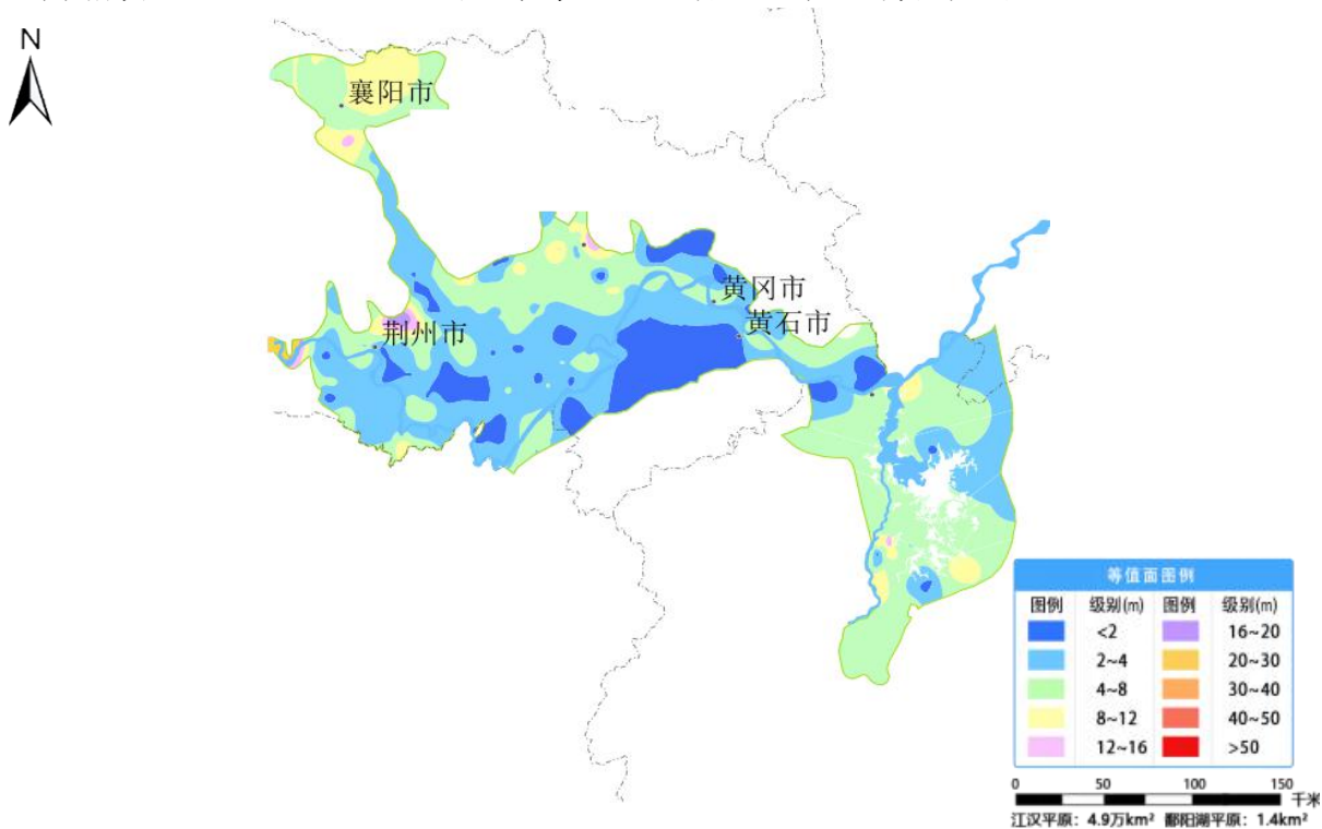
图 29 江汉及鄱阳湖平原 1 月份地下水埋深等值面图
