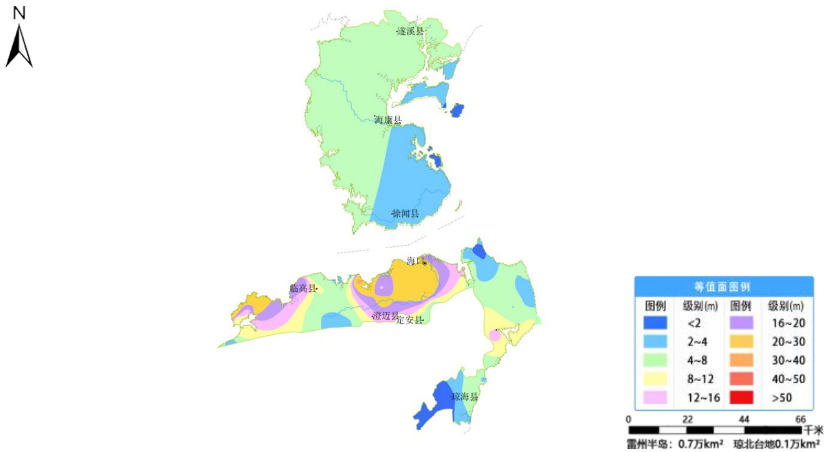
图 34 雷州半岛一般平原、琼北台地一般平原 1 月份地下水埋深等值面图
