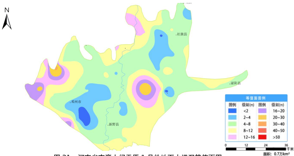
图 31 河南省南襄山间平原 1 月份地下水埋深等值面图
