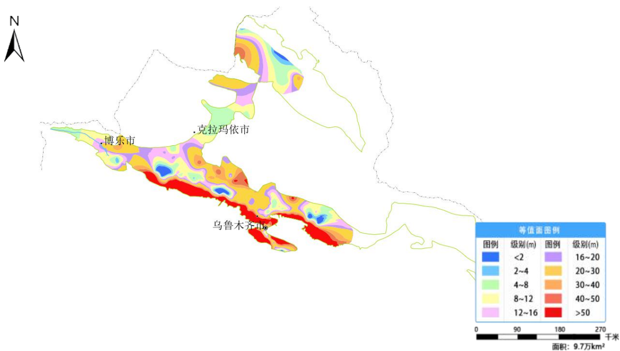
图 28 准噶尔盆地监控区 1 月份地下水埋深等值面图
