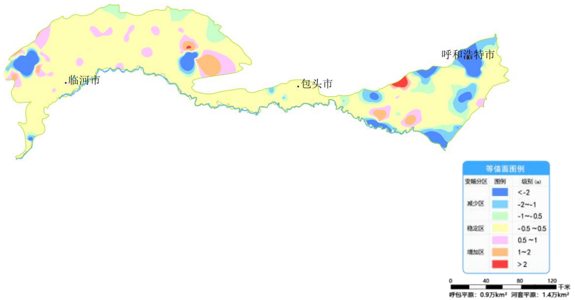
图 17 呼包平原及河套平原 1 月份与上月地下水埋深变幅图
