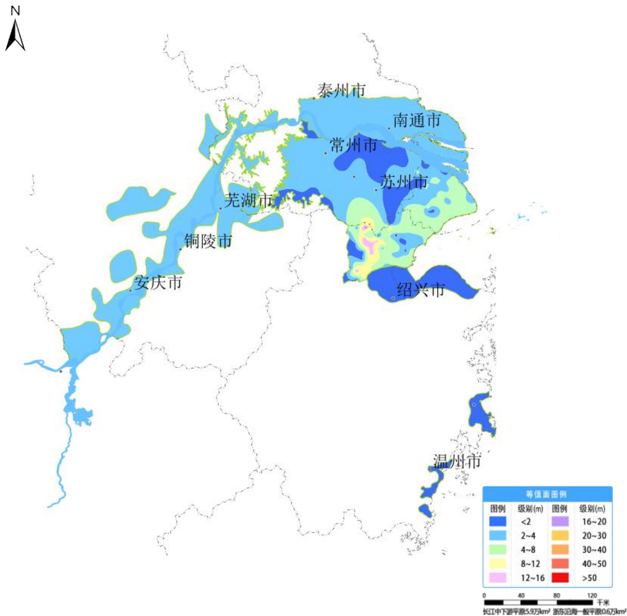
图 30 长江三角洲及浙东沿海一般平原 1 月份地下水埋深等值面图
