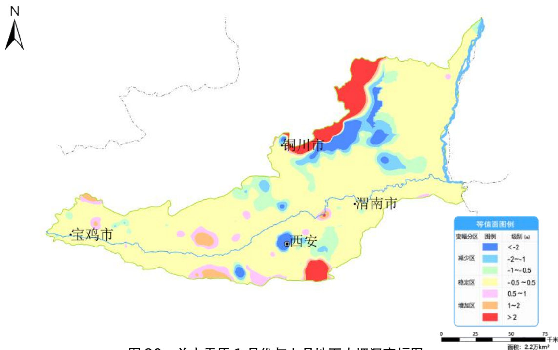
图 20 关中平原 1 月份与上月地下水埋深变幅图
