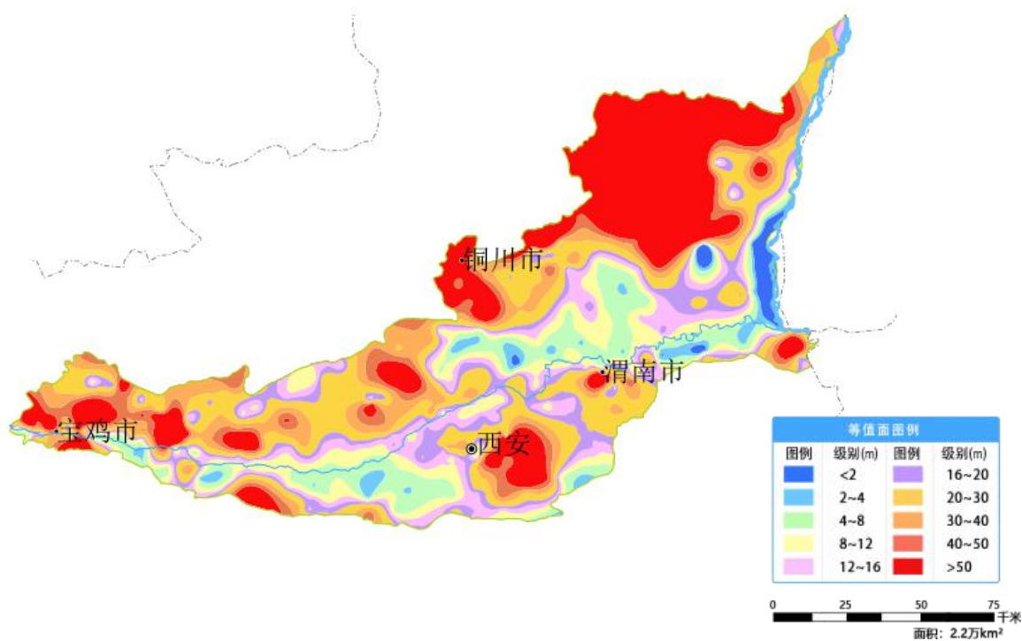
图 19 关中平原 1 月份地下水埋深等值面图
