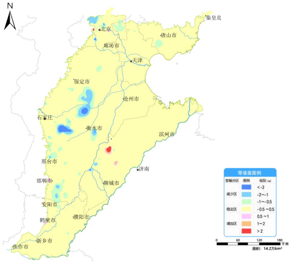
图 11 海河平原 2 月份与上月地下水埋深变幅图
