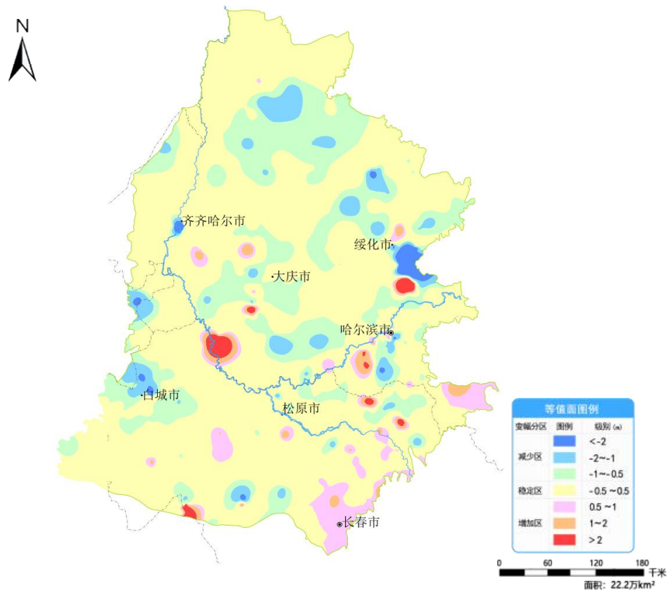
图6 松嫩平原2月份与去年同期地下水埋深变幅图
