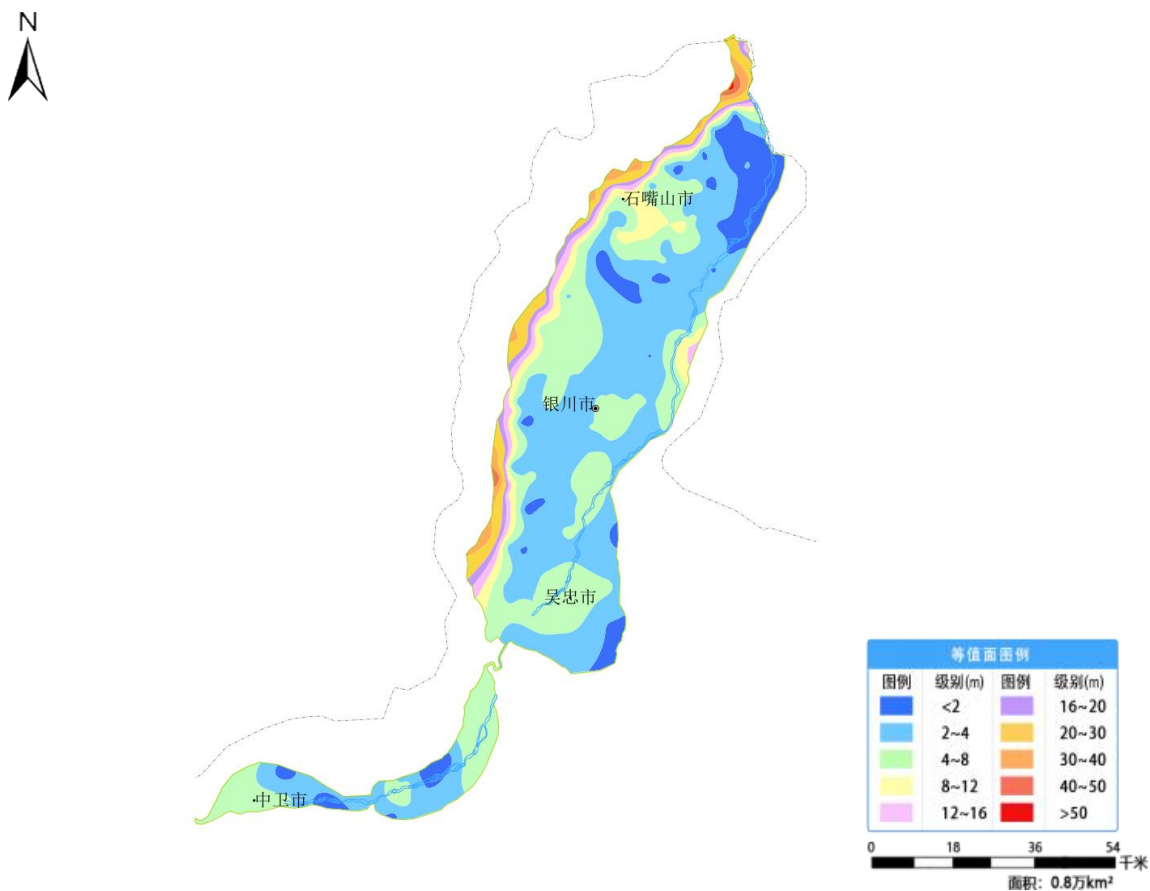
图 25 银川卫宁平原 2 月份地下水埋深等值面图
