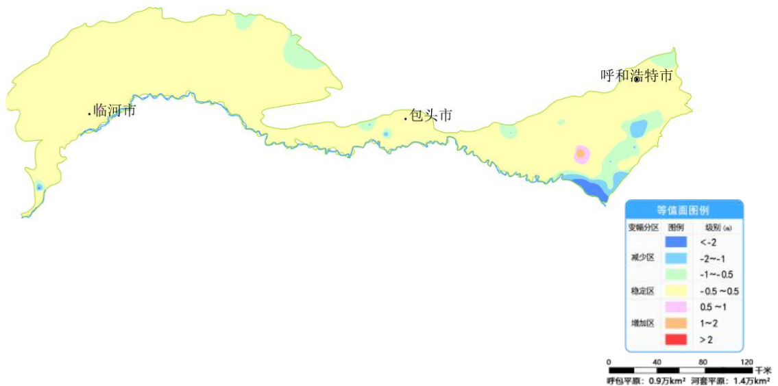
图 17 呼包平原及河套平原 2 月份与上月地下水埋深变幅图
