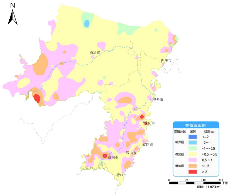
图9 辽河平原2月份与去年同期地下水埋深变幅图
