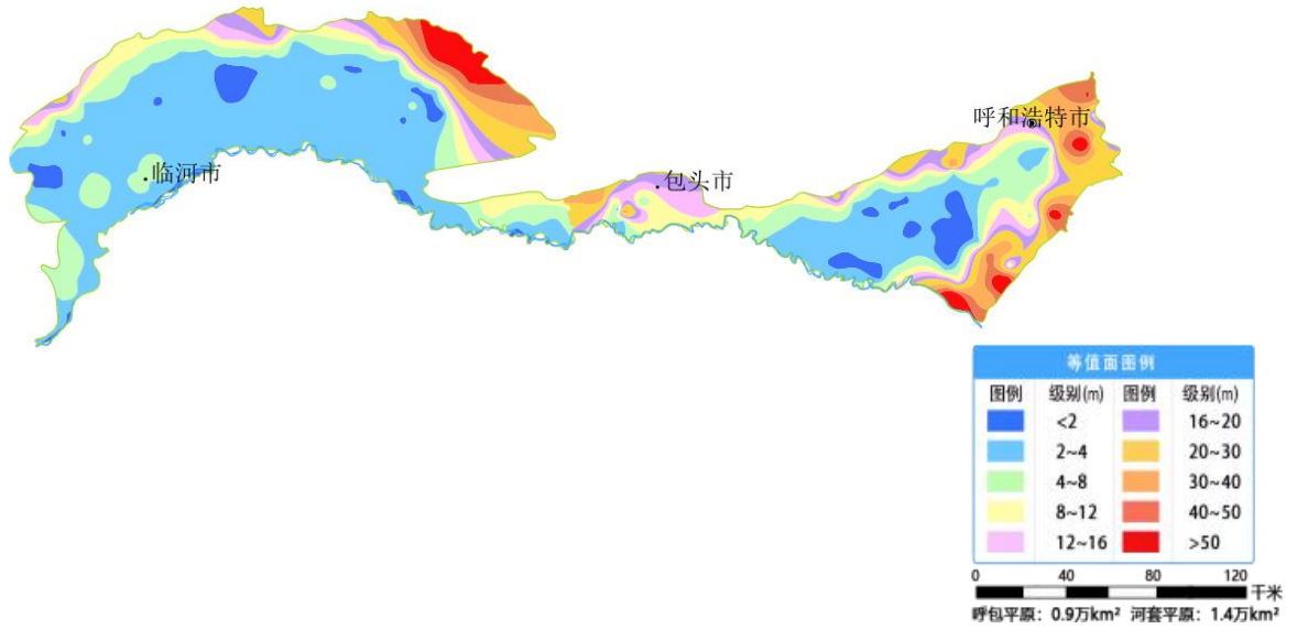
图 16 呼包平原及河套平原 2 月份地下水埋深等值面图
