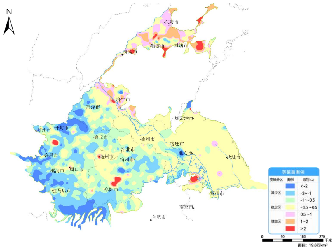
图 15 黄淮平原 2 月份与去年同期地下水埋深变幅图
