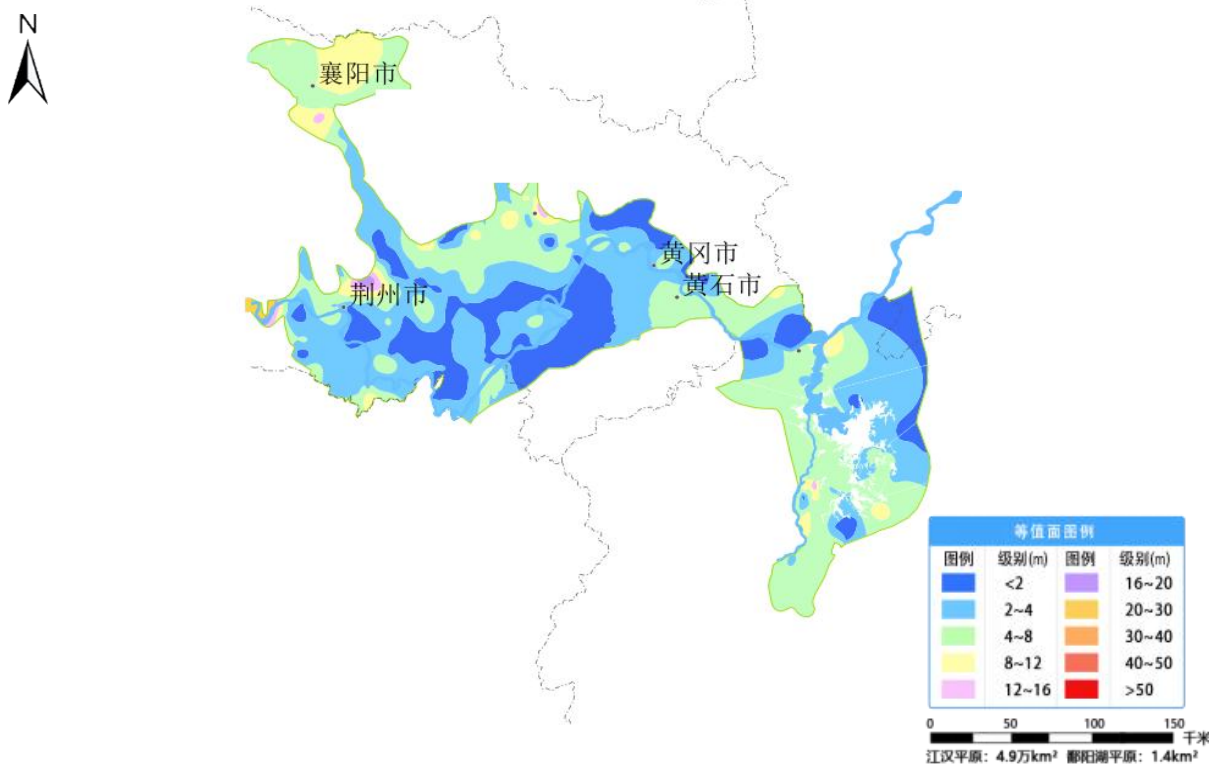
图 29 江汉及鄱阳湖平原 2 月份地下水埋深等值面图
