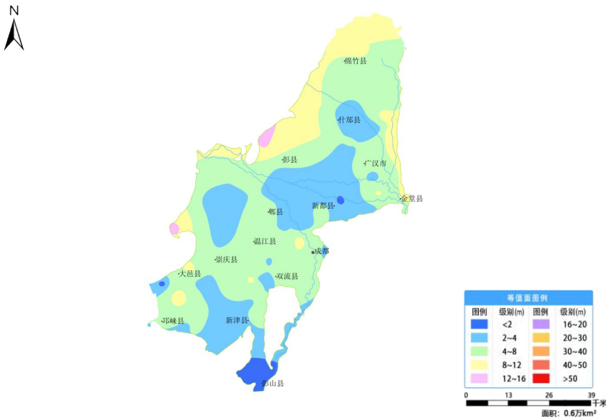
图 32 成都平原 2 月份地下水埋深等值面图
