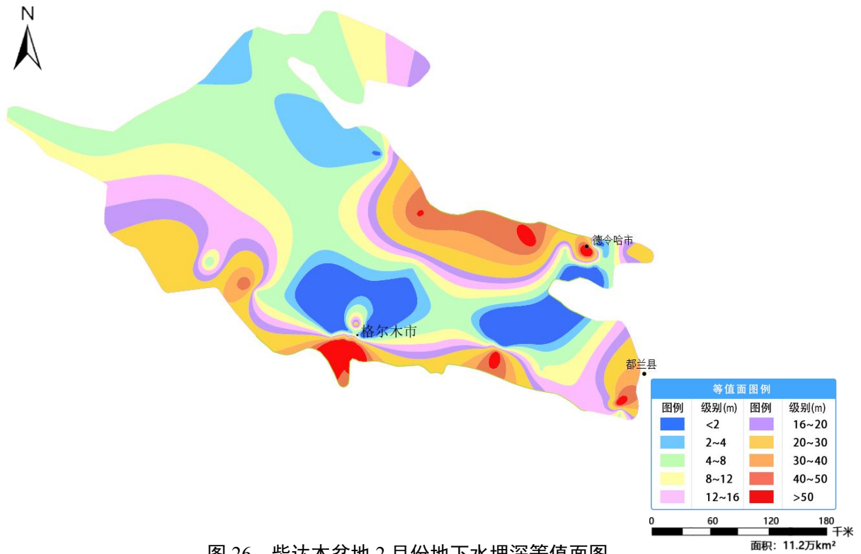
图 26 柴达木盆地 2 月份地下水埋深等值面图
