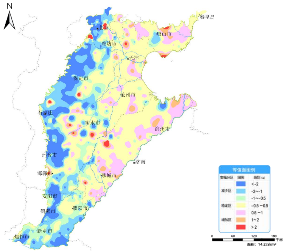
图 12 海河平原 2 月份与去年同期地下水埋深变幅图
