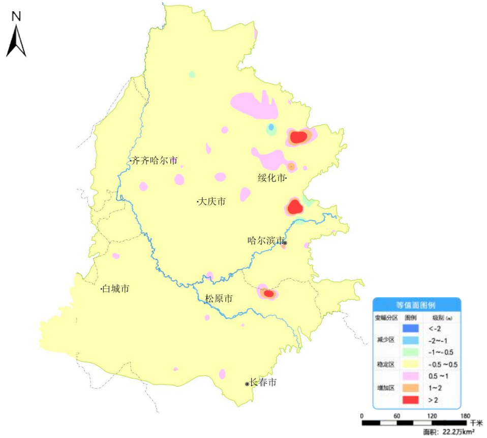
图5 松嫩平原2月份与上月地下水埋深变幅图
