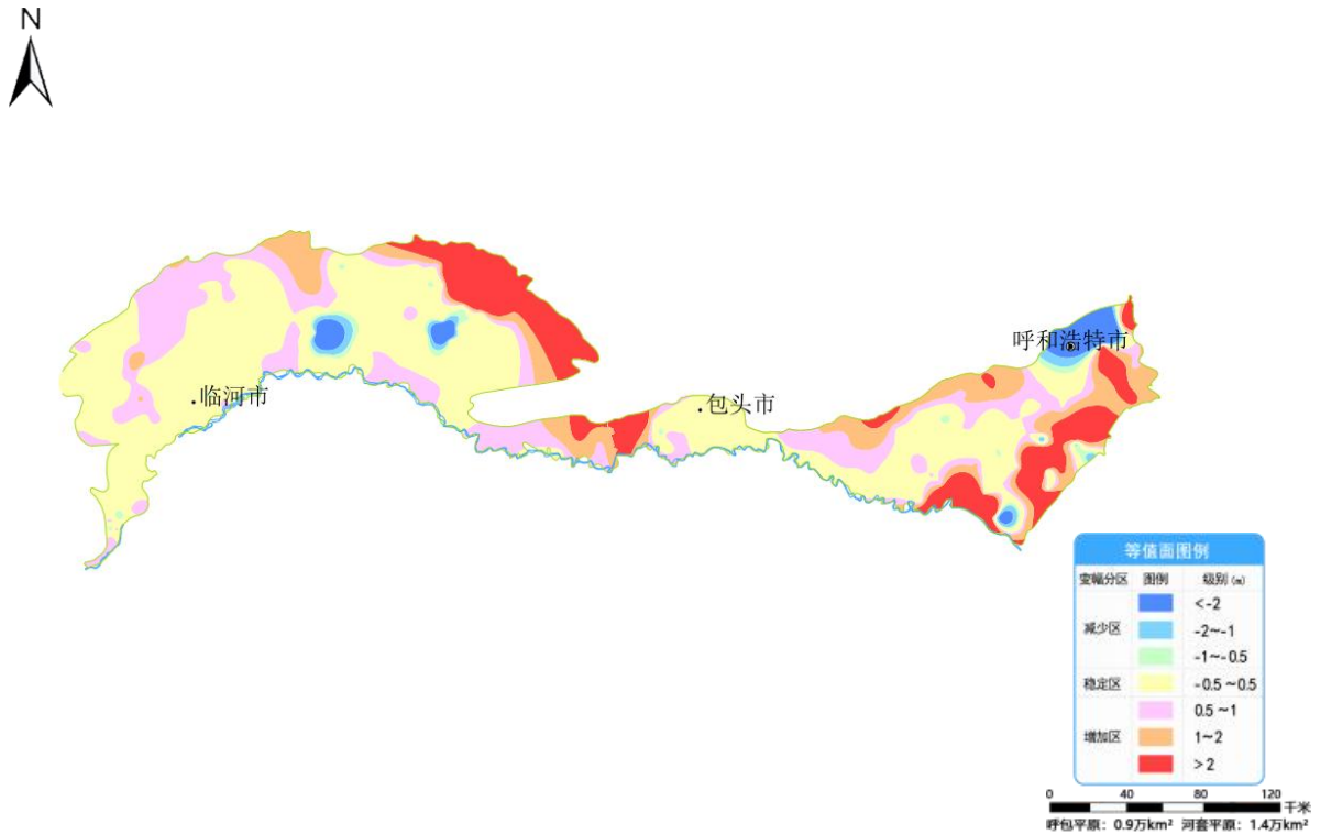
图 18 呼包平原及河套平原 2 月份与去年同期地下水埋深变幅图
