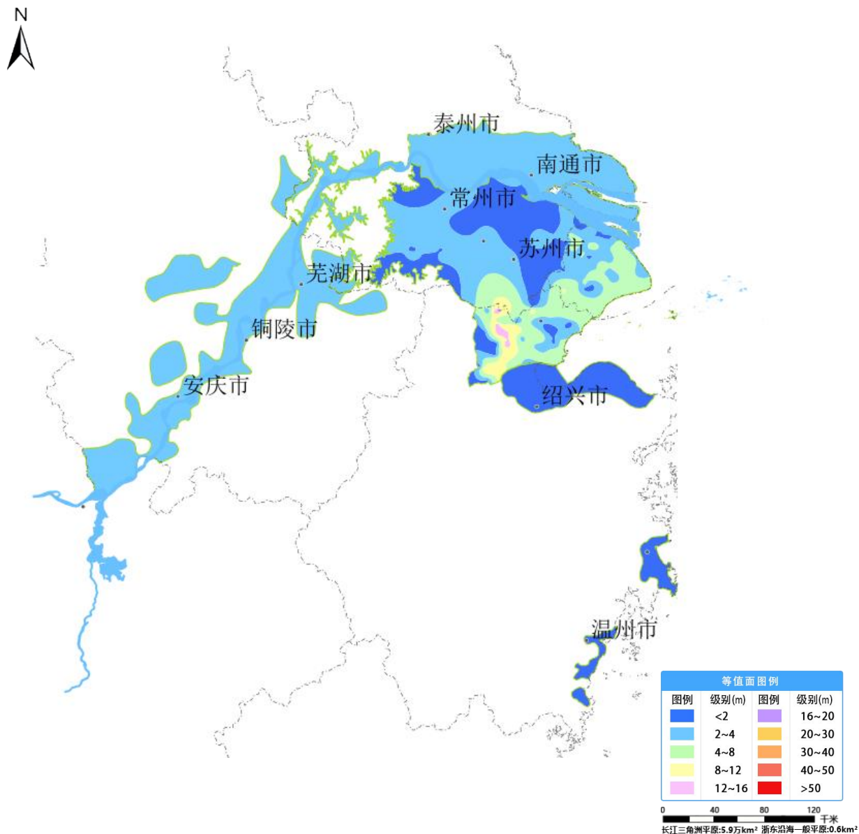
图 30 长江三角洲及浙东沿海一般平原 2 月份地下水埋深等值面图
