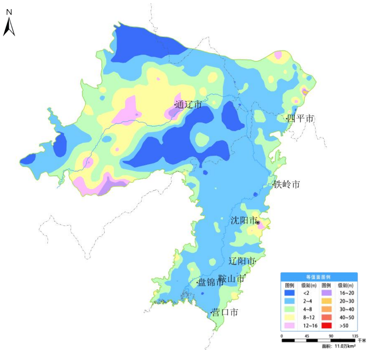
图 7 辽河平原 2 月份地下水埋深等值面图
