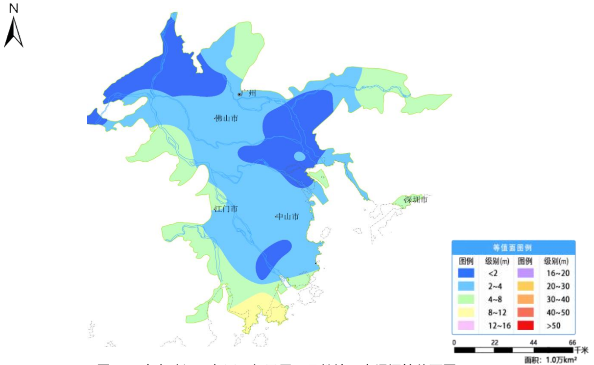
图 33 广东珠江三角洲一般平原 2 月份地下水埋深等值面图
