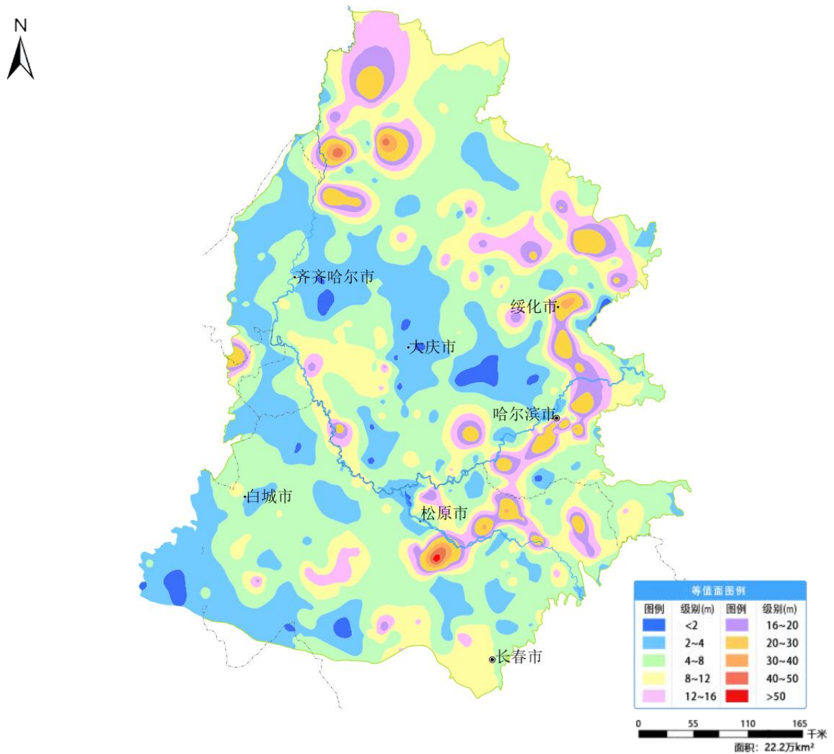
图 4 松嫩平原 2 月份地下水埋深等值面图
