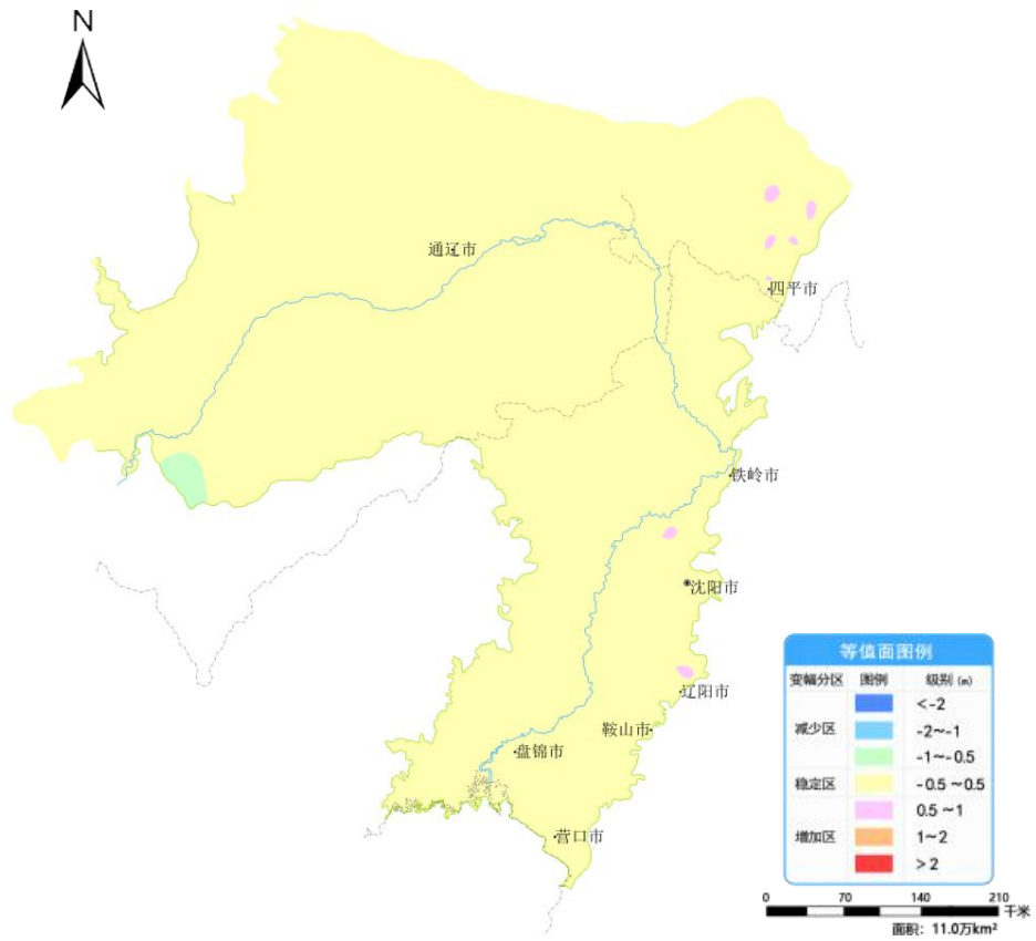
图8 辽河平原2月份与上月地下水埋深变幅图
