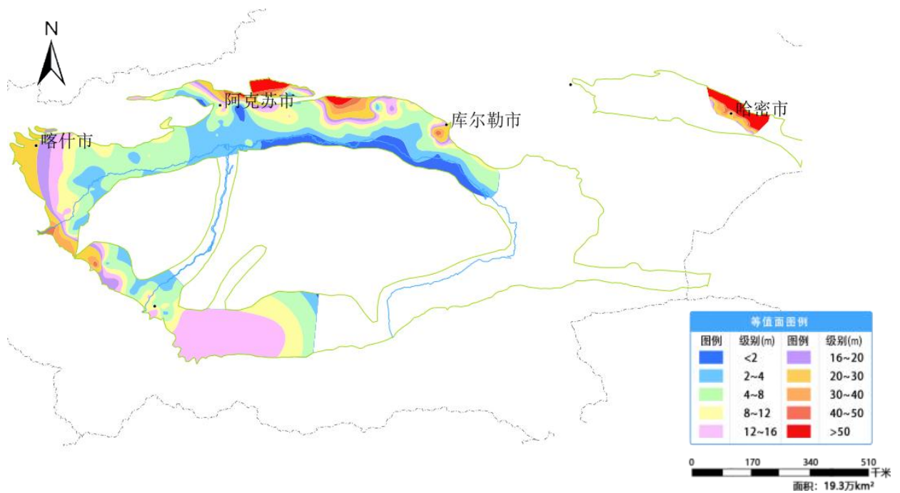
图 27 塔里木盆地监控区 2 月份地下水埋深等值面图
