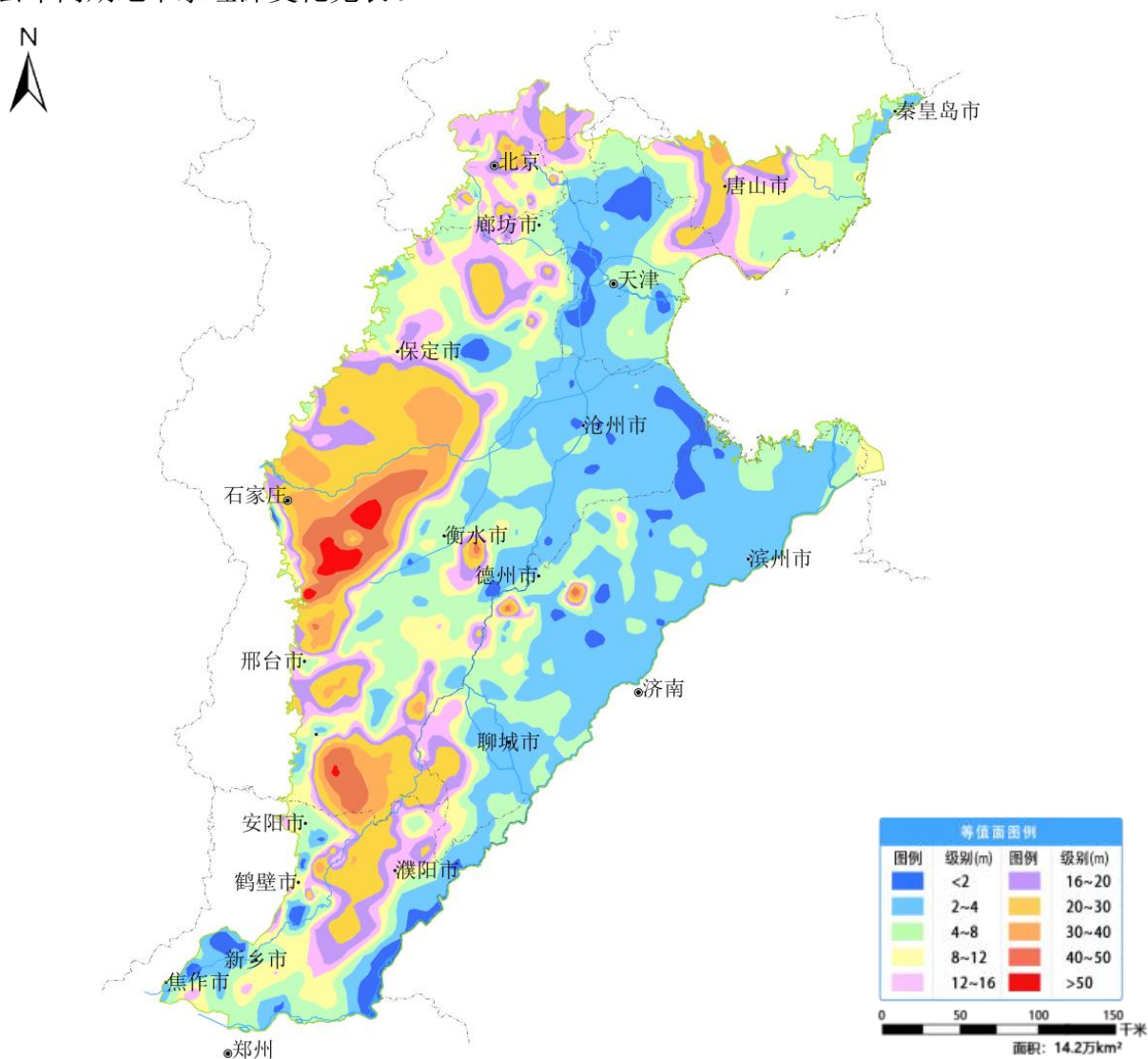
图 10 海河平原 2 月份地下水埋深等值面图
