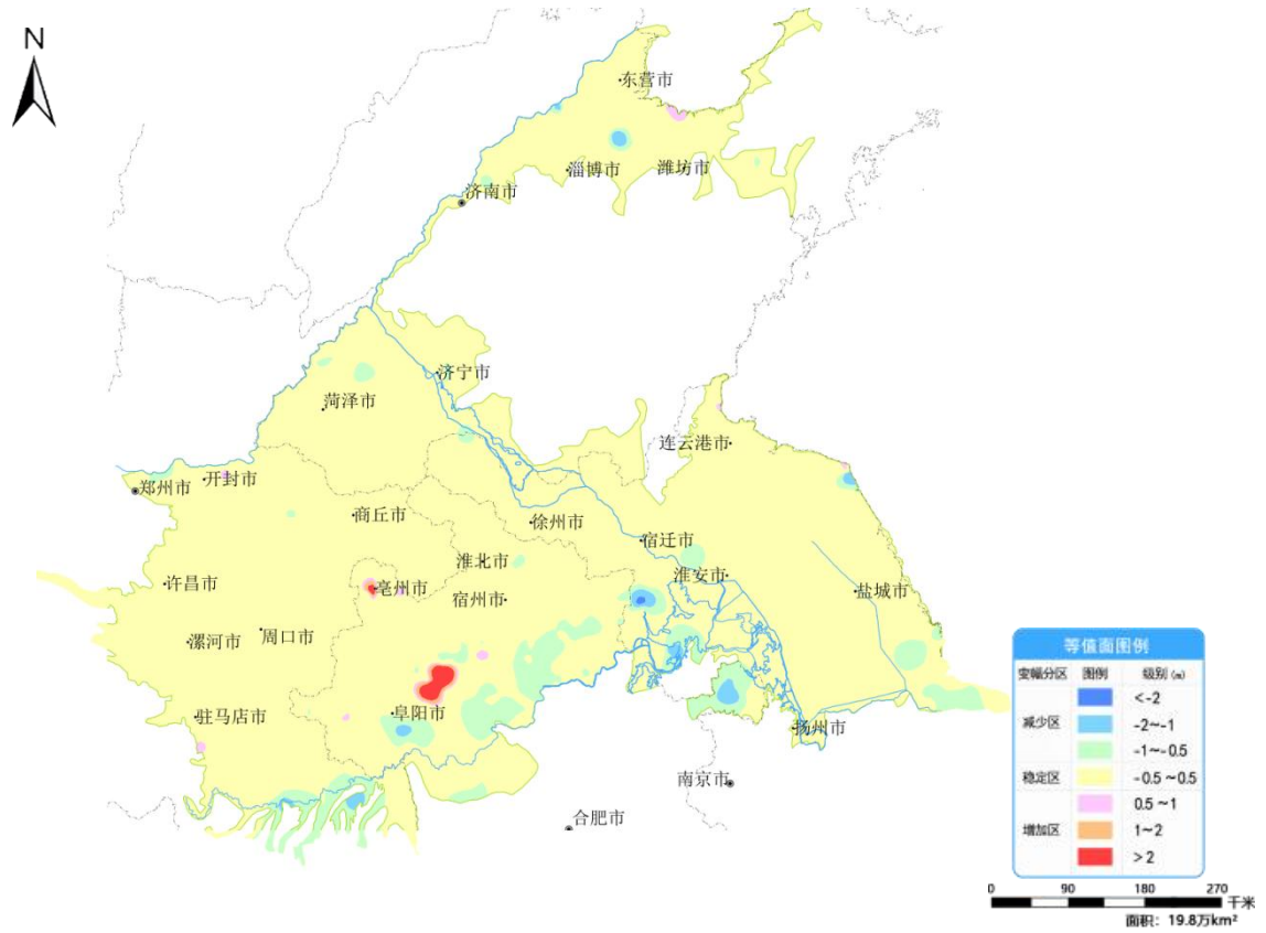
图 14 黄淮平原 2 月份与上月地下水埋深变幅图
