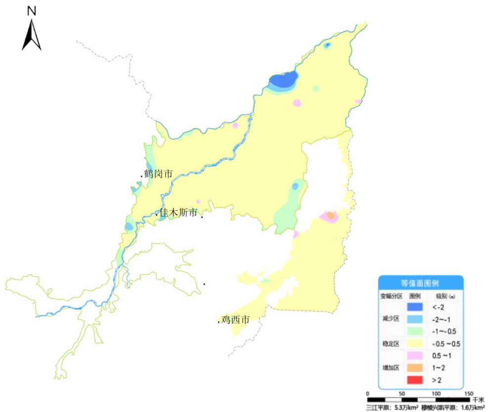
图3 三江平原及穆棱兴凯平原2月份与去年同期地下水埋深变幅图
