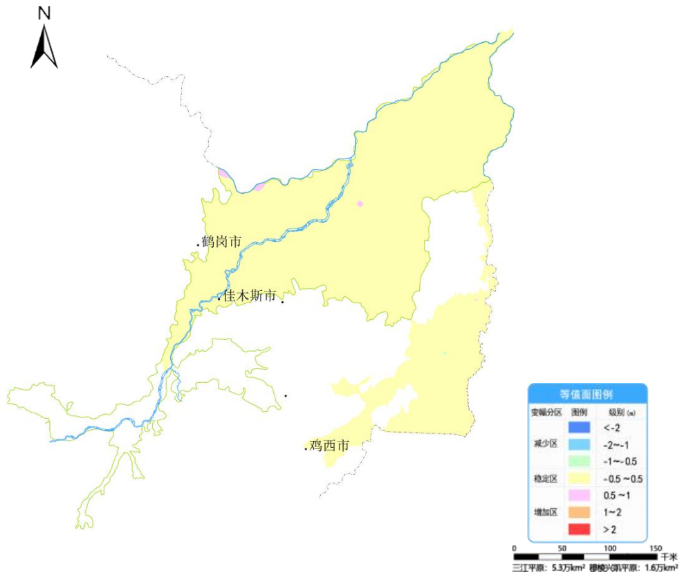
图2 三江平原及穆棱兴凯平原2月份与上月地下水埋深变幅图
