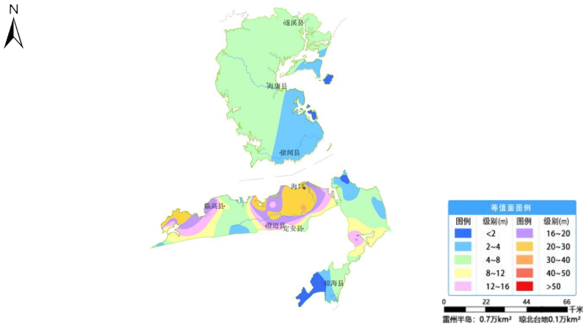
图 34 雷州半岛一般平原、琼北台地一般平原 2 月份地下水埋深等值面图
