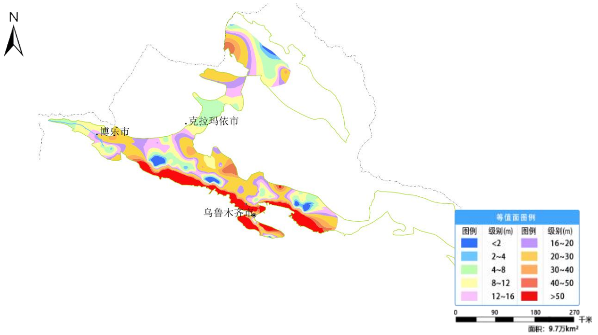
图 28 准噶尔盆地监控区 2 月份地下水埋深等值面图
