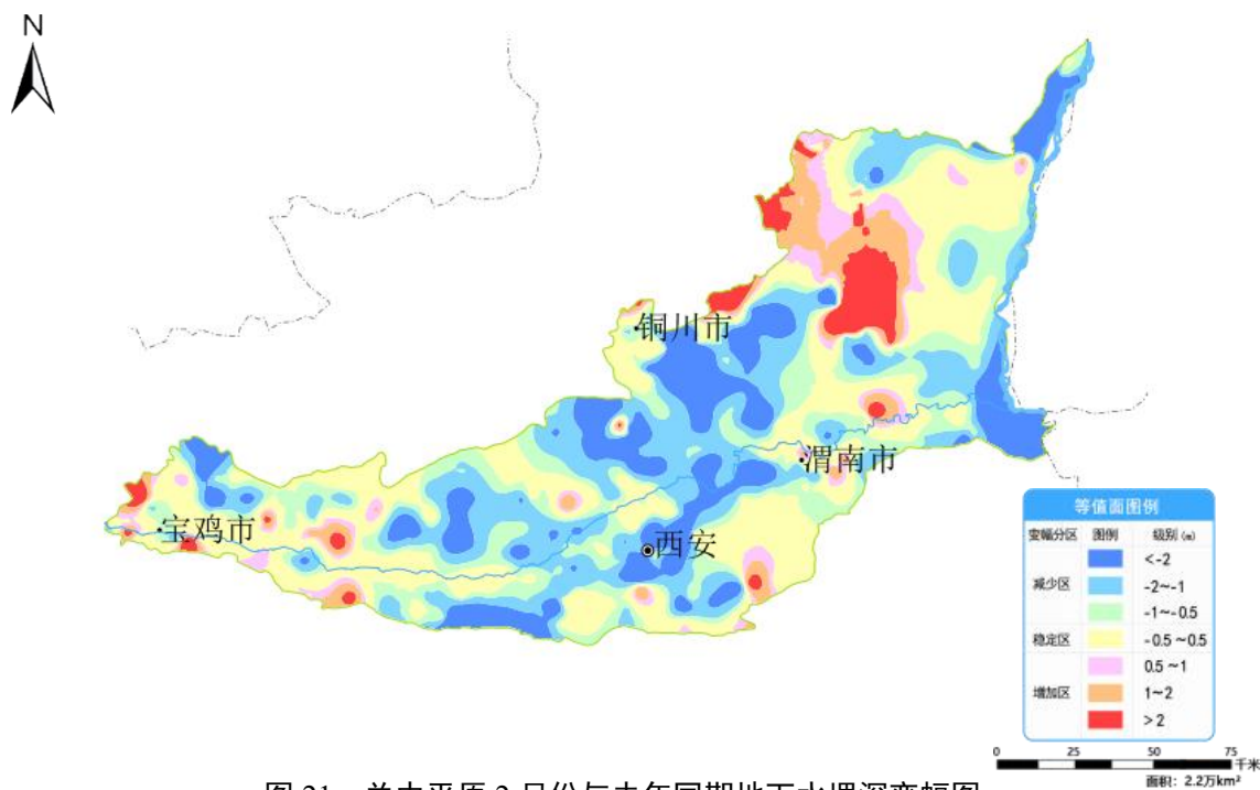
图 21 关中平原 2 月份与去年同期地下水埋深变幅图
