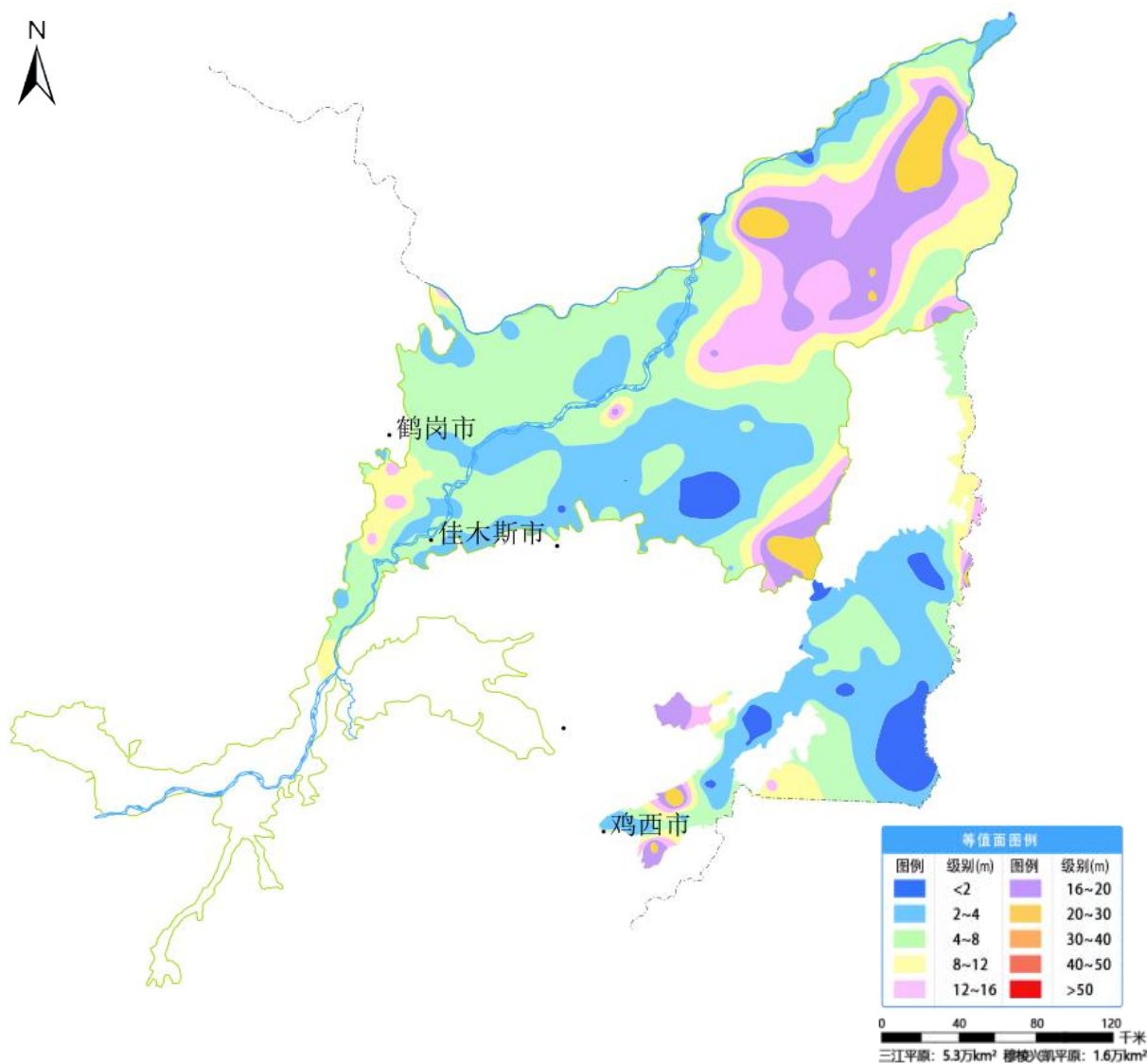
图 1 三江平原及穆棱兴凯平原 2 月份地下水埋深等值面图
