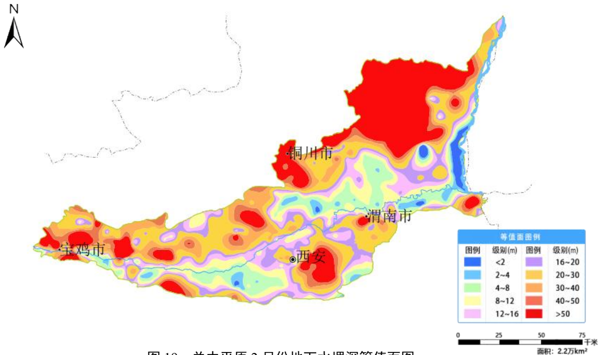
图 19 关中平原 2 月份地下水埋深等值面图
