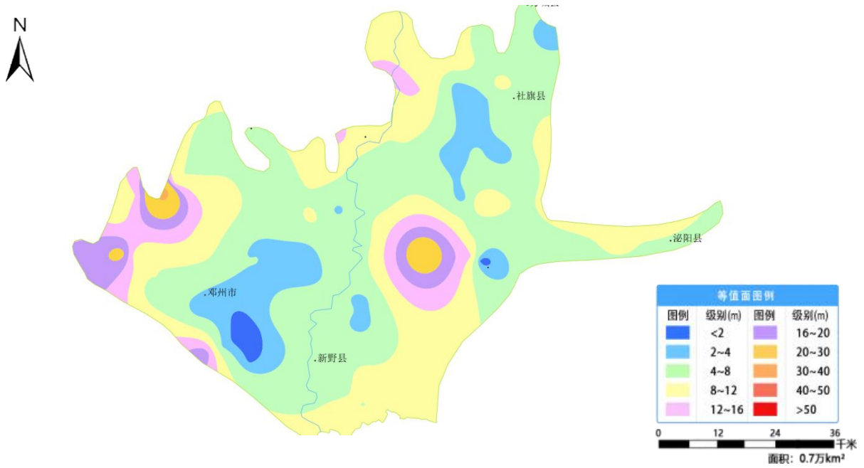
图 31 河南省南襄山间平原 2 月份地下水埋深等值面图
