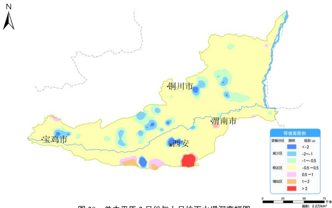
图 20 关中平原 2 月份与上月地下水埋深变幅图
