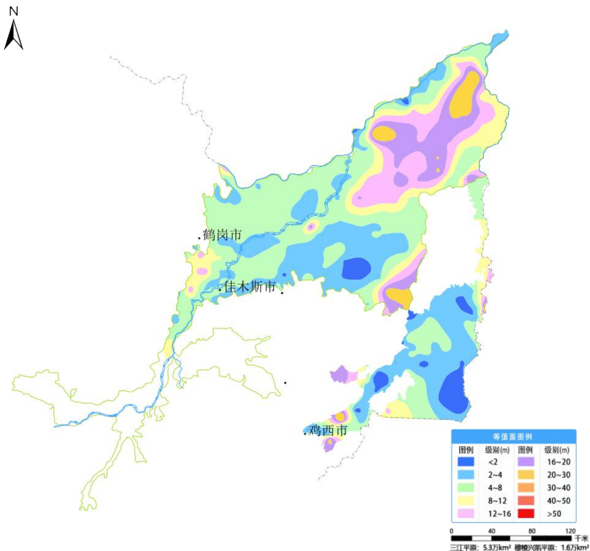
图1 三江平原和穆棱兴凯平原3月份地下水埋深等值面图
