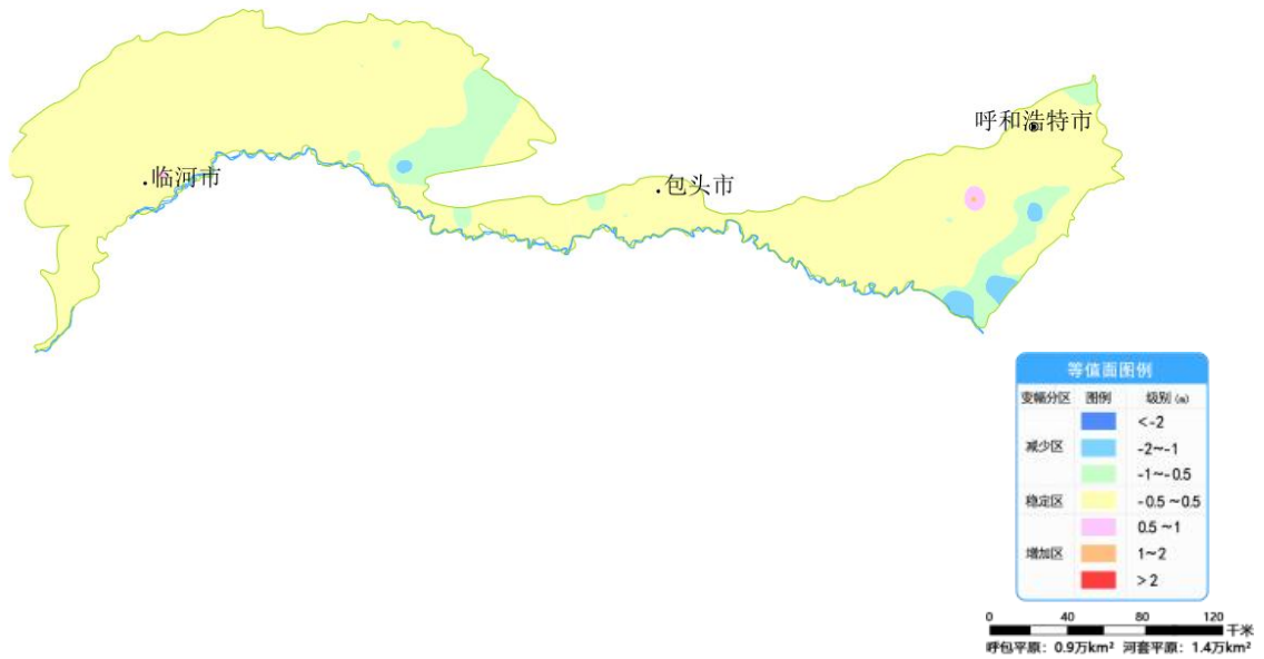
图 17 呼包平原和河套平原 3 月份与上月相比地下水埋深变幅图
