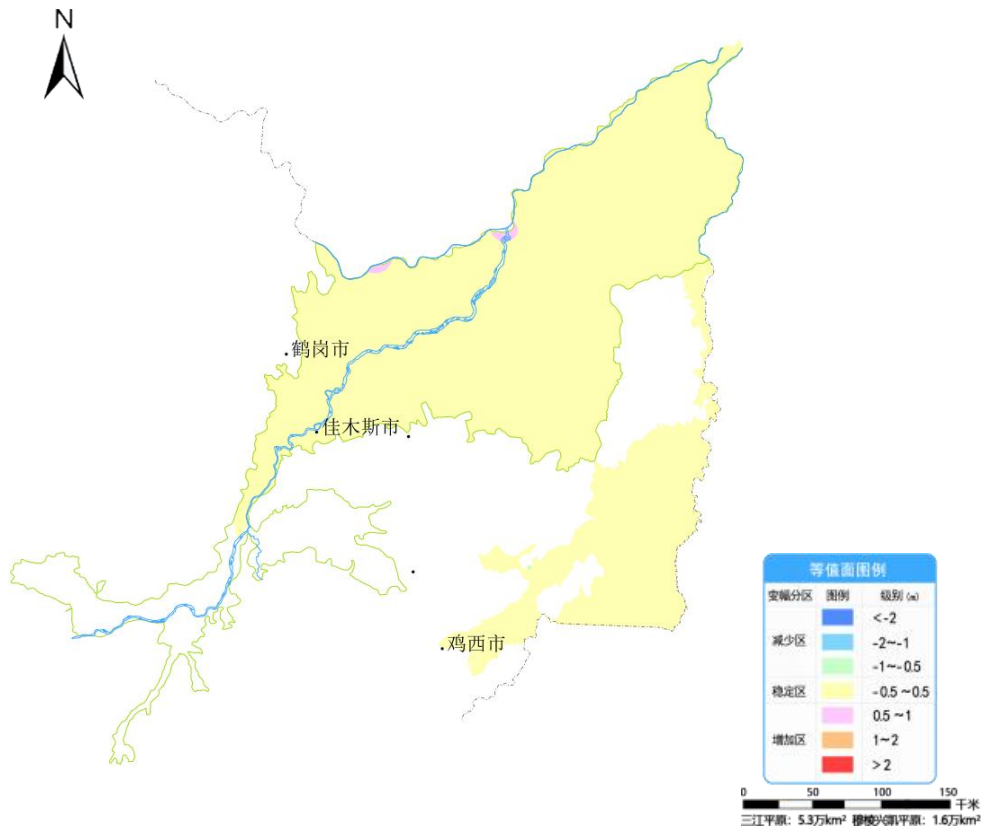
图2 三江平原和穆棱兴凯平原3月份与上月相比地下水埋深变幅图
