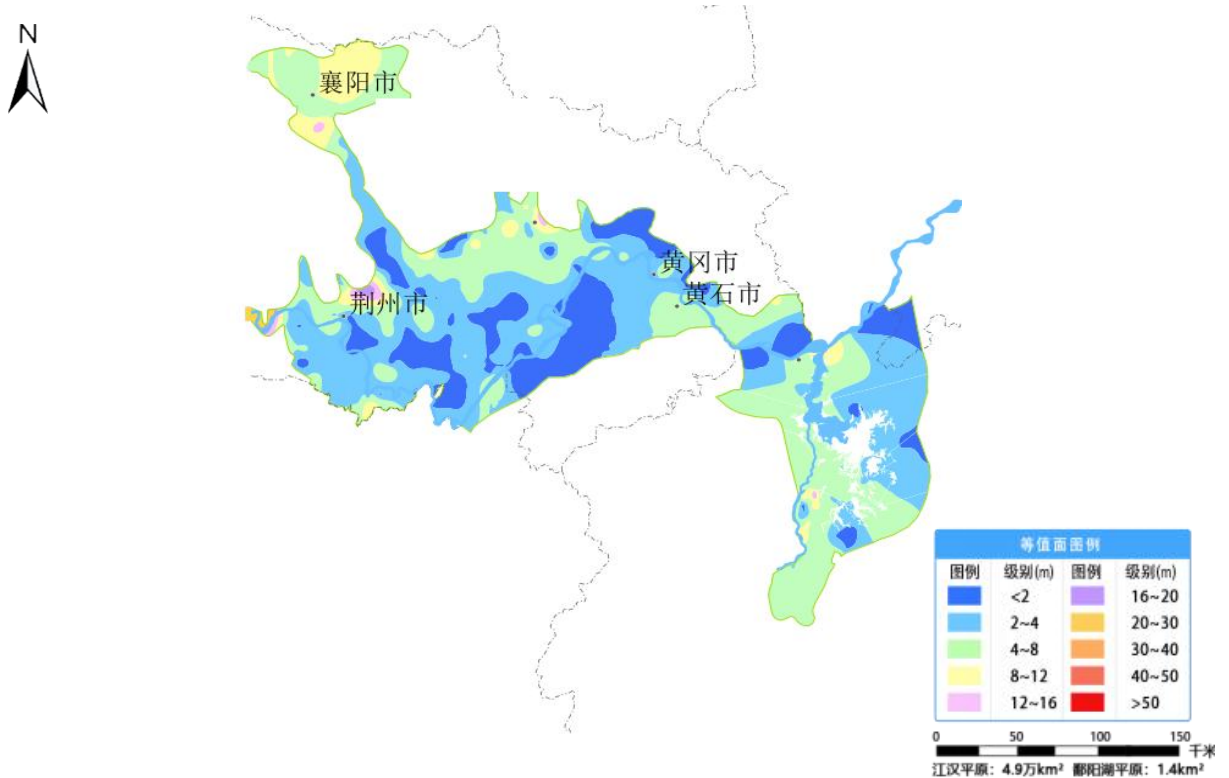
图 29 江汉平原和鄱阳湖平原 3 月份地下水埋深等值面图
