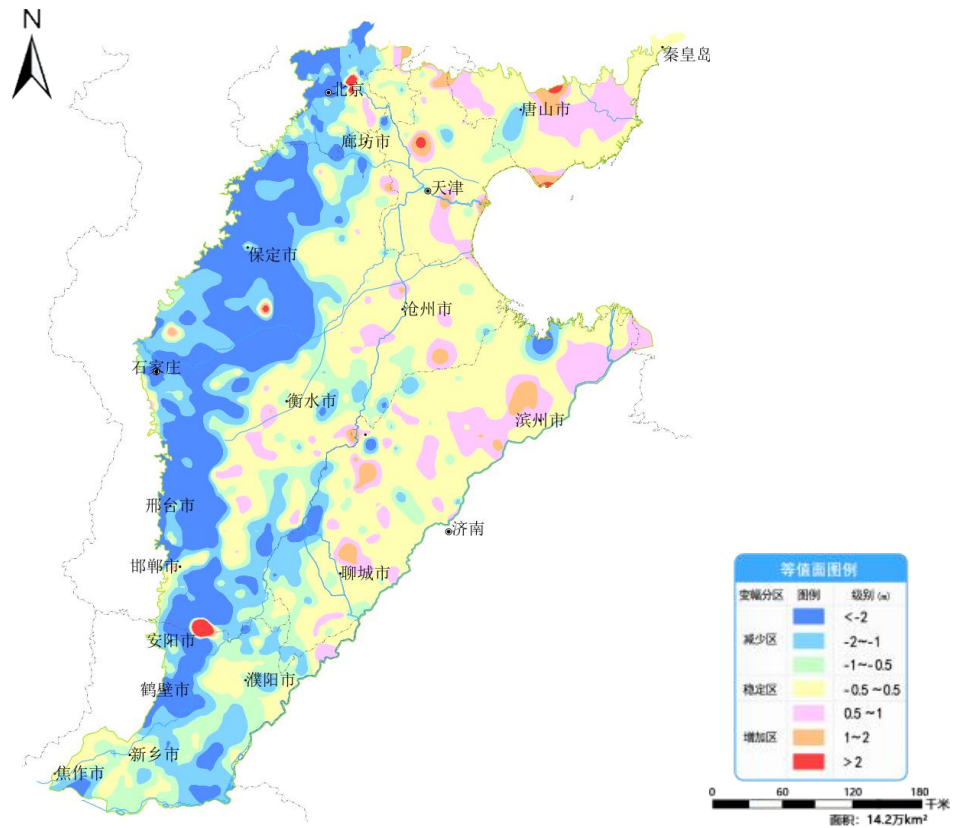
图 12 海河平原 3 月份与去年同期相比地下水埋深变幅图
