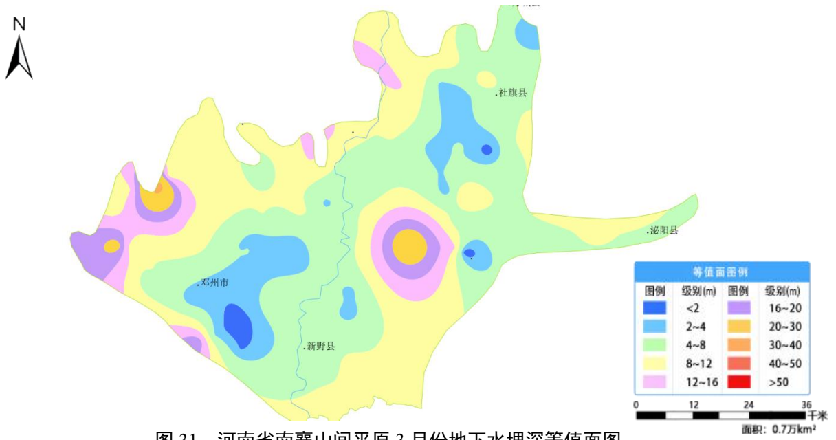
图 31 河南省南襄山间平原 3 月份地下水埋深等值面图
