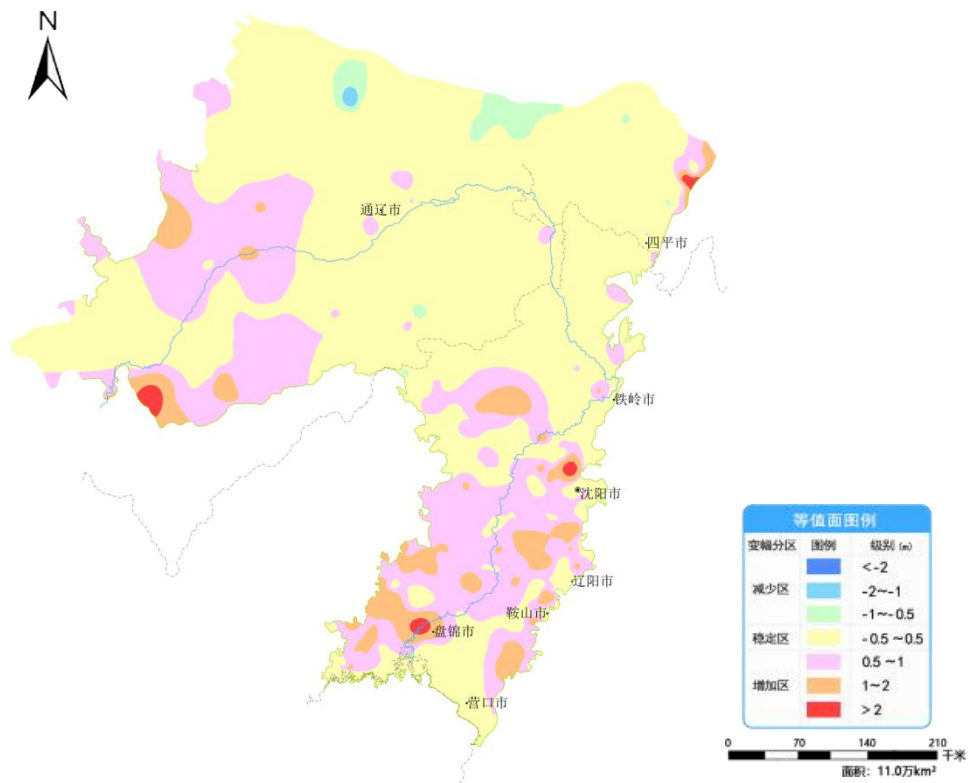
图 9 辽河平原 3 月份与去年同期相比地下水埋深变幅图
