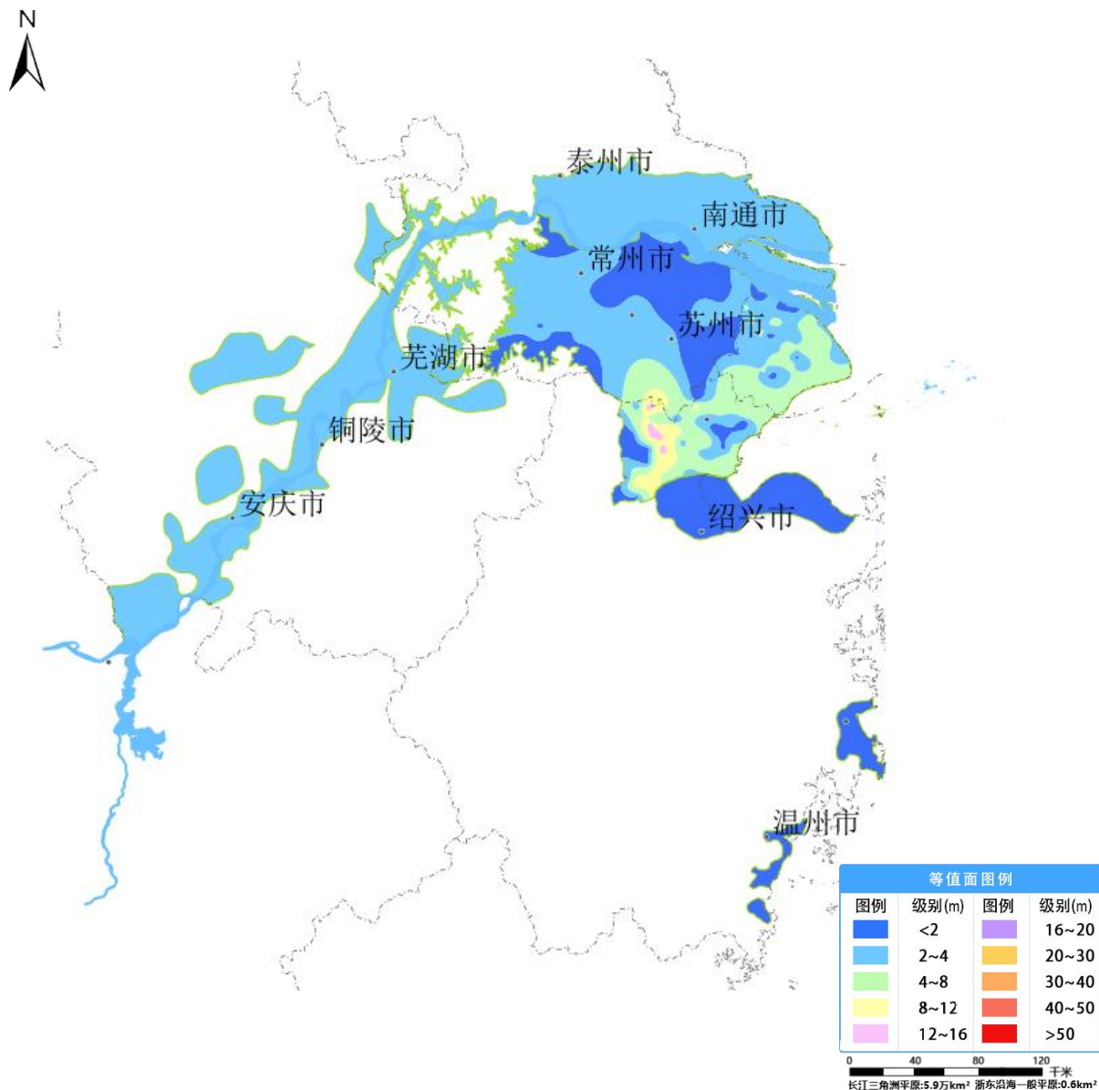
图30 长江三角洲平原和浙东沿海一般平原3月份地下水埋深等值面图
