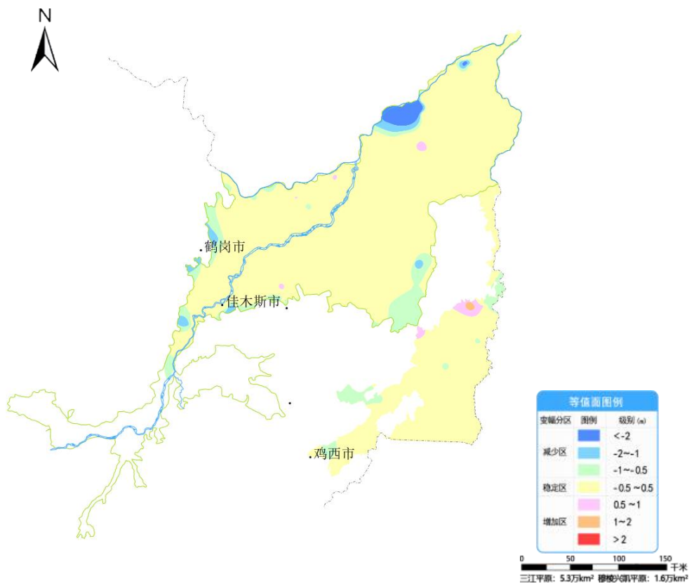
图3 三江平原和穆棱兴凯平原3月份与去年同期相比地下水埋深变幅图
