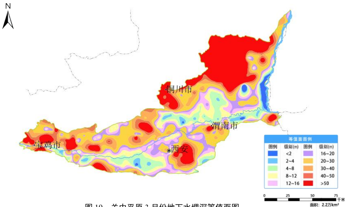
图 19 关中平原 3 月份地下水埋深等值面图
