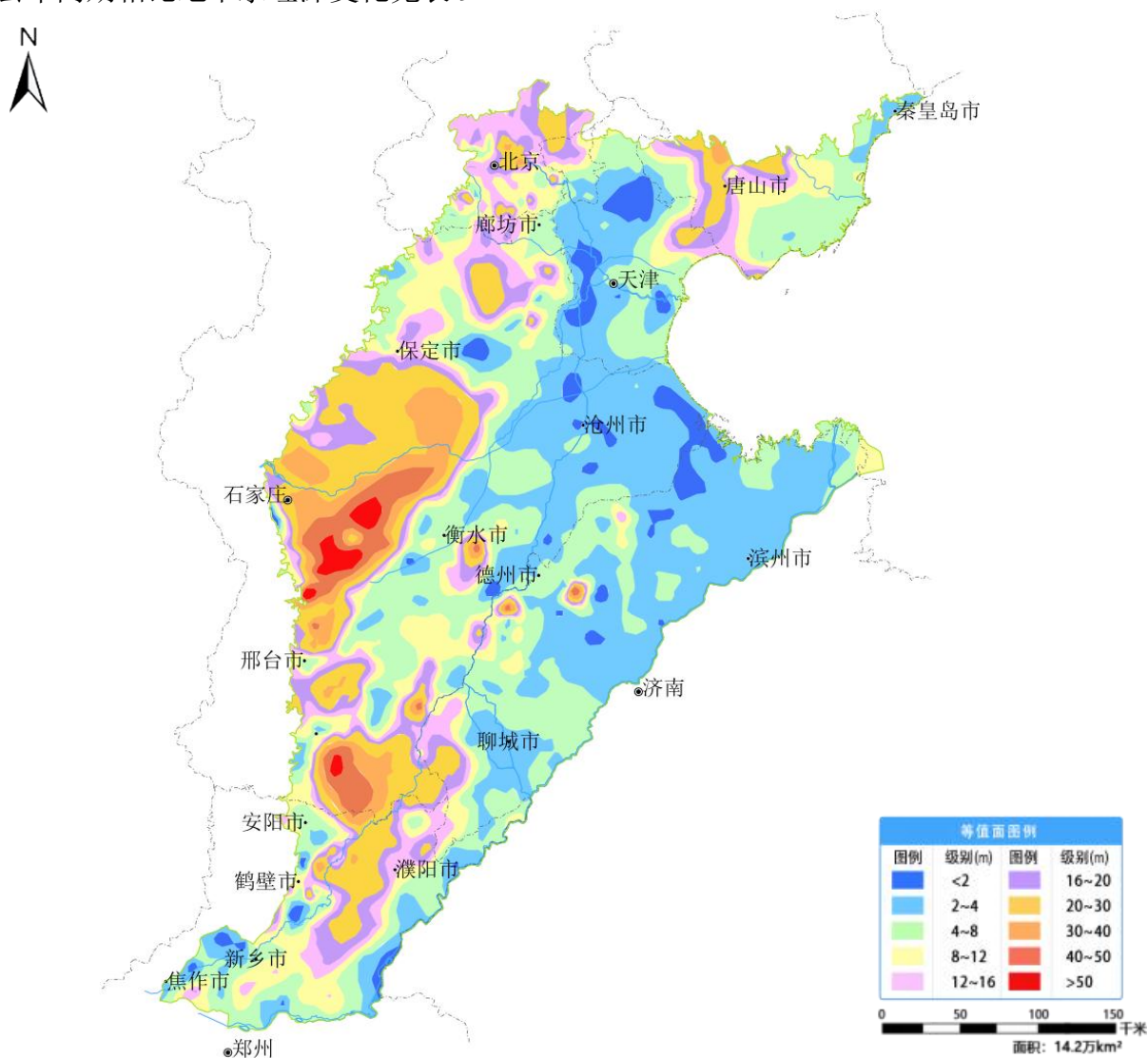
图 10 海河平原 3 月份地下水埋深等值面图
