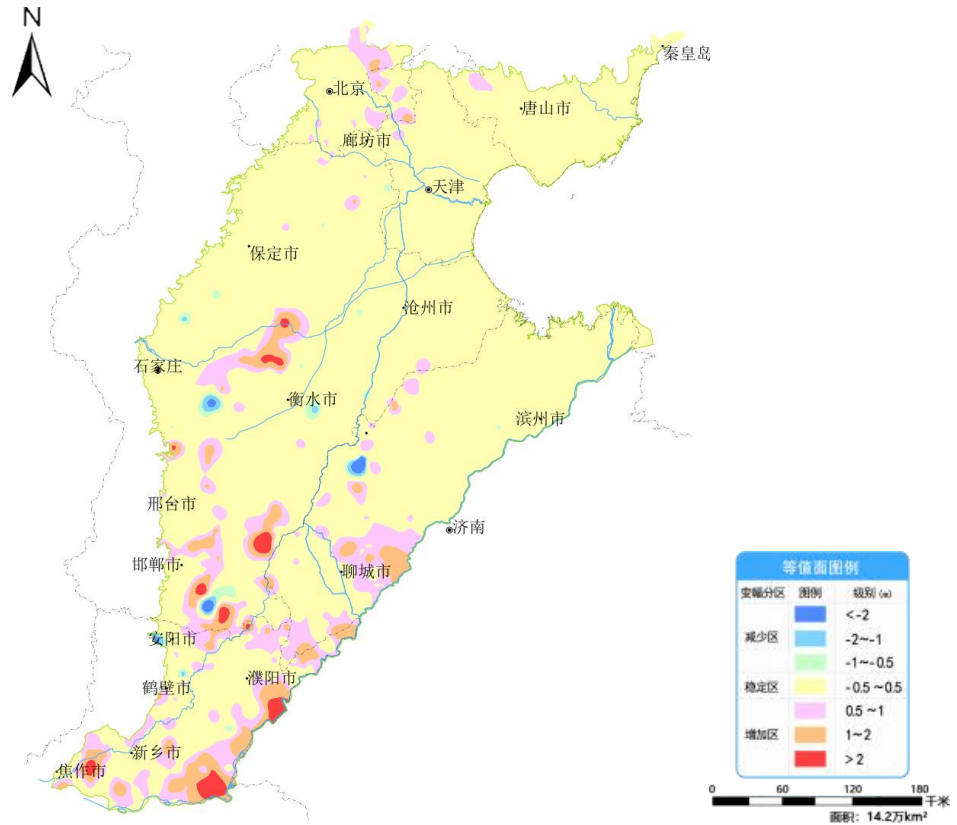
图 11 海河平原 3 月份与上月相比地下水埋深变幅图
