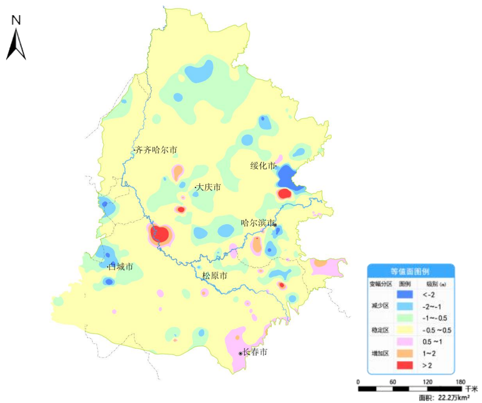
图6 松嫩平原3月份与去年同期相比地下水埋深变幅图
