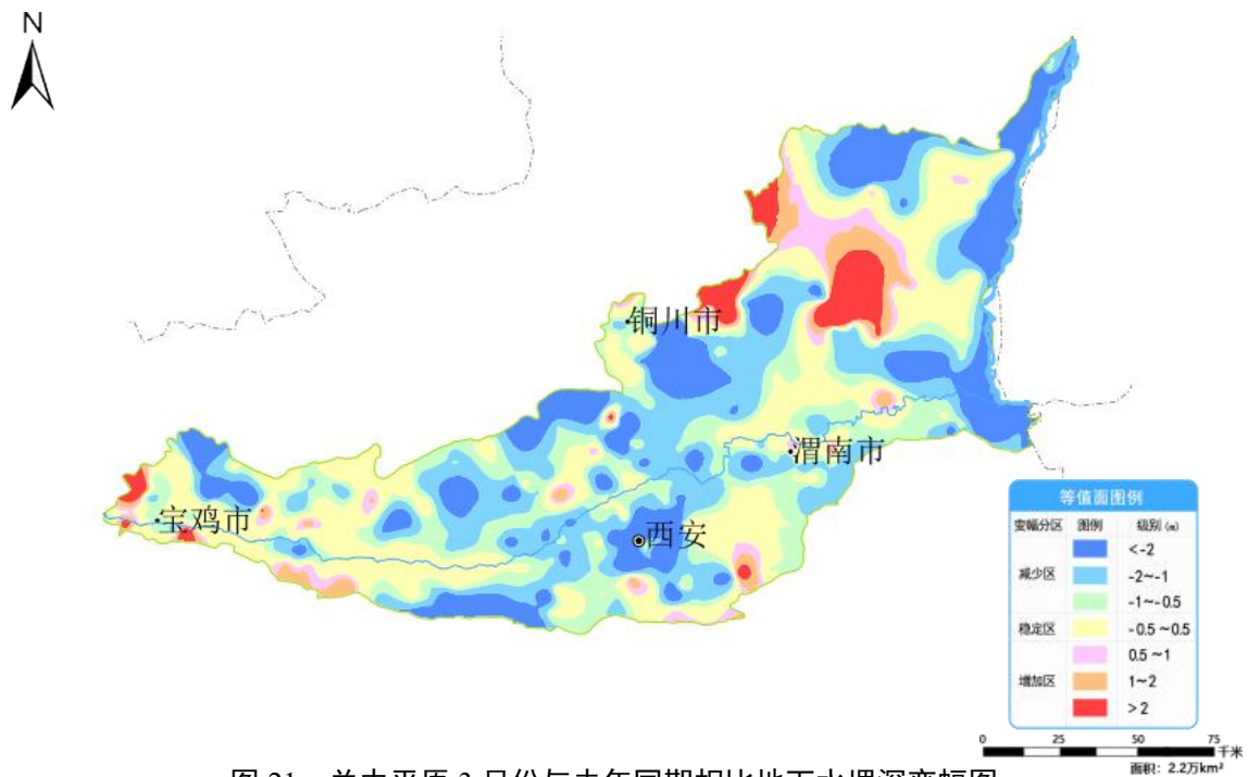
图 21 关中平原 3 月份与去年同期相比地下水埋深变幅图
