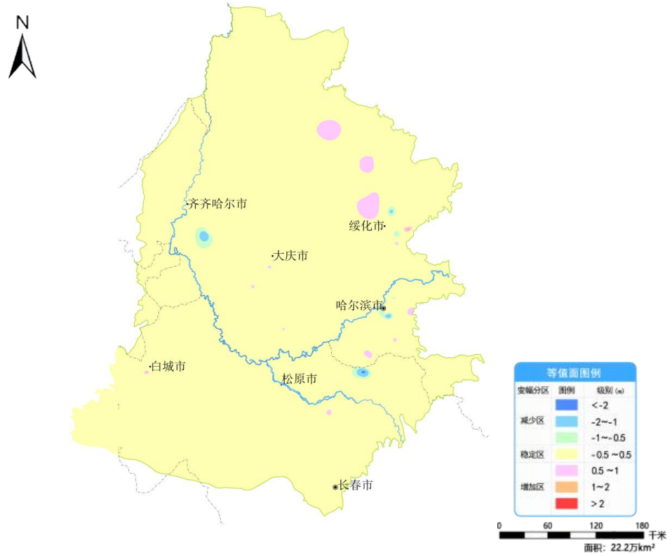
图5 松嫩平原3月份与上月相比地下水埋深变幅图
