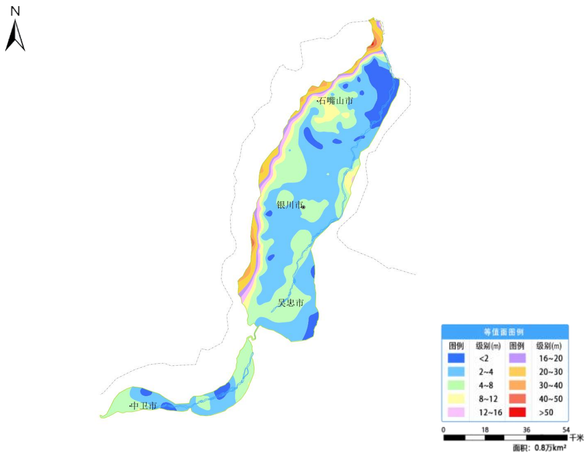
图 25 银川卫宁平原 3 月份地下水埋深等值面图
