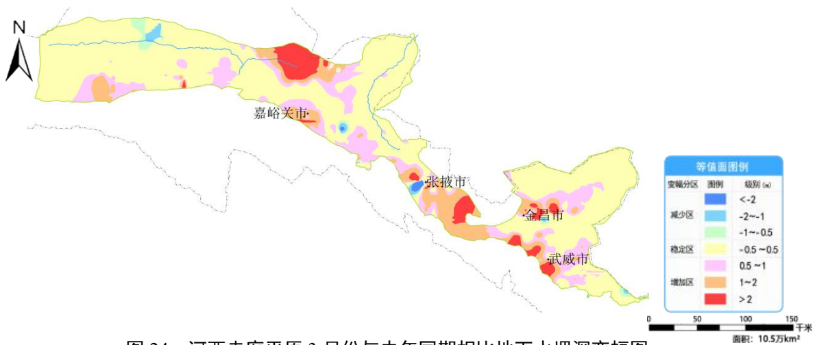
图24 河西走廊平原3月份与去年同期相比地下水埋深变幅图
