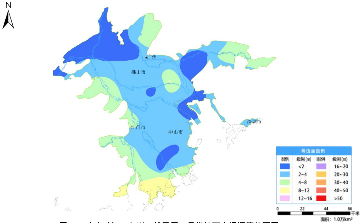
图 33 广东珠江三角洲一般平原 3 月份地下水埋深等值面图
