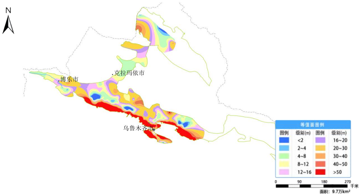
图 28 准噶尔盆地监控区 3 月份地下水埋深等值面图
