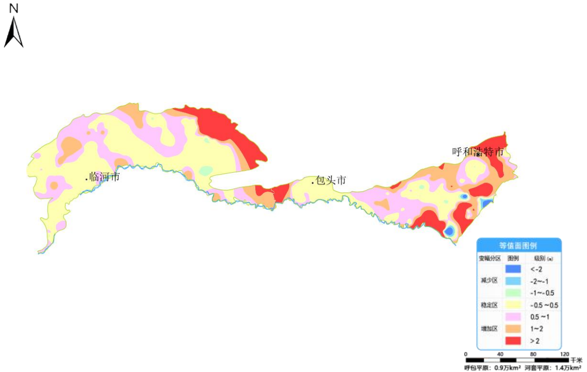
图 18 呼包平原和河套平原 3 月份与去年同期相比地下水埋深变幅图
