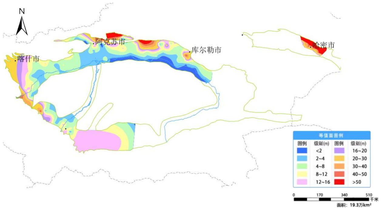
图 27 塔里木盆地监控区 3 月份地下水埋深等值面图
