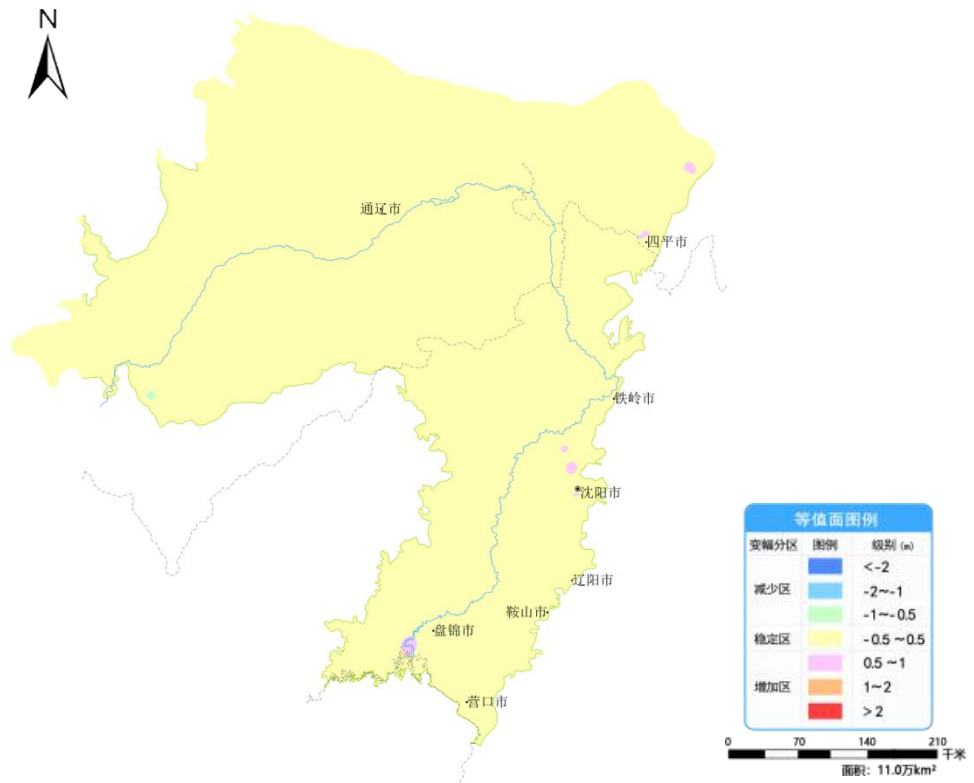
图 8 辽河平原 3 月份与上月相比地下水埋深变幅图
