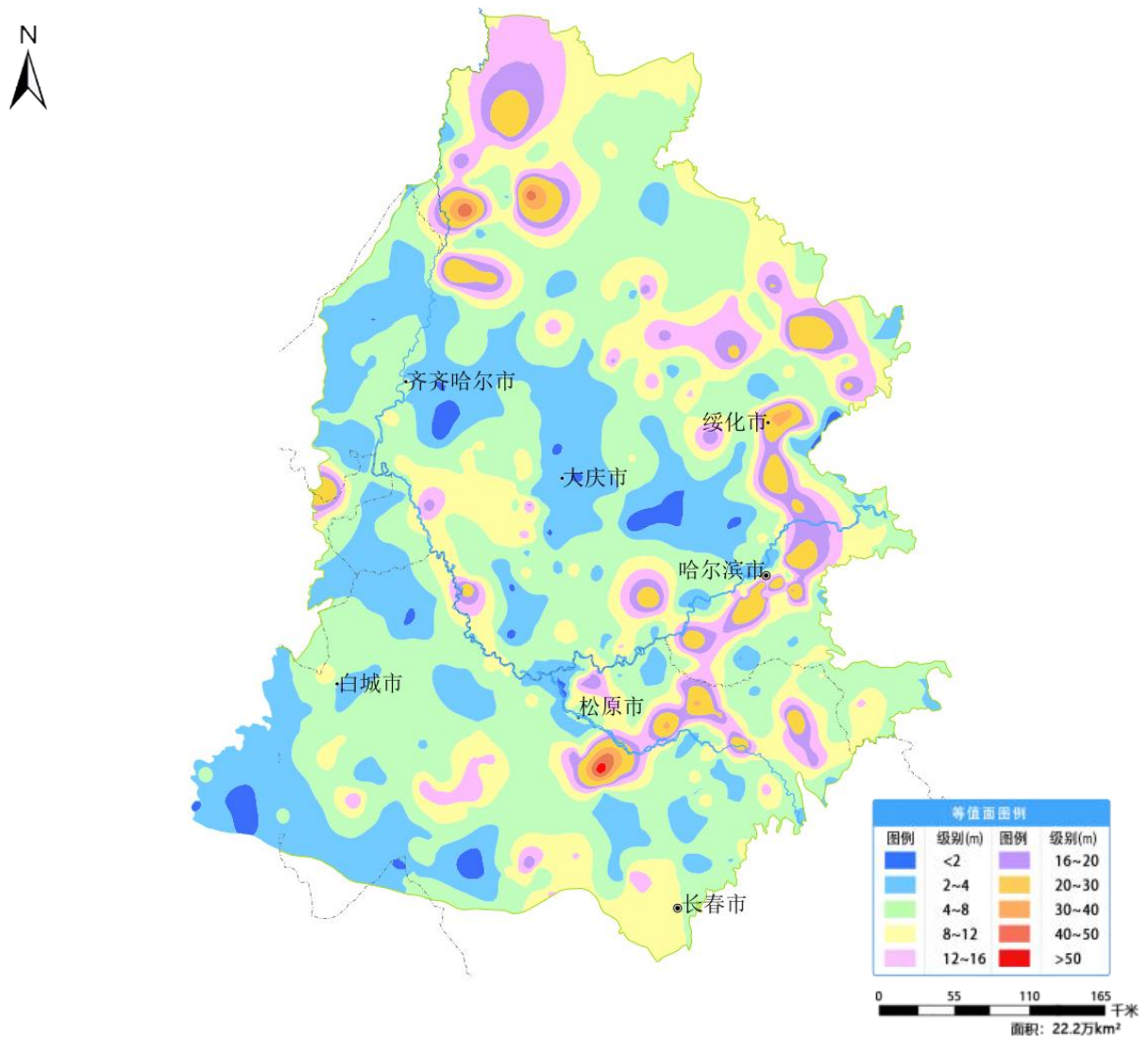
图 4 松嫩平原 3 月份地下水埋深等值面图
