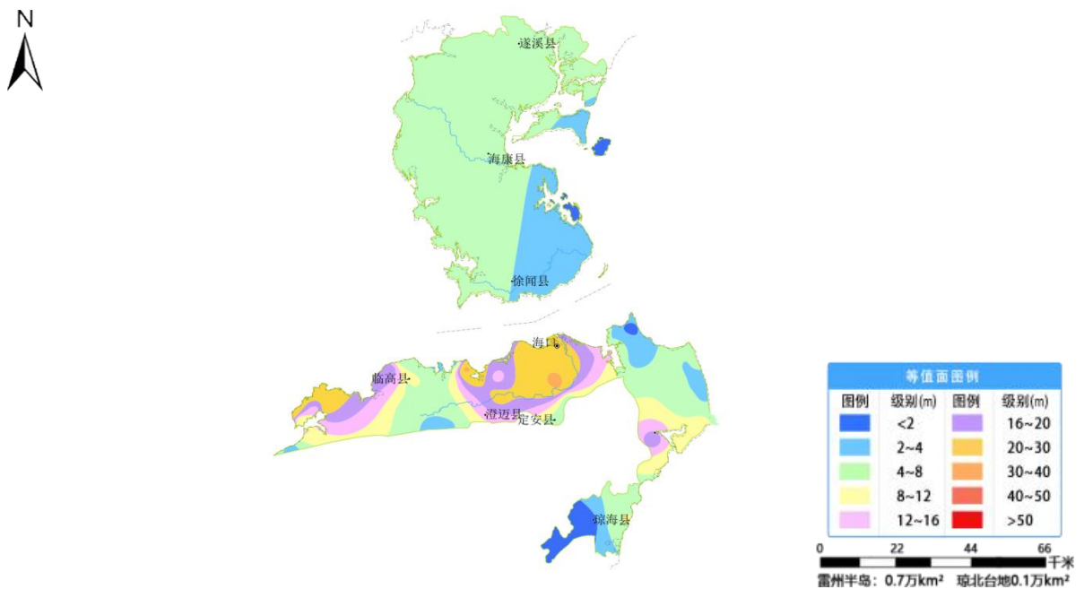
图 34 雷州半岛一般平原、琼北台地一般平原 3 月份地下水埋深等值面图
