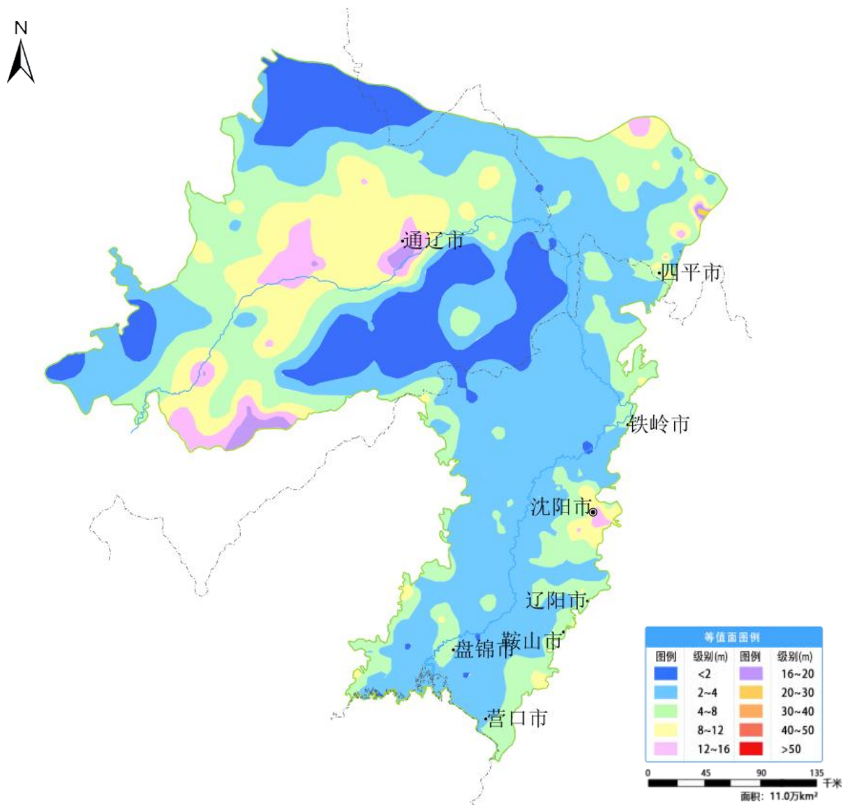
图 7 辽河平原 3 月份地下水埋深等值面图
