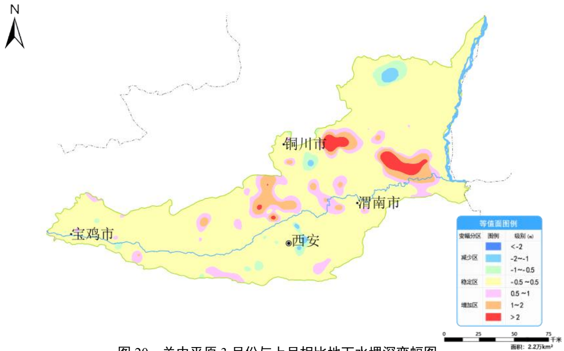
图 20 关中平原 3 月份与上月相比地下水埋深变幅图
