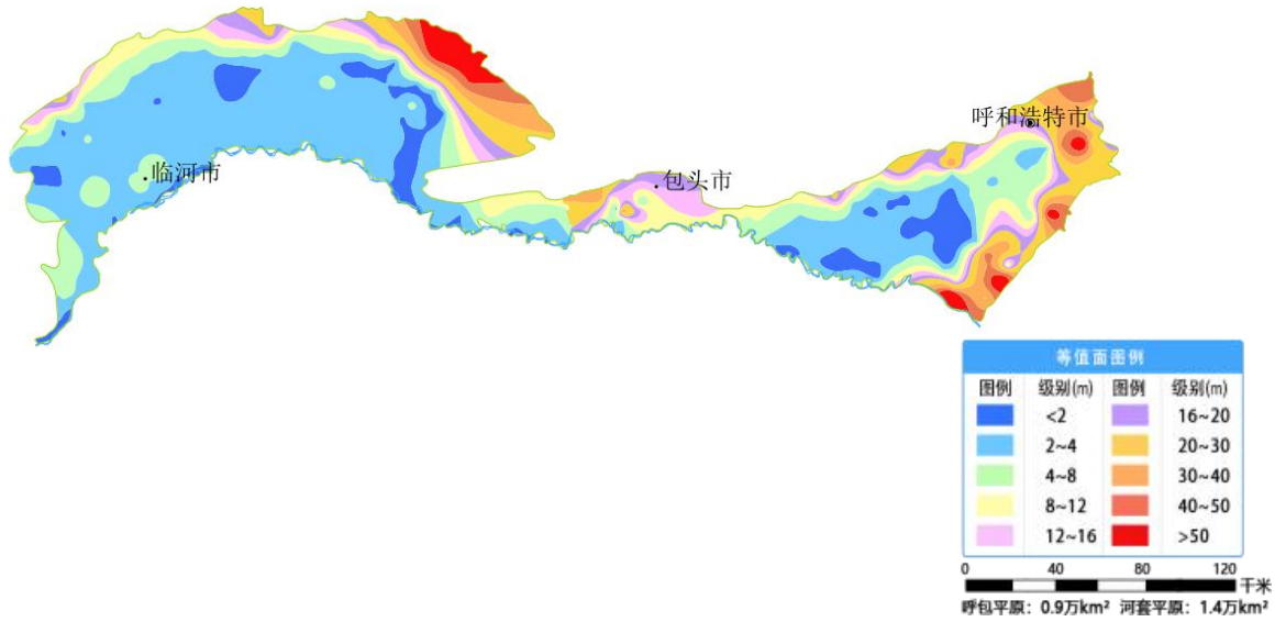
图 16 呼包平原和河套平原 3 月份地下水埋深等值面图
