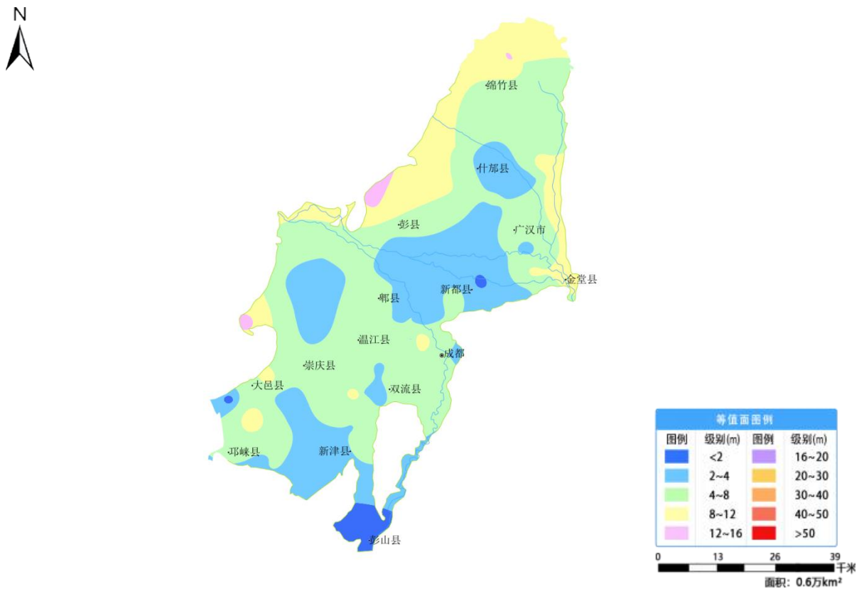
图 32 成都平原 3 月份地下水埋深等值面图
