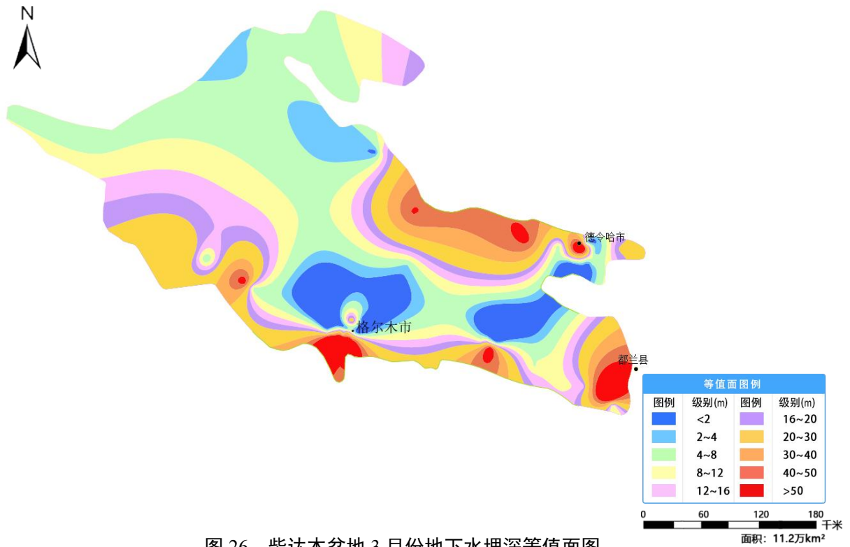
图 26 柴达木盆地 3 月份地下水埋深等值面图
