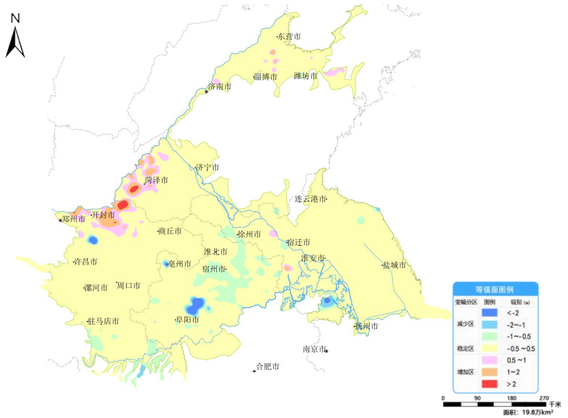
图 14 黄淮平原 3 月份与上月相比地下水埋深变幅图
