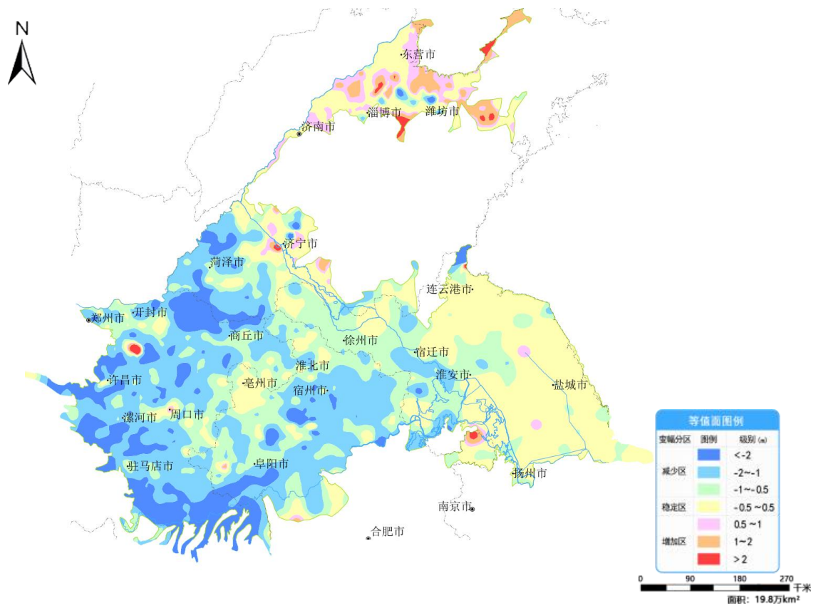
图 15 黄淮平原 3 月份与去年同期相比地下水埋深变幅图
