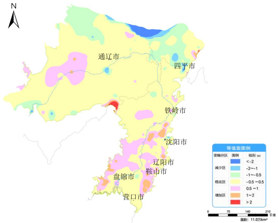
图 9 辽河平原 6 月份与去年同期相比地下水埋深变幅图
