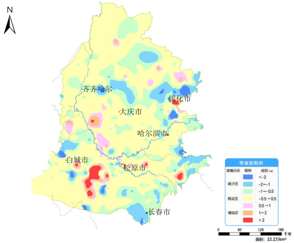
图5 松嫩平原6月份与上月相比地下水埋深变幅图
