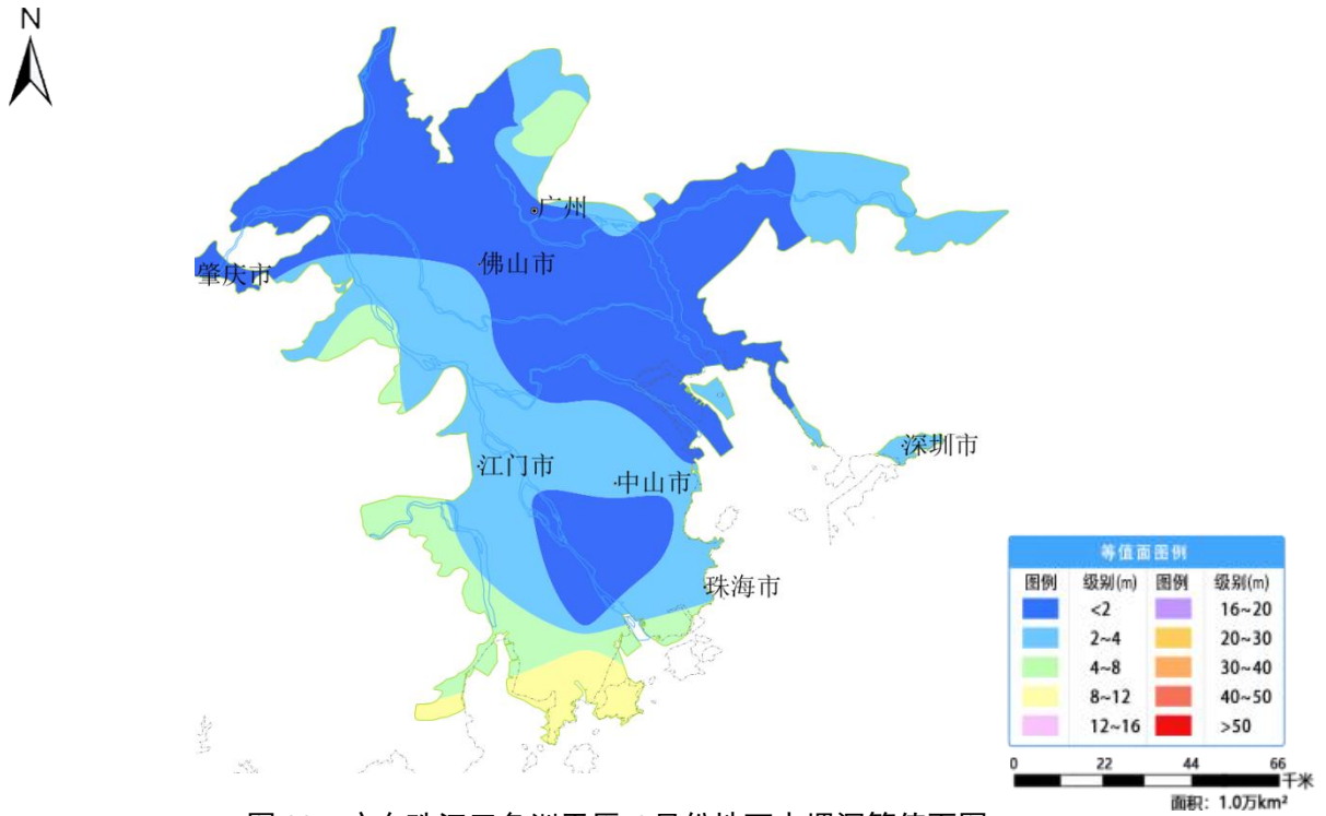
图 33 广东珠江三角洲平原 6 月份地下水埋深等值面图
