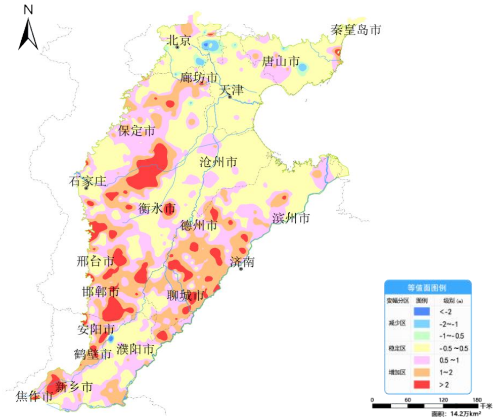
图 11 海河平原 6 月份与上月相比地下水埋深变幅图
