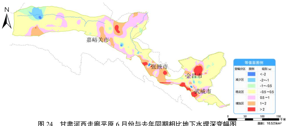
图 24 甘肃河西走廊平原 6 月份与去年同期相比地下水埋深变幅图
