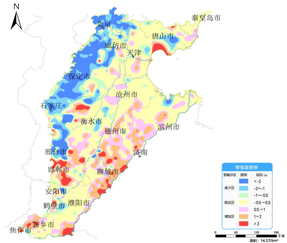
图 12 海河平原 6 月份与去年同期相比地下水埋深变幅图
