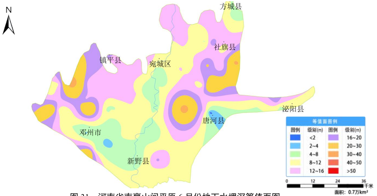
图 31 河南省南襄山间平原 6 月份地下水埋深等值面图
