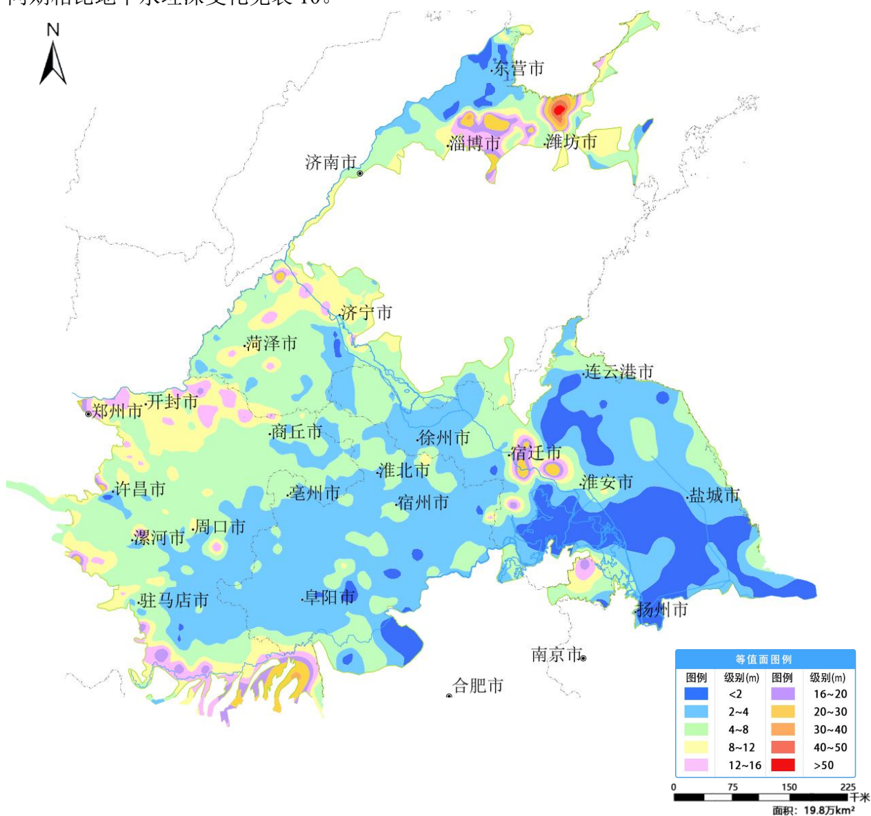
图13 黄淮平原6月份地下水埋深等值线图
