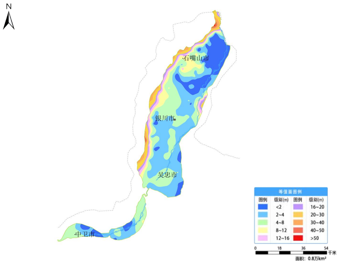
图 25 宁夏银川卫宁平原 6 月份地下水埋深等值面图
