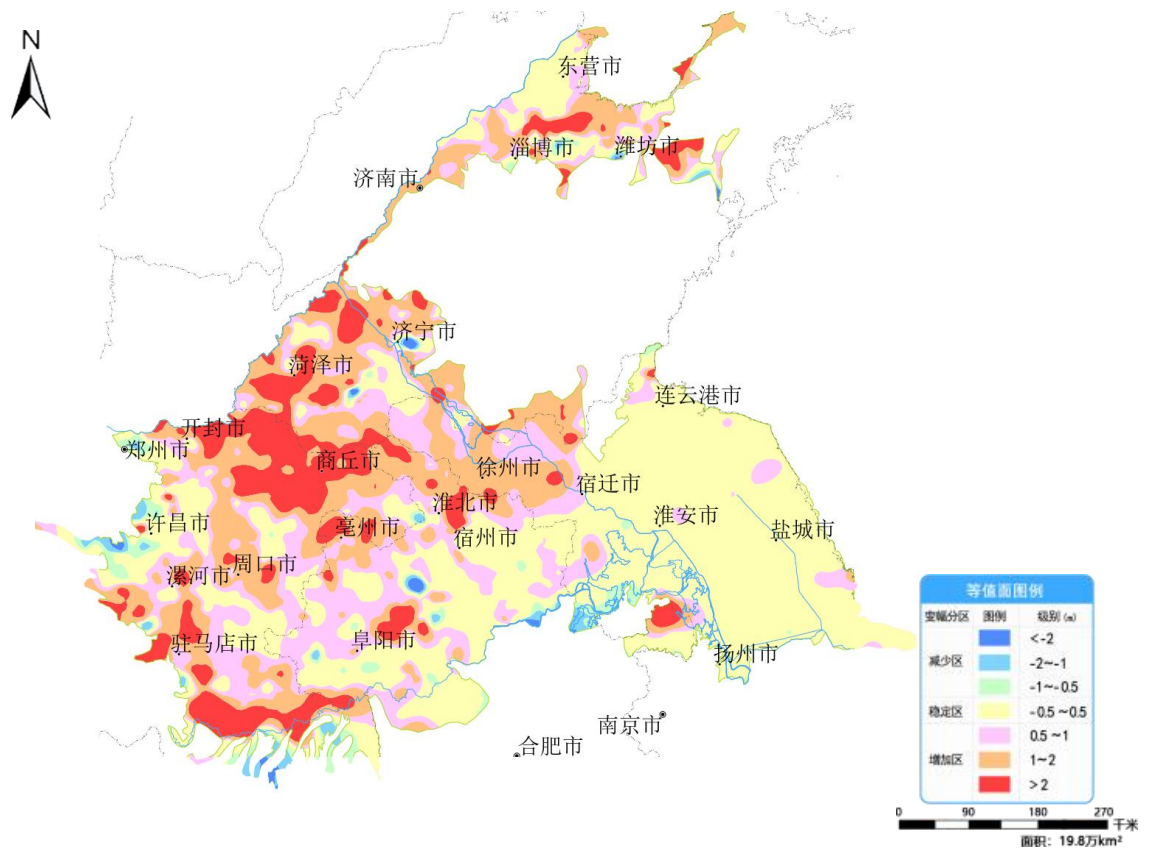
图 15 黄淮平原 6 月份与去年同期相比地下水埋深变幅图
