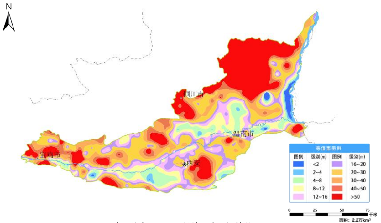
图 19 陕西关中平原 6 月份地下水埋深等值面图
