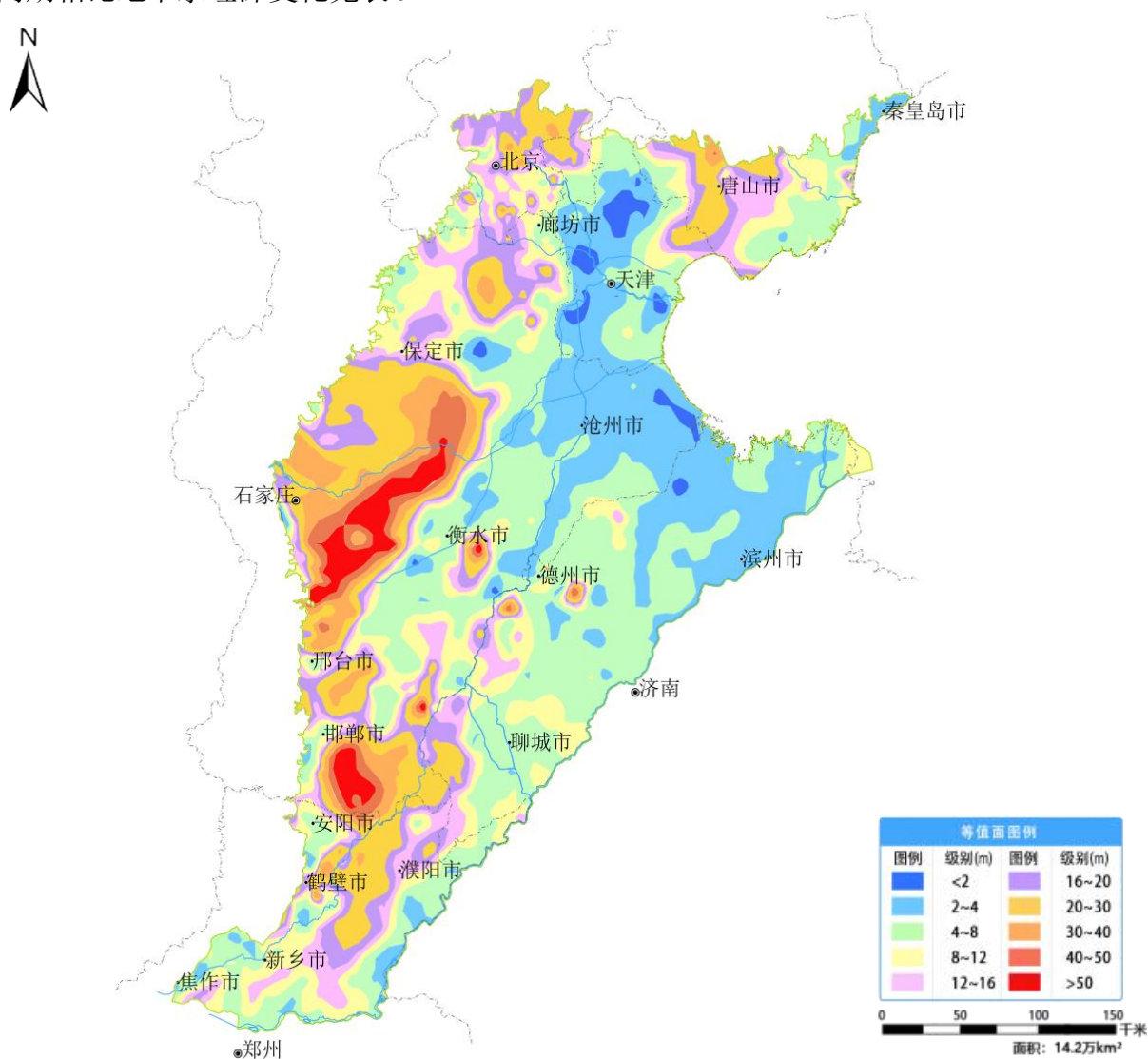
图 10 海河平原 6 月份地下水埋深等值面图
