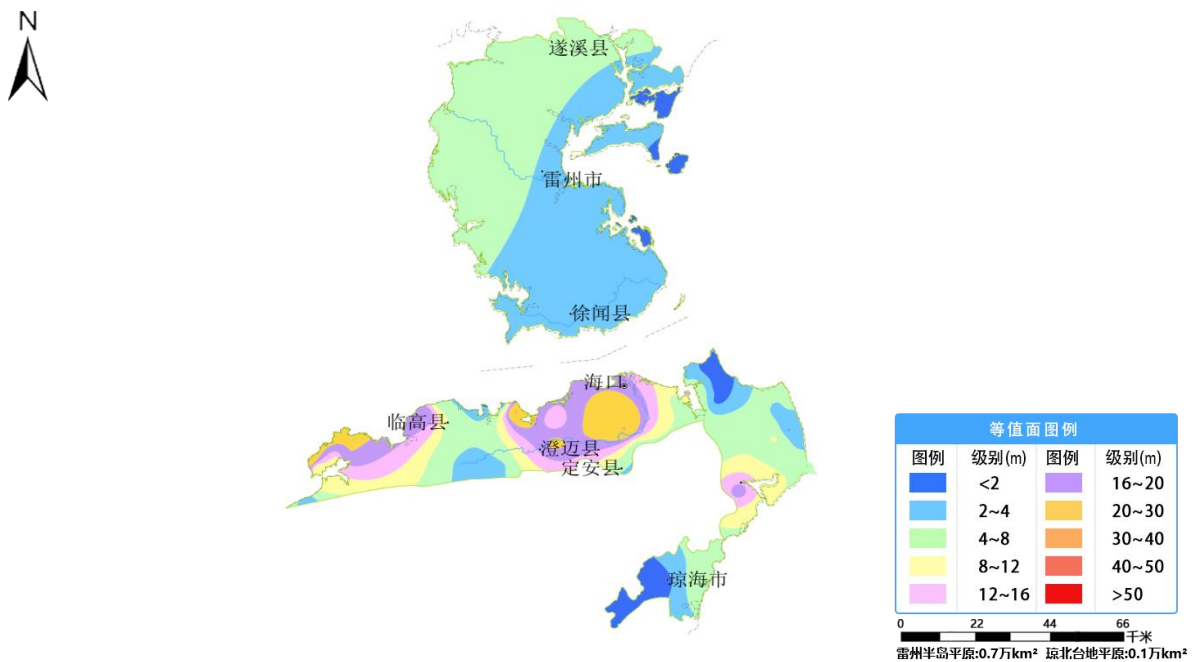
图 34 雷州半岛平原和琼北台地平原 6 月份地下水埋深等值面图
