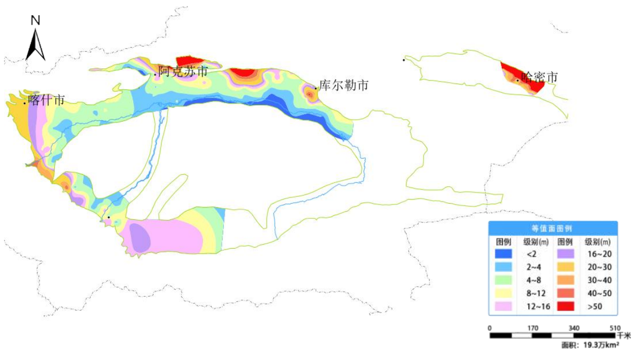
图 27 新疆塔里木盆地监控区 6 月份地下水埋深等值面图
