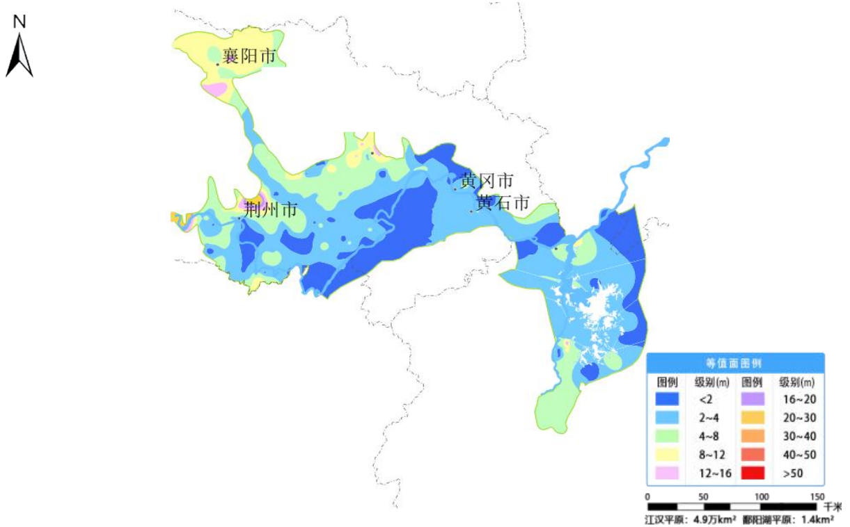
图 29 江汉平原和鄱阳湖平原 6 月份地下水埋深等值面图
