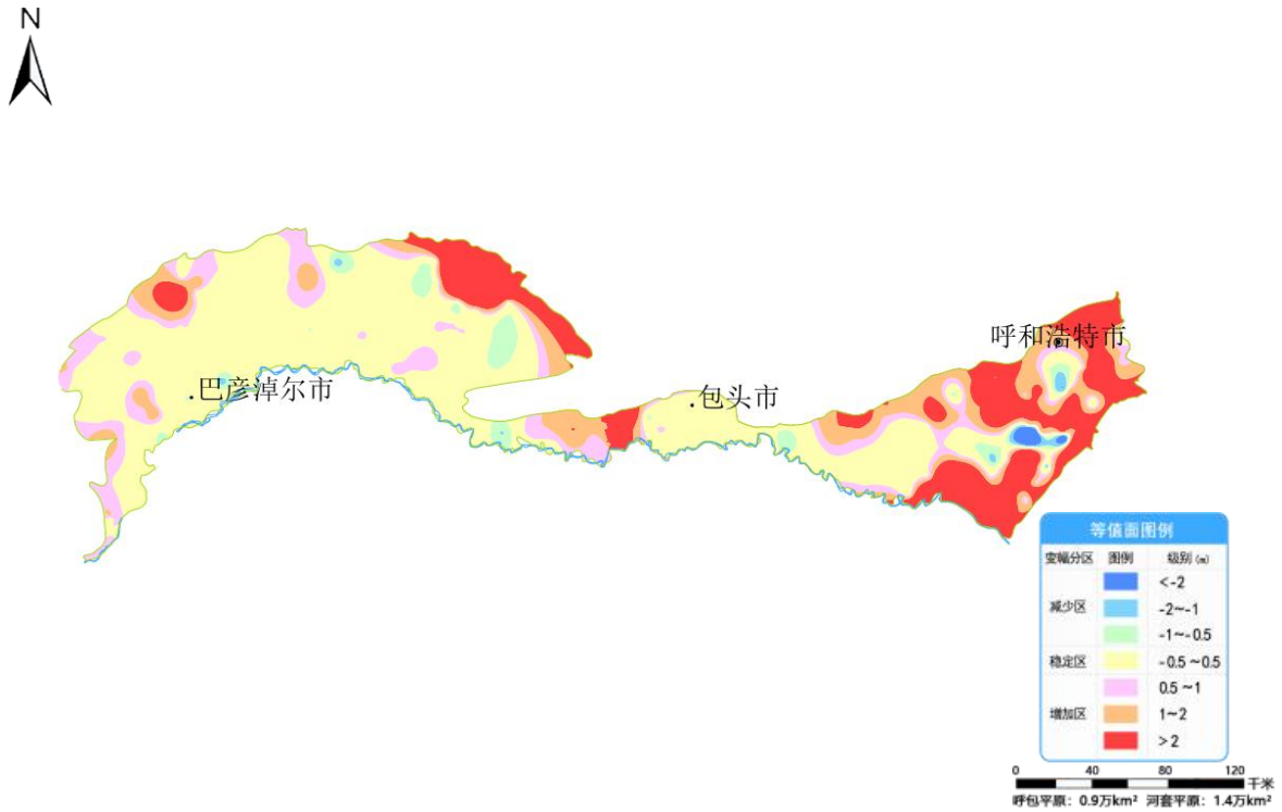
图 18 内蒙古呼包平原及河套平原 6 月份与去年同期相比地下水埋深变幅图
