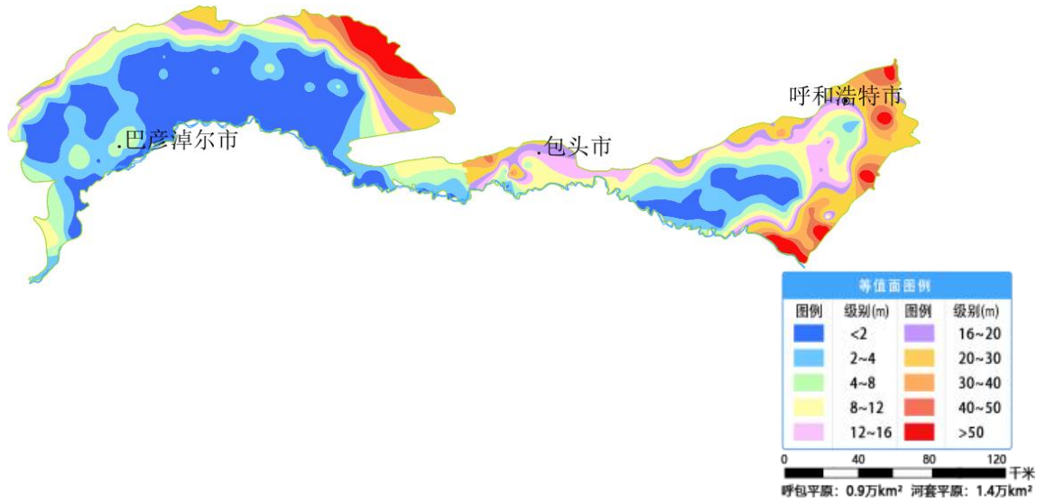
图 16 内蒙古呼包平原及河套平原 6 月份地下水埋深等值面图
