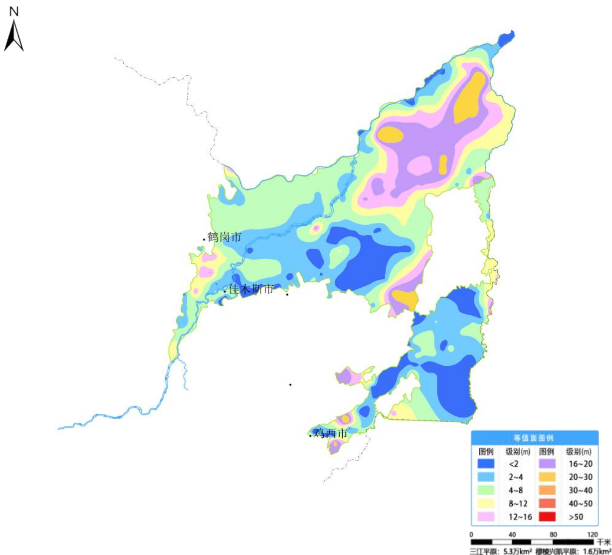
图 1 三江平原和穆棱兴凯平原 6 月份地下水埋深等值面图
