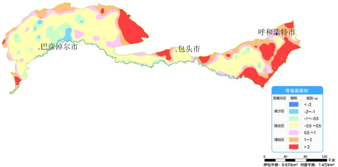
图 17 内蒙古呼包平原及河套平原 6 月份与上月相比地下水埋深变幅图
