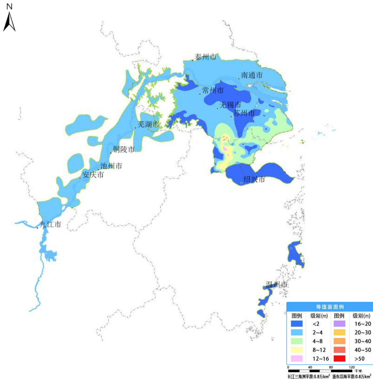
图 30 长江三角洲平原和浙东沿海平原 6 月份地下水埋深等值面图
