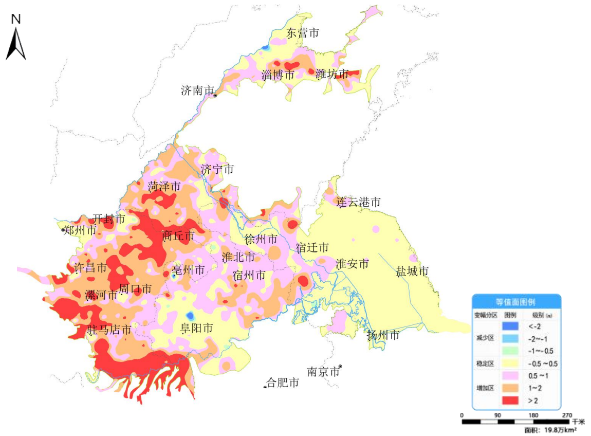
图 14 黄淮平原 6 月份与上月相比地下水埋深变幅图
