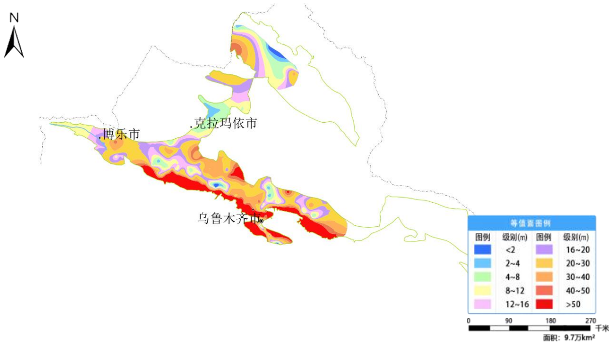
图 28 新疆准噶尔盆地监控区 6 月份地下水埋深等值面图
