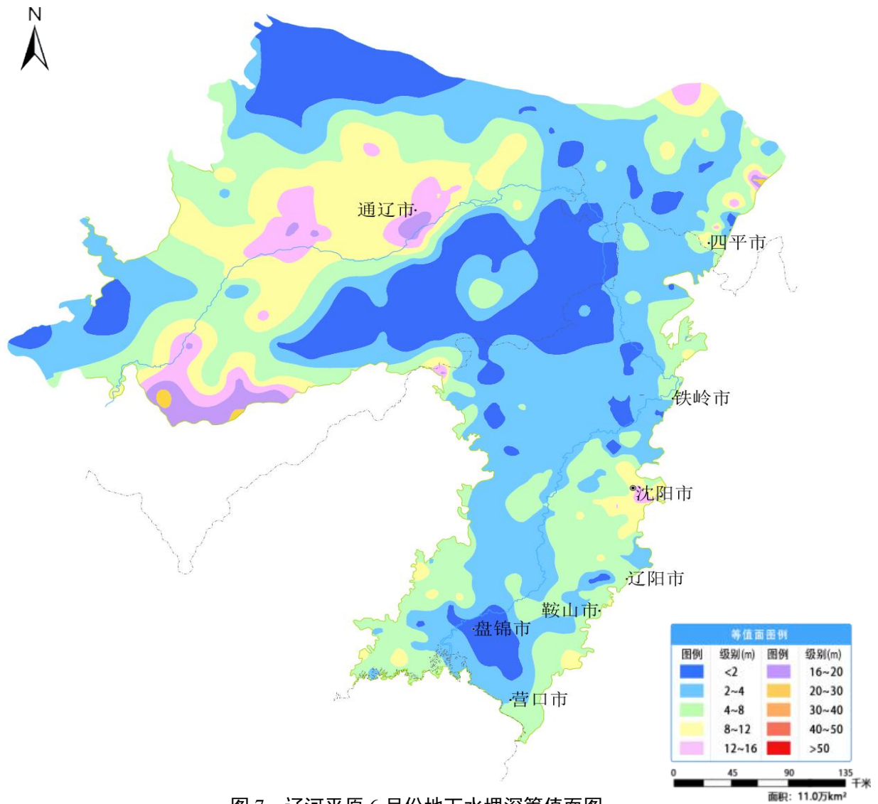
图 7 辽河平原 6 月份地下水埋深等值面图
