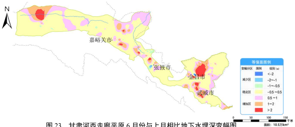
图 23 甘肃河西走廊平原 6 月份与上月相比地下水埋深变幅图
