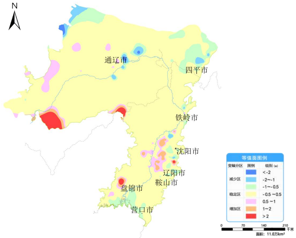
图 8 辽河平原 6 月份与上月相比地下水埋深变幅图
