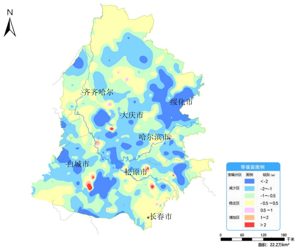
图6 松嫩平原6月份与去年同期相比地下水埋深变幅图
