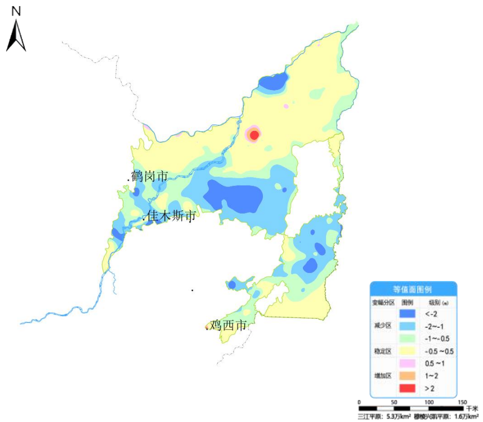
图3 三江平原和穆棱兴凯平原6月份与去年同期相比地下水埋深变幅图
