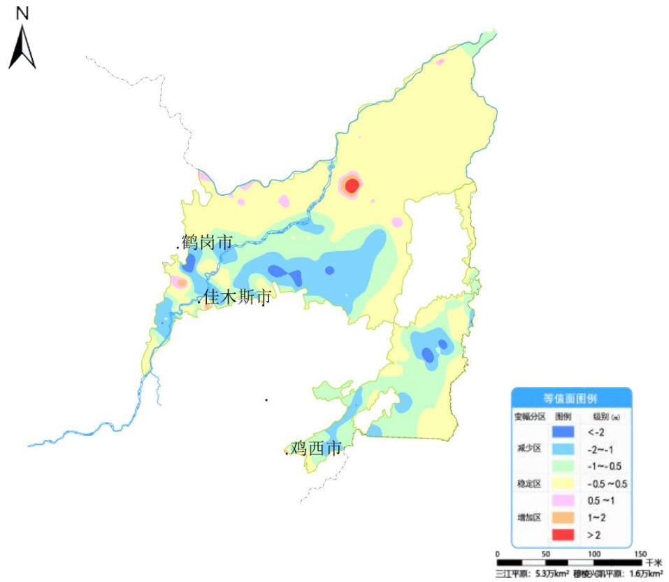
图2 三江平原和穆棱兴凯平原6月份与上月相比地下水埋深变幅图
