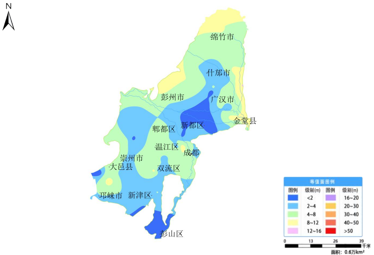
图 32 成都平原 6 月份地下水埋深等值面图
