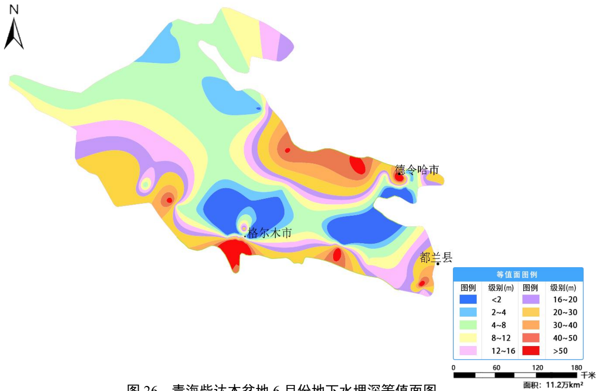
图 26 青海柴达木盆地 6 月份地下水埋深等值面图
