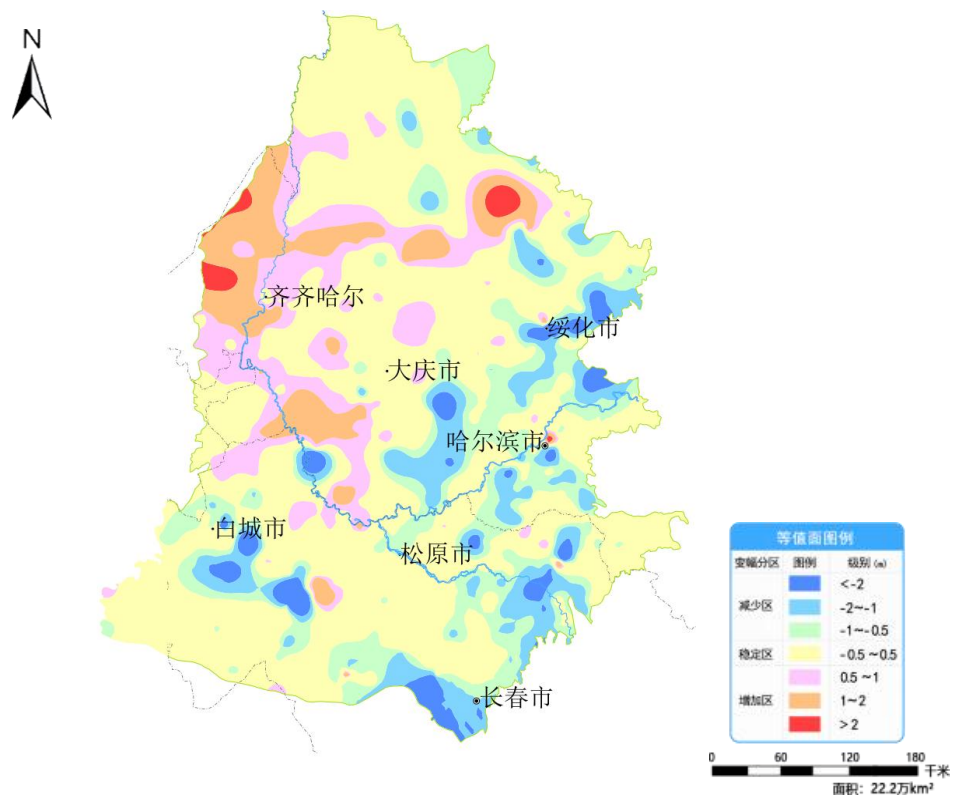
图 6 松嫩平原 8 月份与去年同期相比地下水埋深变幅图
