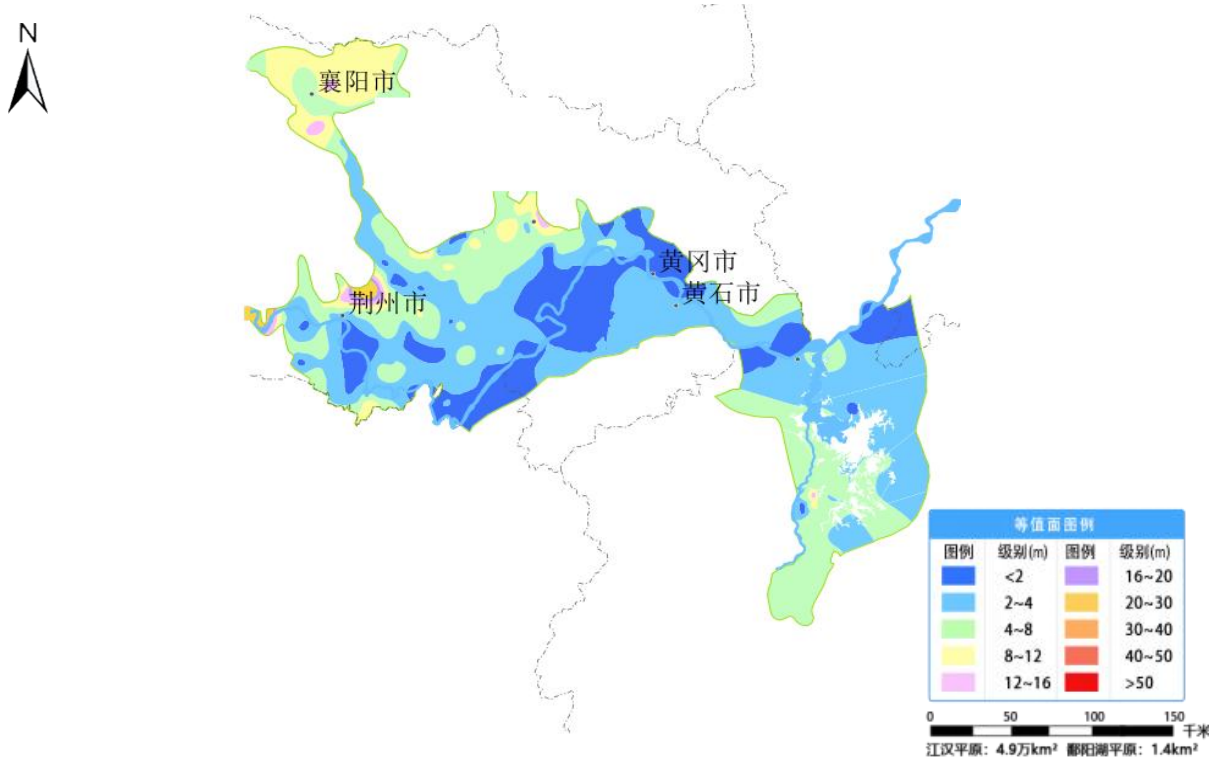
图 29 江汉平原和鄱阳湖平原 8 月份地下水埋深等值面图
