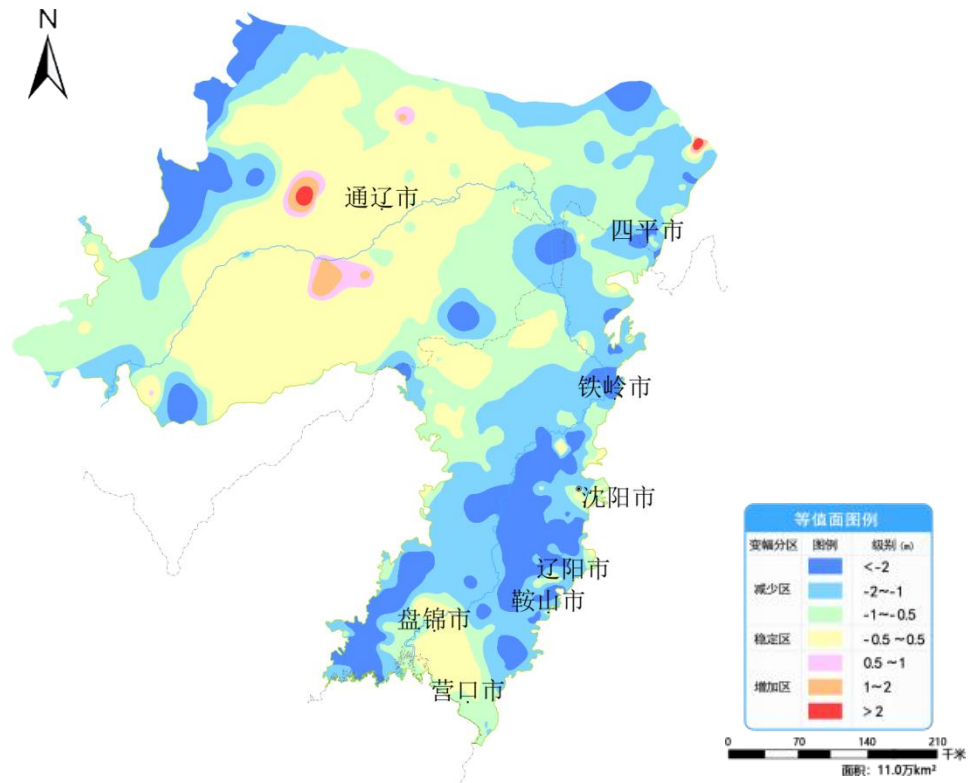
图8 辽河平原8月份与上月相比地下水埋深变幅图
