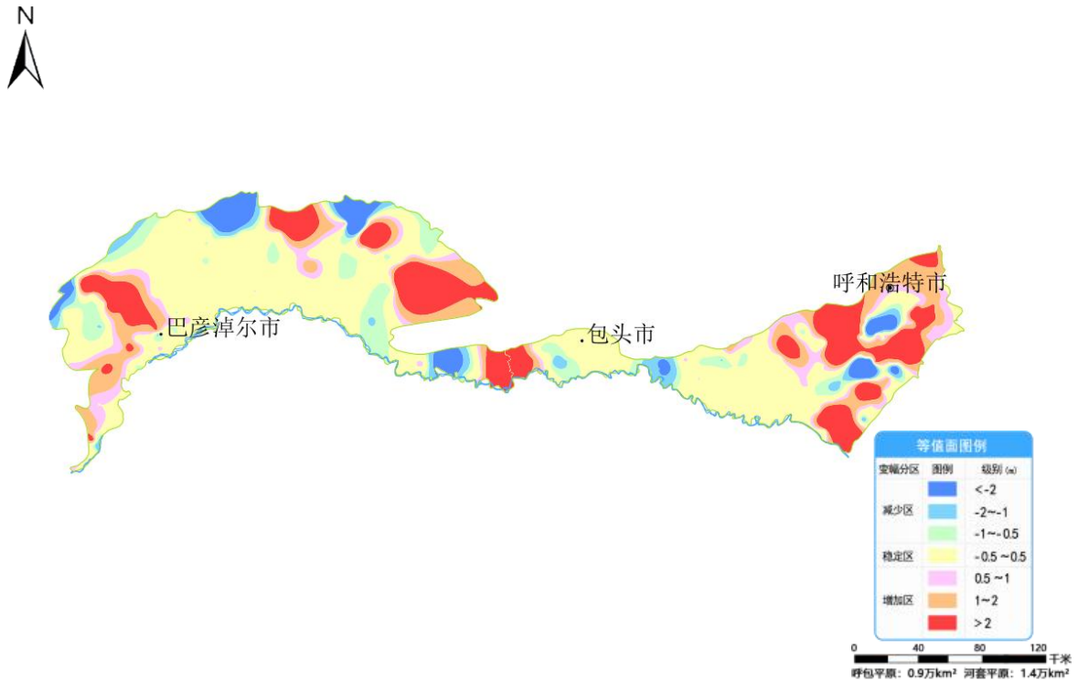
图 18 内蒙古呼包平原及河套平原 8 月份与去年同期相比地下水埋深变幅图
