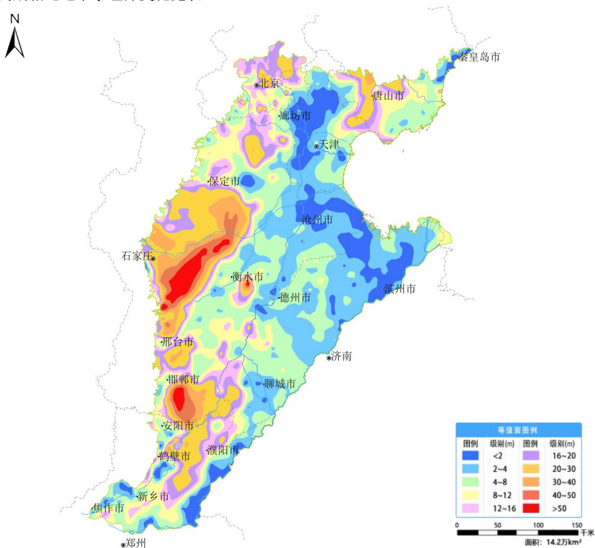
图 10 海河平原 8 月份地下水埋深等值面图
