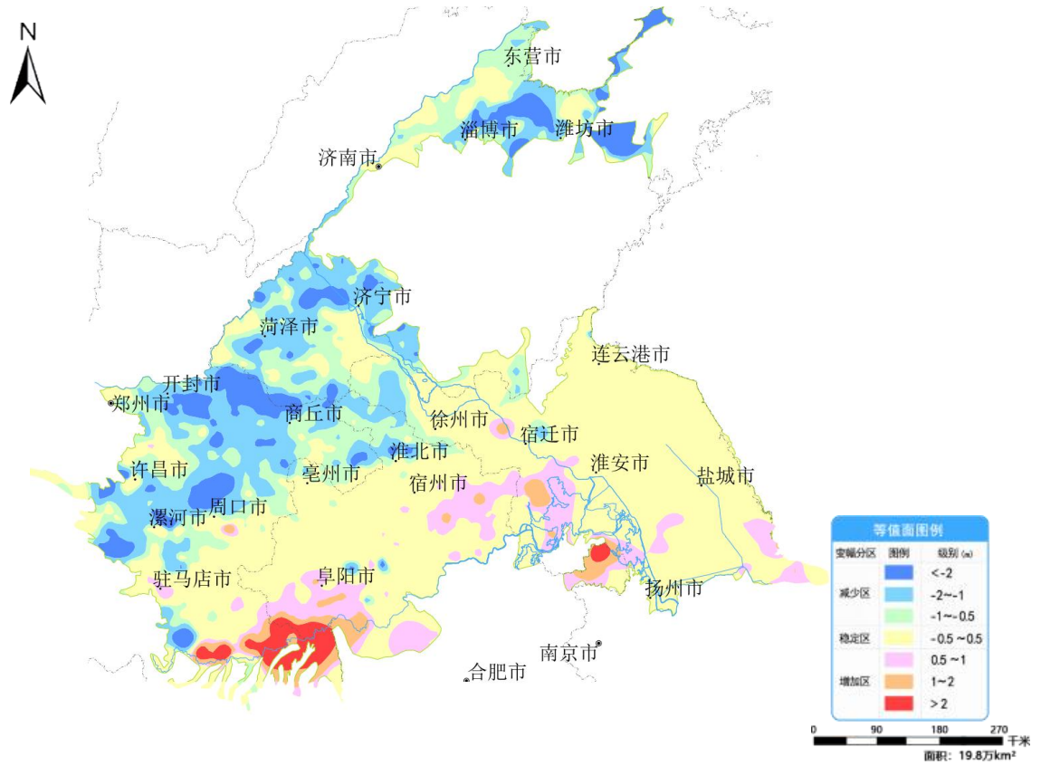
图 14 黄淮平原 8 月份与上月相比地下水埋深变幅图
