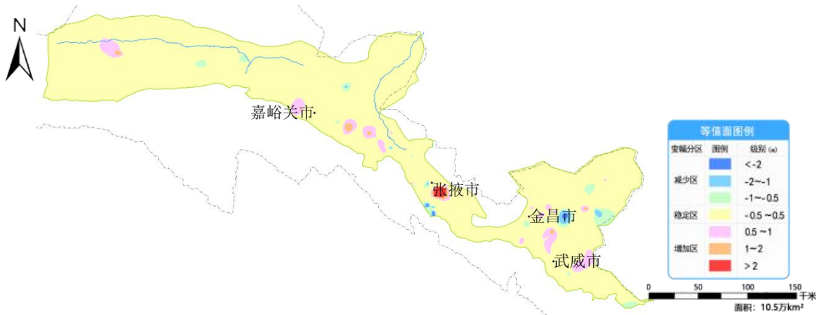
图 23 甘肃河西走廊平原 8 月份与上月相比地下水埋深变幅图
