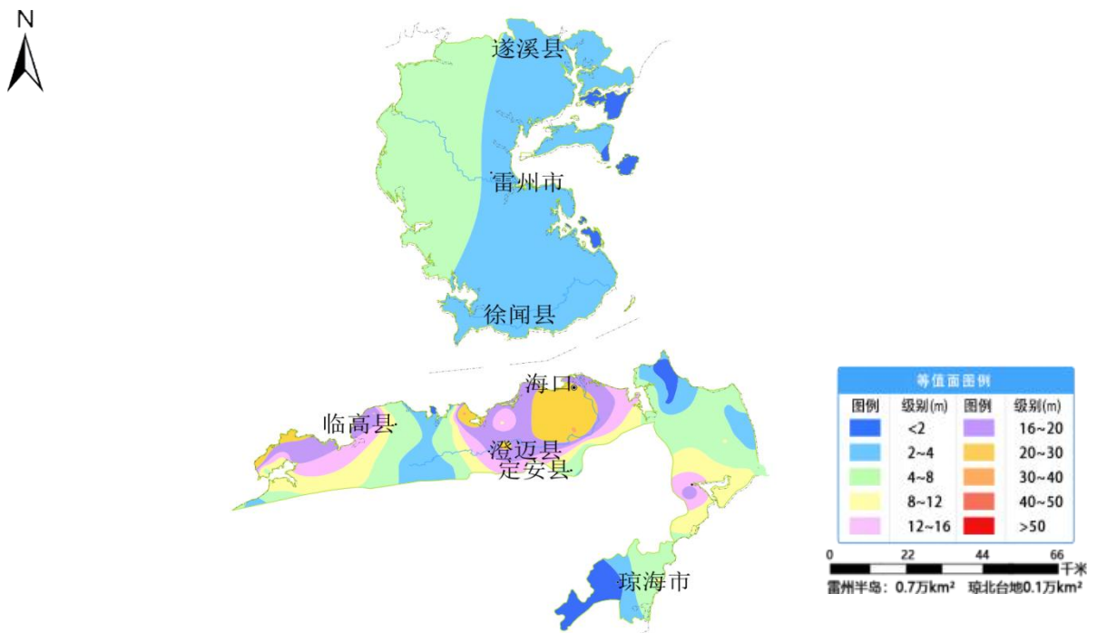
图 34 雷州半岛平原和琼北台地平原 8 月份地下水埋深等值面图
