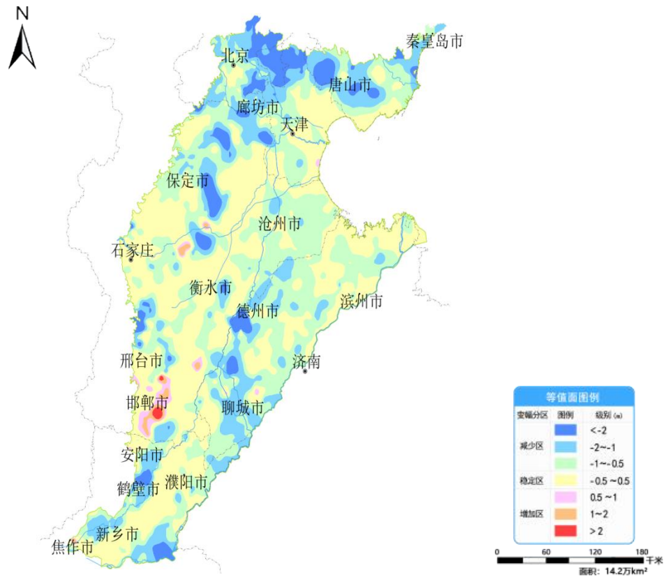
图 11 海河平原 8 月份与上月相比地下水埋深变幅图
