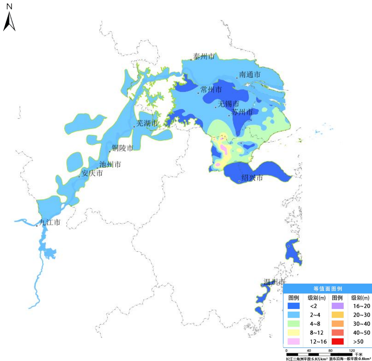
图 30 长江三角洲平原和浙东沿海平原 8 月份地下水埋深等值面图
