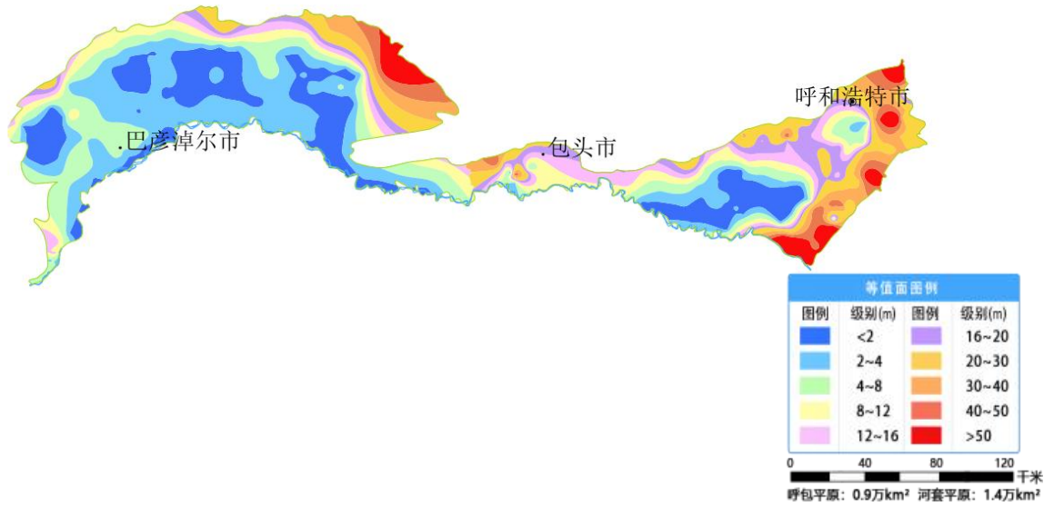
图 16 内蒙古呼包平原及河套平原 8 月份地下水埋深等值面图
