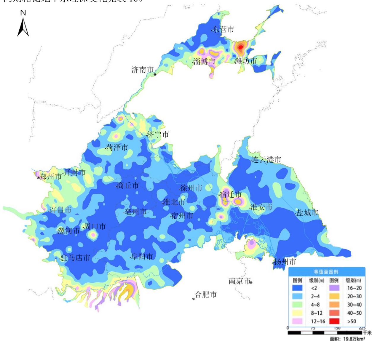
图13 黄淮平原8月份地下水埋深等值面图
