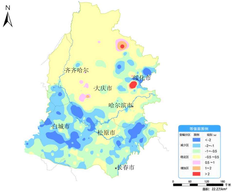
图 5 松嫩平原 8 月份与上月相比地下水埋深变幅图
