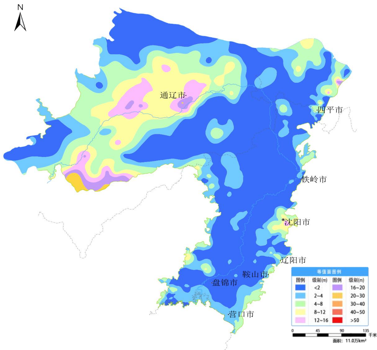
图 7 辽河平原 8 月份地下水埋深等值面图
