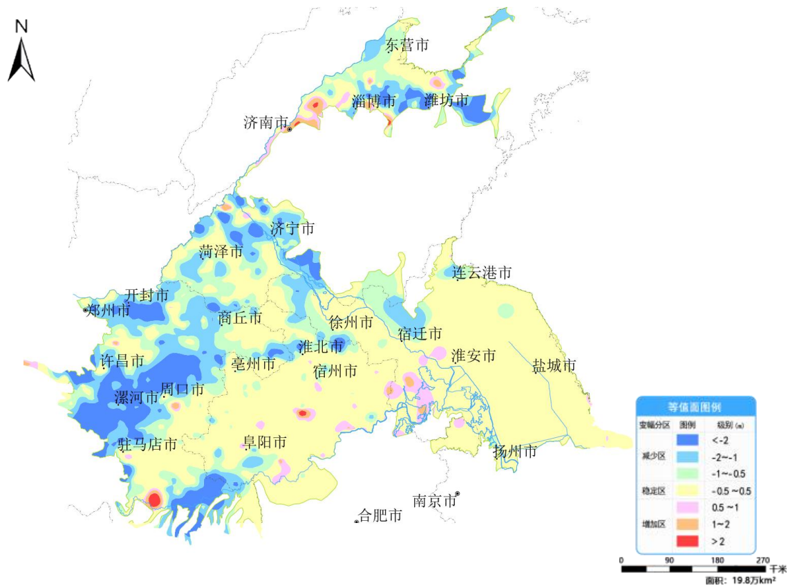
图 15 黄淮平原 8 月份与去年同期相比地下水埋深变幅图
