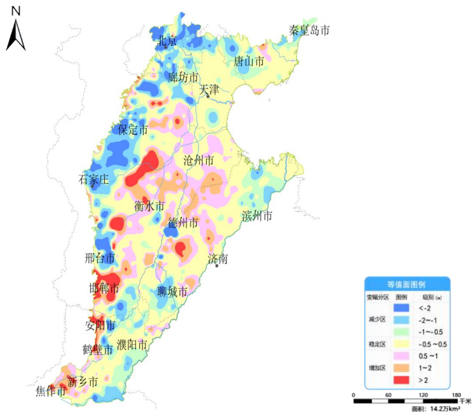
图 12 海河平原 8 月份与去年同期相比地下水埋深变幅图
