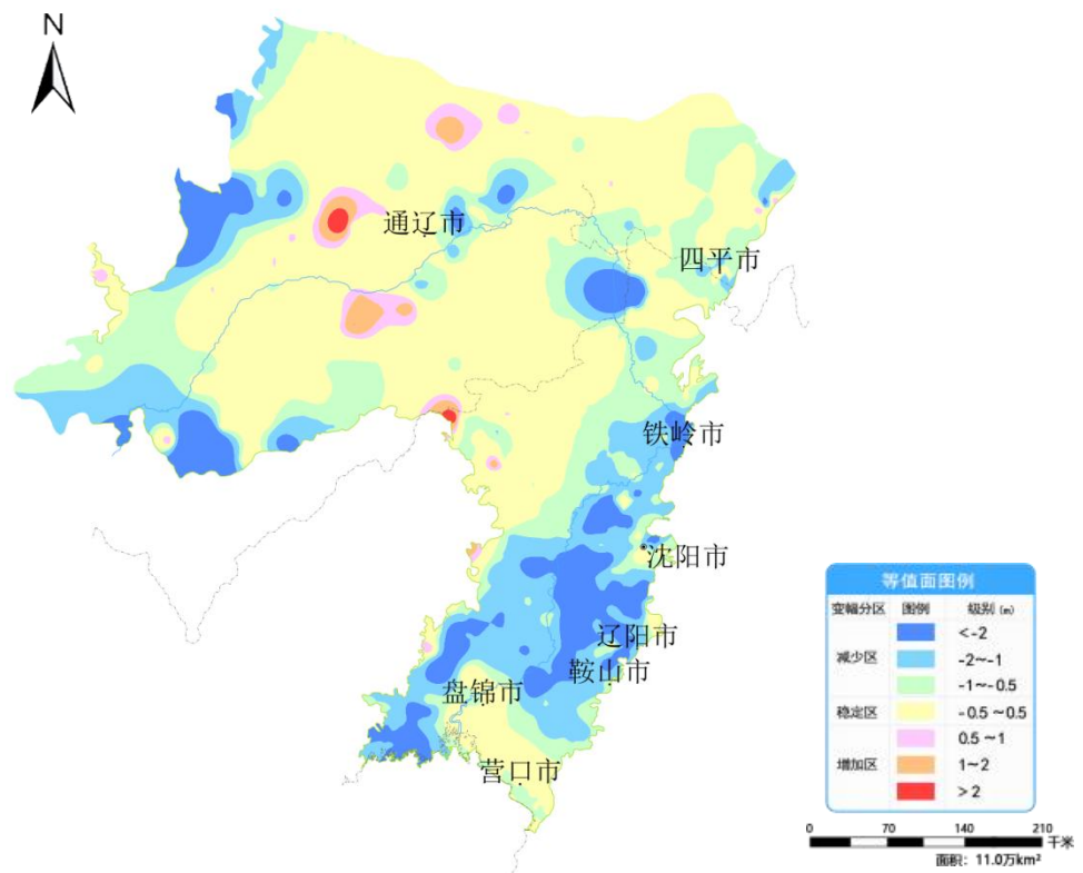
图9 辽河平原8月份与去年同期相比地下水埋深变幅图
