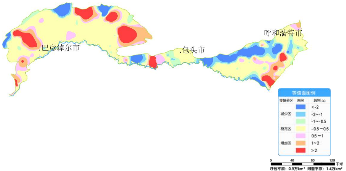
图 17 内蒙古呼包平原及河套平原 8 月份与上月相比地下水埋深变幅图
