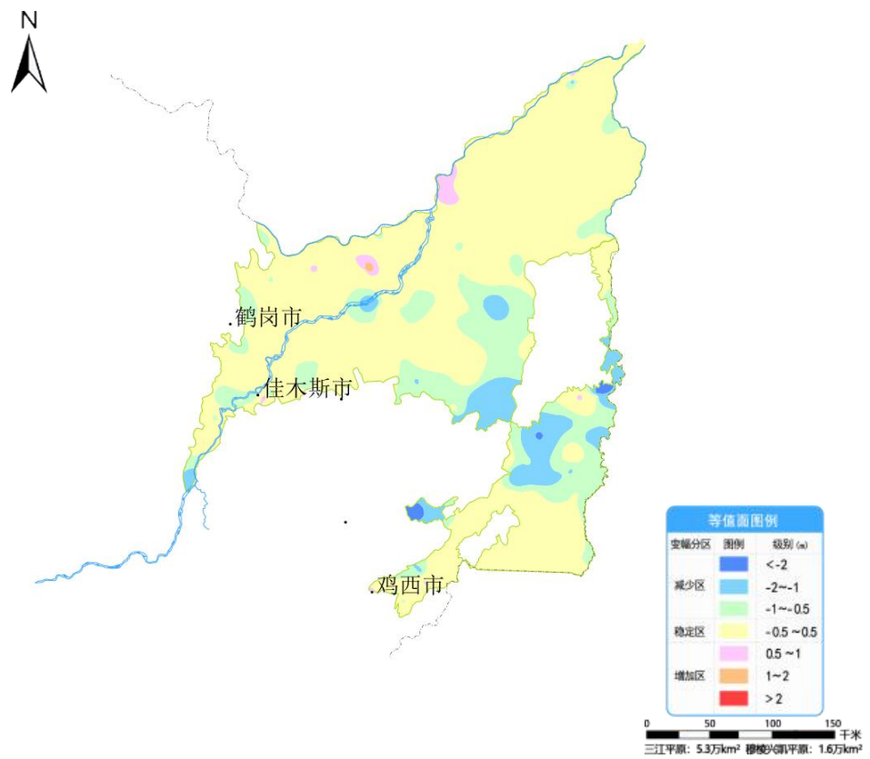
图3 三江平原和穆棱兴凯平原8月份与去年同期相比地下水埋深变幅图
