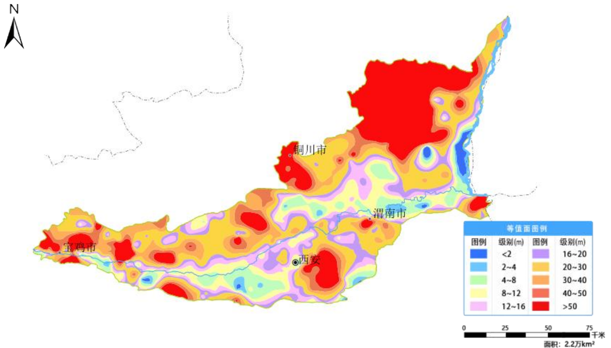
图 19 陕西关中平原 8 月份地下水埋深等值面图
