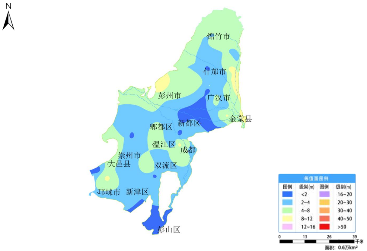
图 32 成都平原 8 月份地下水埋深等值面图
