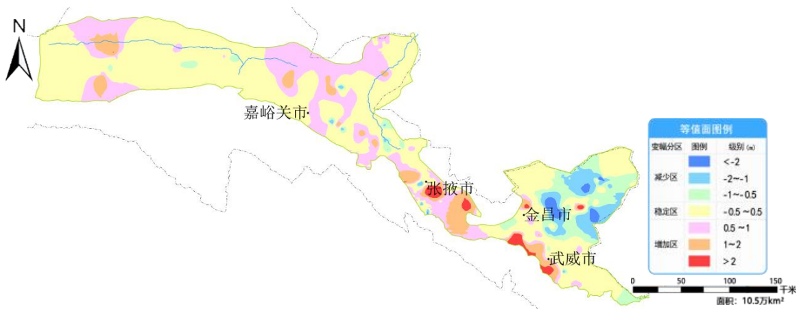
图 24 甘肃河西走廊平原 8 月份与去年同期相比地下水埋深变幅图
