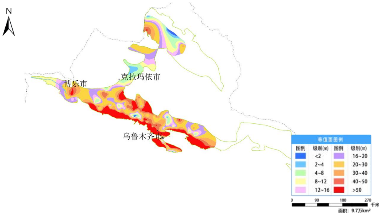
图 28 新疆准噶尔盆地监控区 8 月份地下水埋深等值面图
