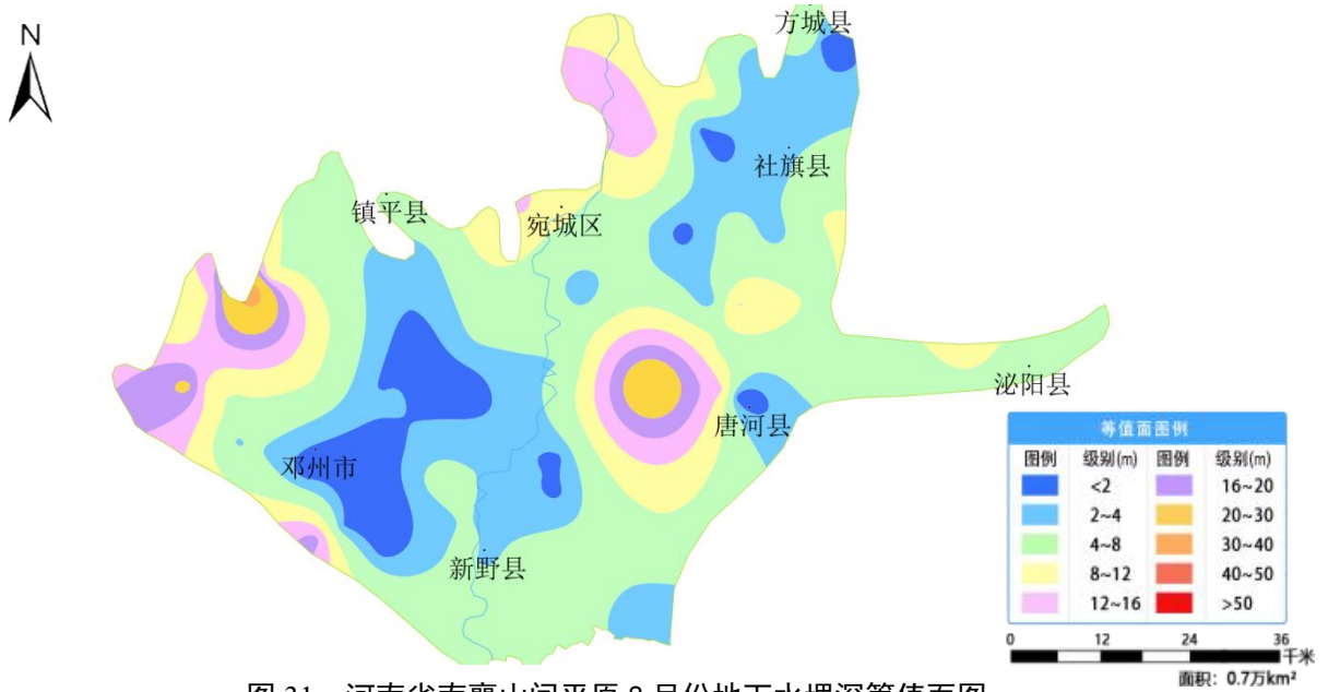
图 31 河南省南襄山间平原 8 月份地下水埋深等值面图
