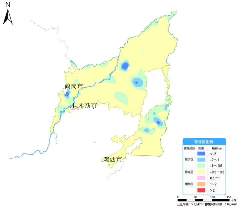
图2 三江平原和穆棱兴凯平原8月份与上月相比地下水埋深变幅图
