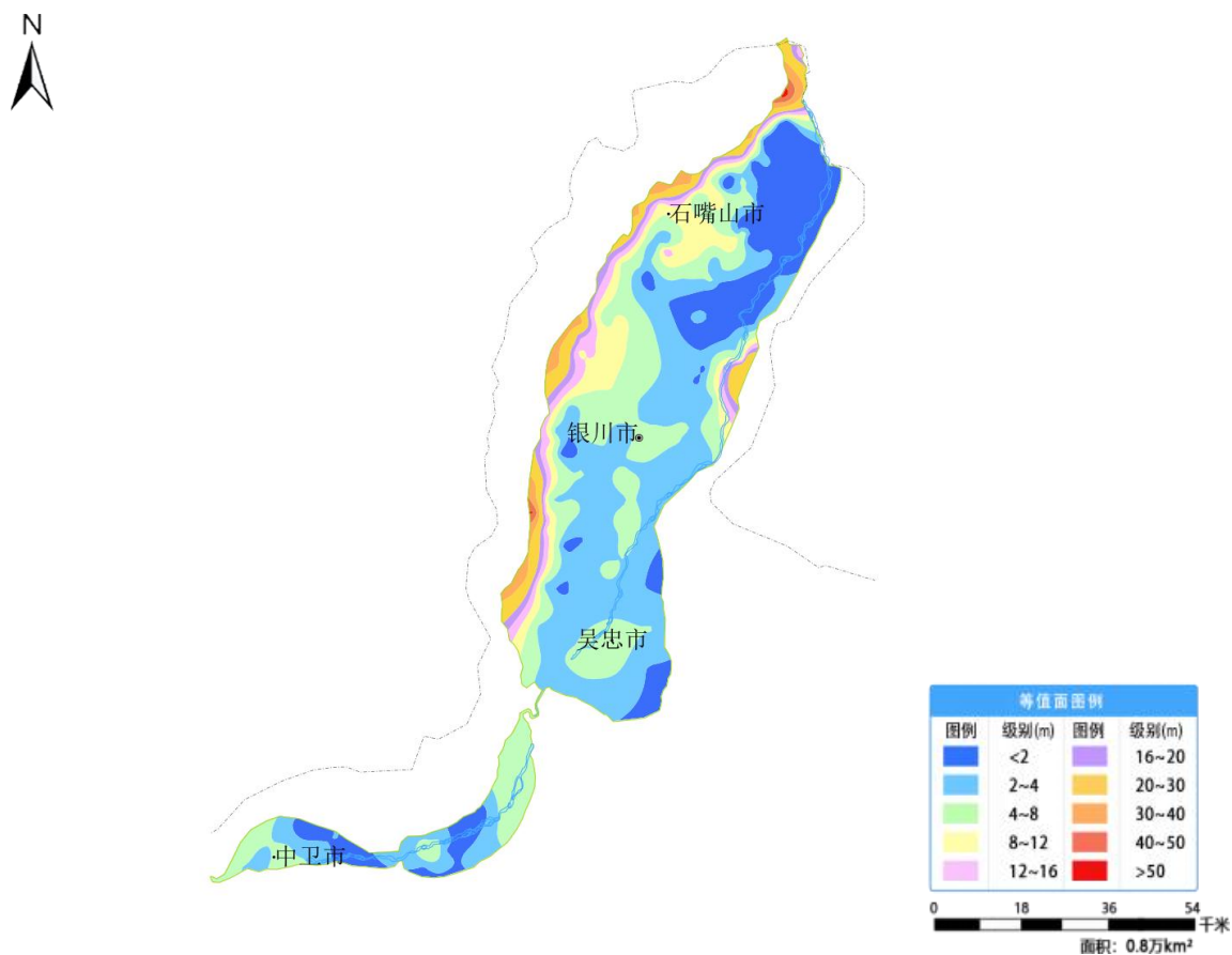
图 25 宁夏银川卫宁平原 8 月份地下水埋深等值面图
