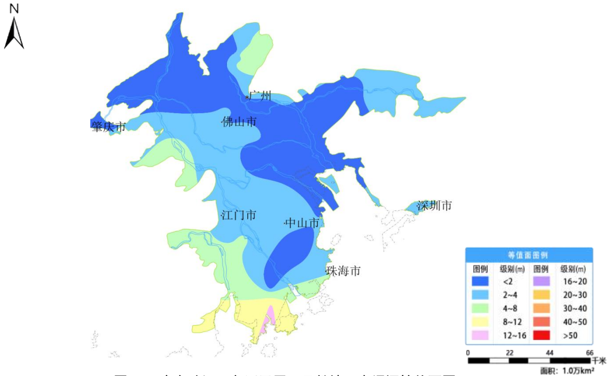
图 33 广东珠江三角洲平原 8 月份地下水埋深等值面图
