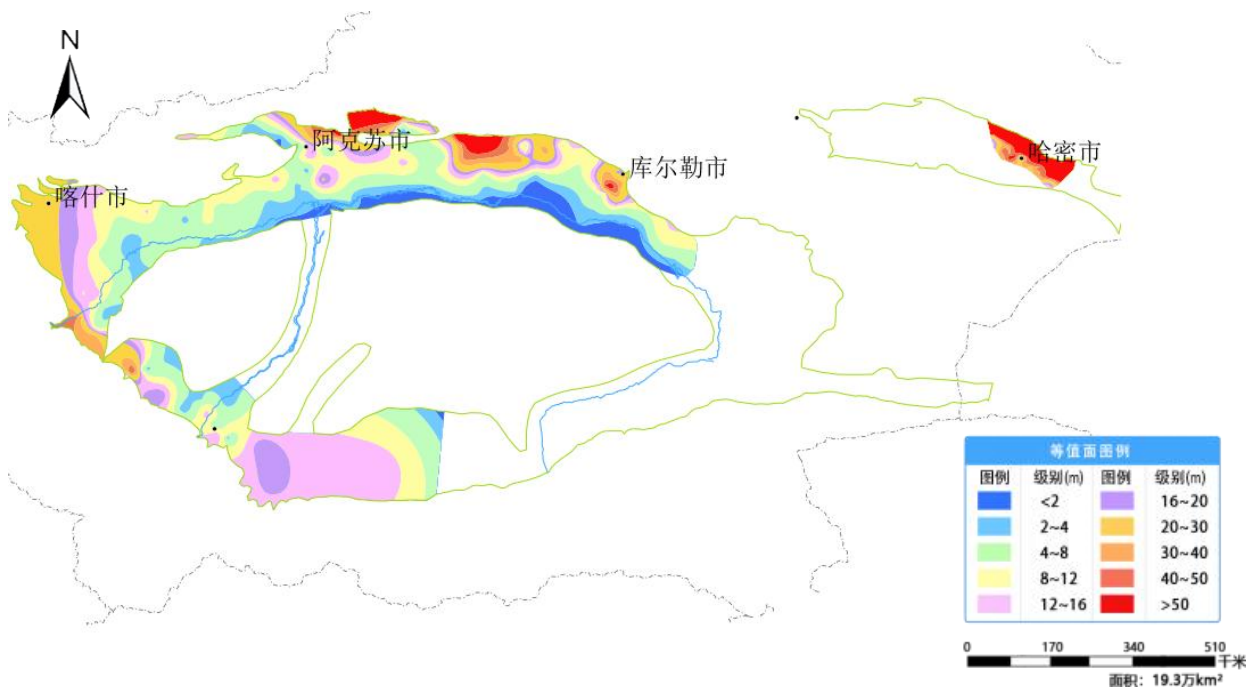
图 27 新疆塔里木盆地监控区 8 月份地下水埋深等值面图
