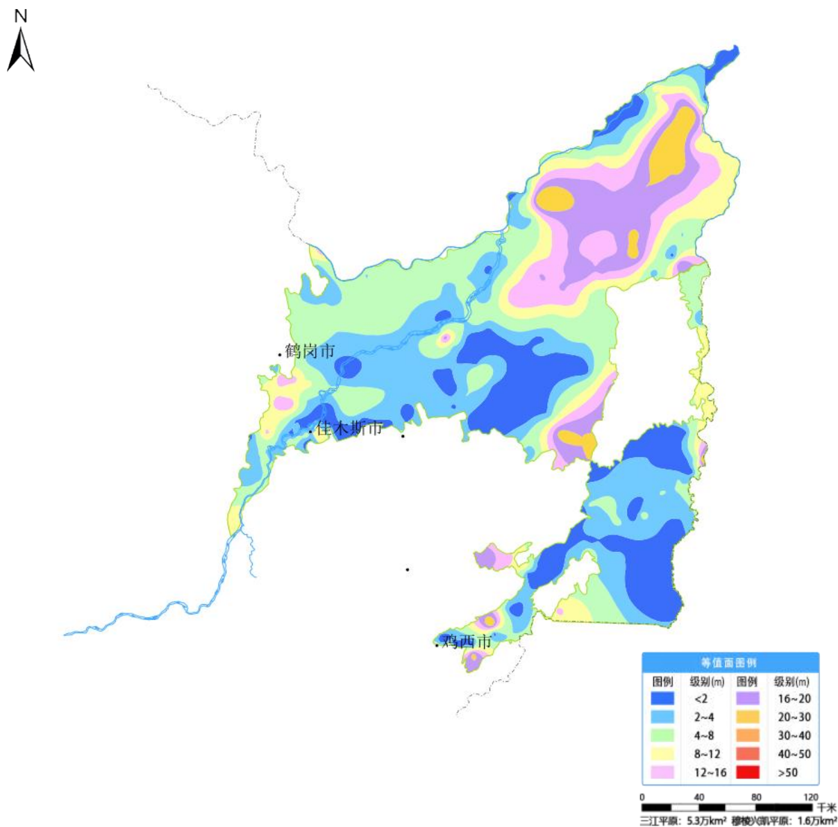
图 1 三江平原和穆棱兴凯平原 8 月份地下水埋深等值面图
