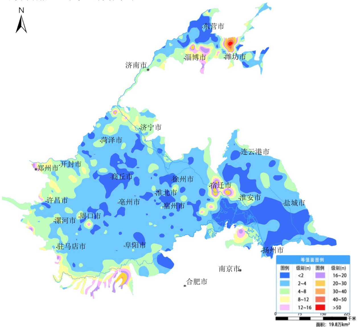
图 13 黄淮平原 12 月份地下水埋深等值面图
