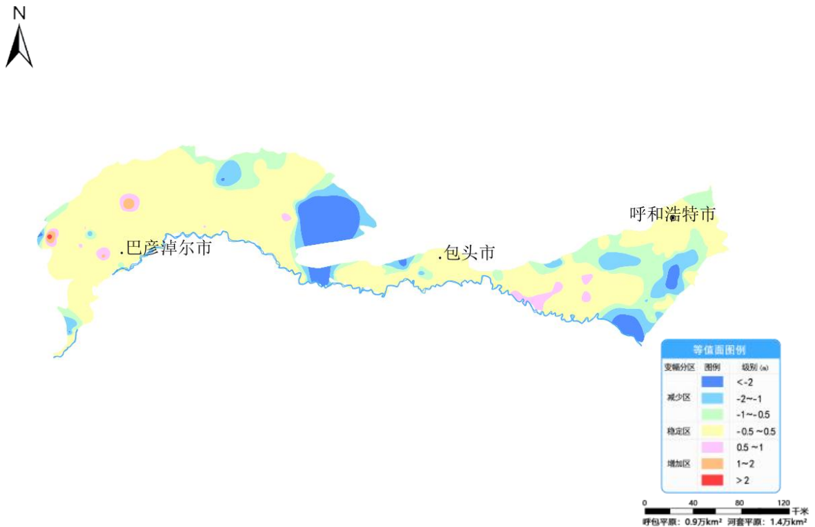
图 17 内蒙古呼包平原及河套平原 12 月份与上月相比地下水埋深变幅图
