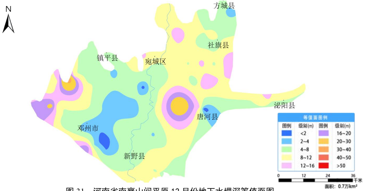
图 31 河南省南襄山间平原 12 月份地下水埋深等值面图
