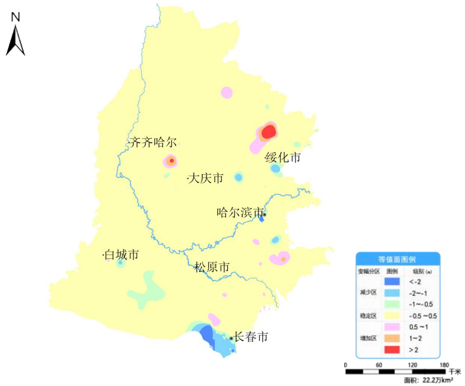
图 5 松嫩平原 12 月份与上月相比地下水埋深变幅图
