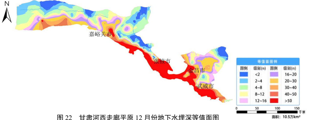
图 22 甘肃河西走廊平原 12 月份地下水埋深等值面图
