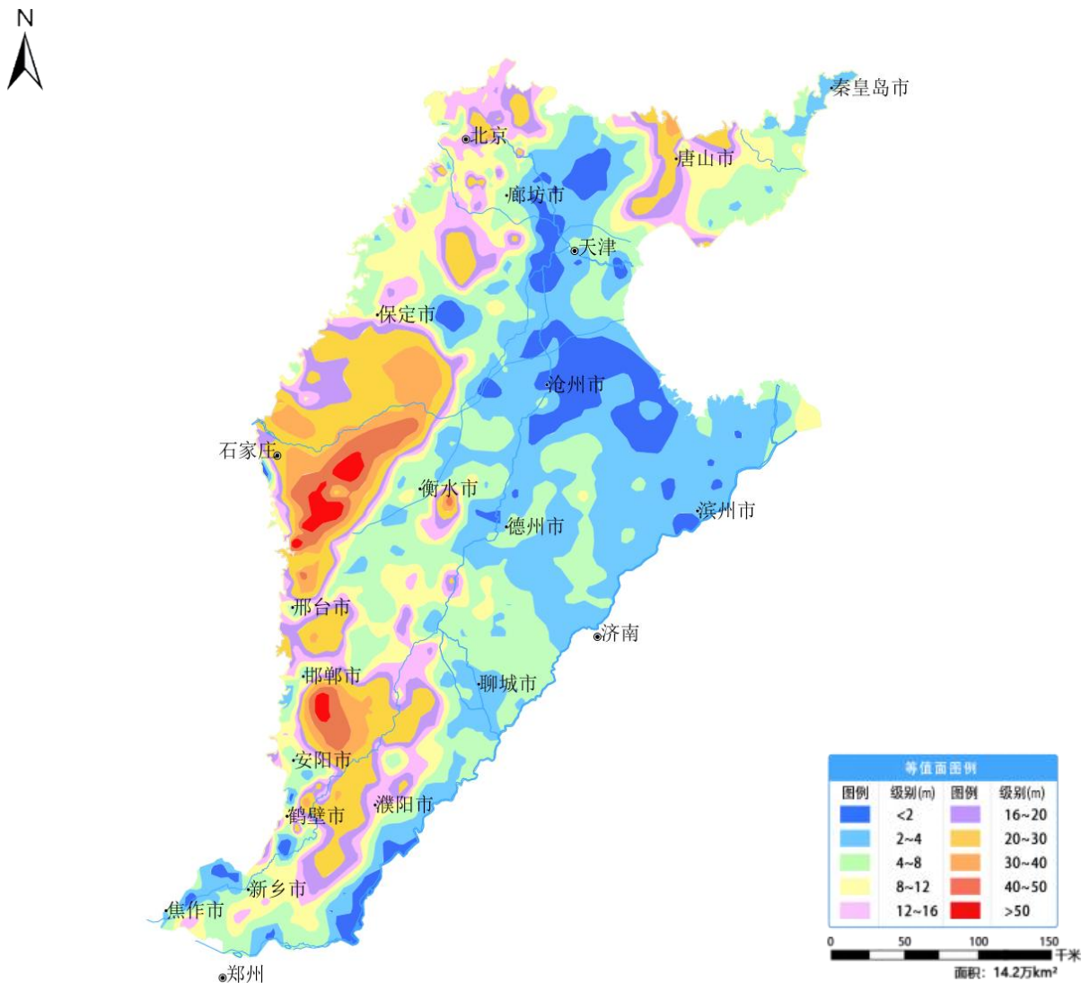
图 10 海河平原 12 月份地下水埋深等值面图
