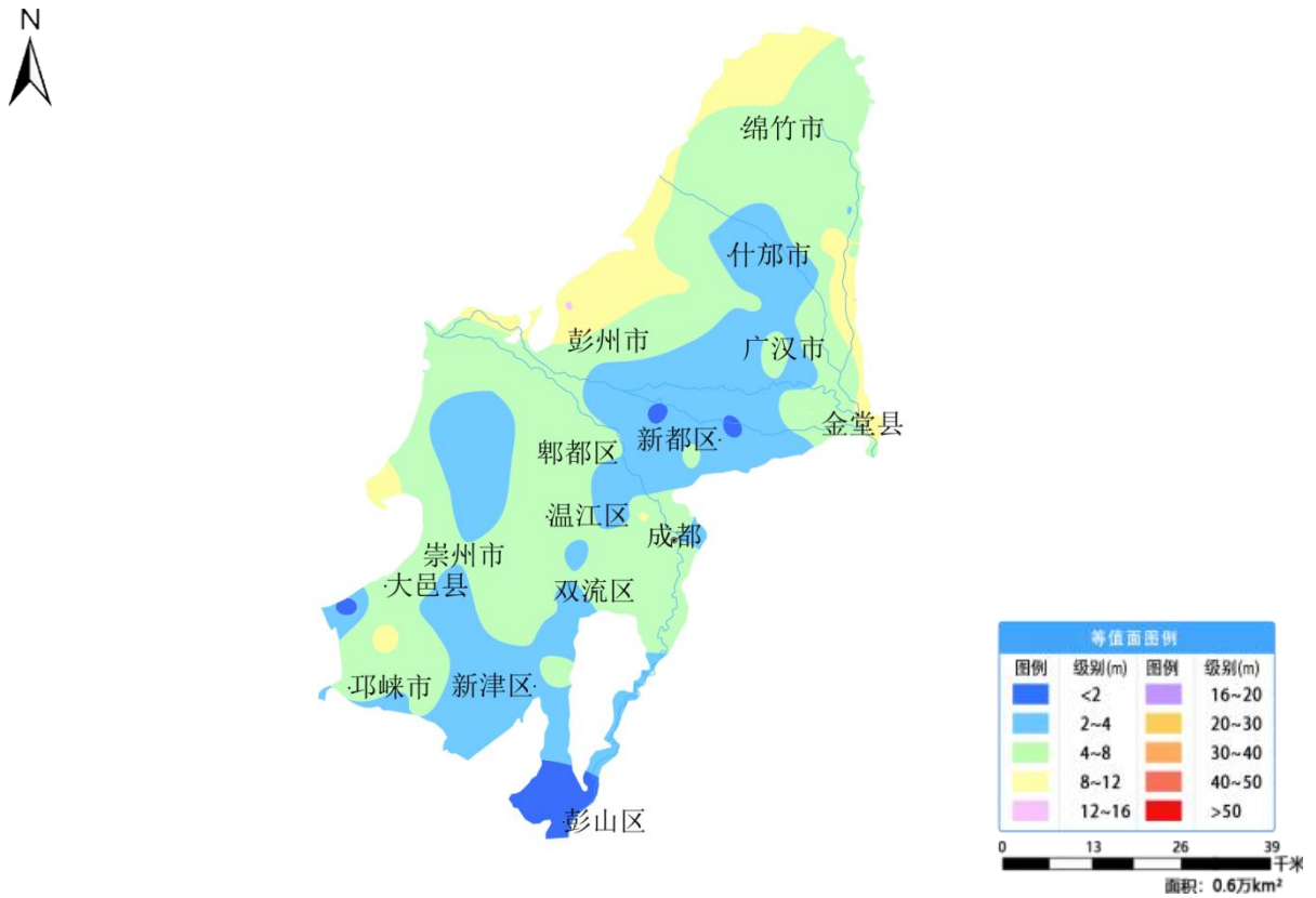
图 32 成都平原 12 月份地下水埋深等值面图
