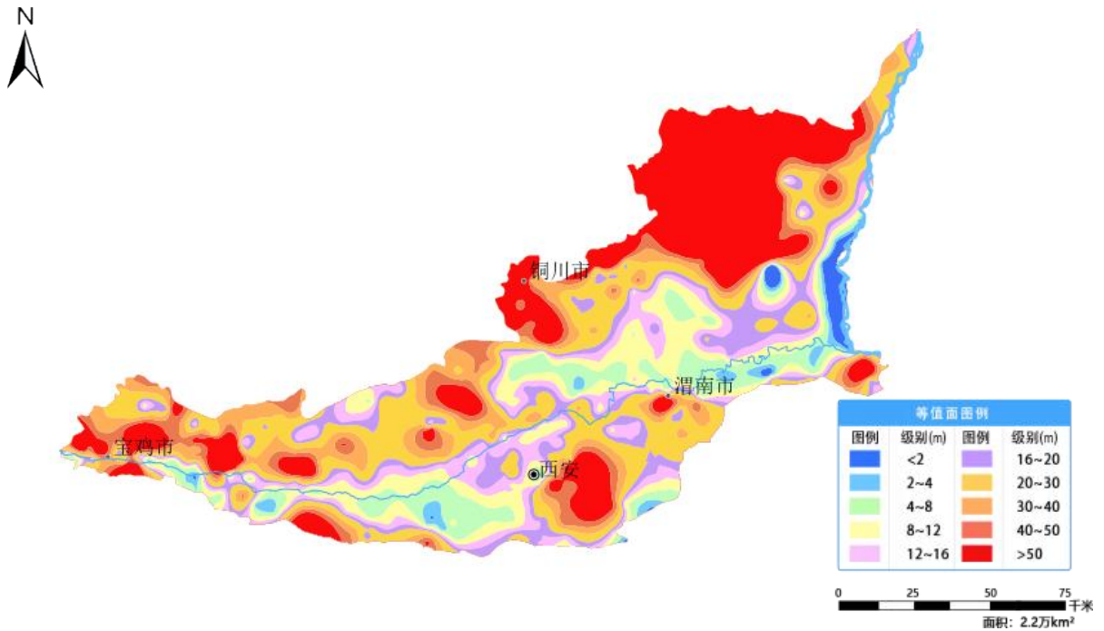
图 19 陕西关中平原 12 月份地下水埋深等值面图
