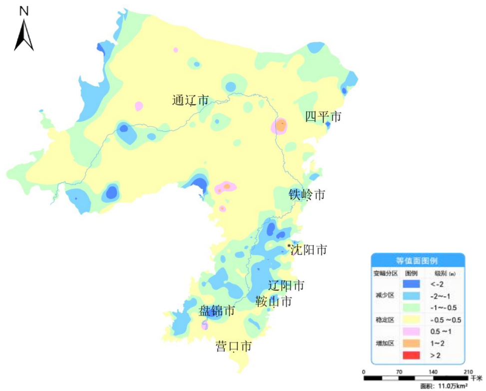
图 9 辽河平原 12 月份与去年同期相比地下水埋深变幅图
