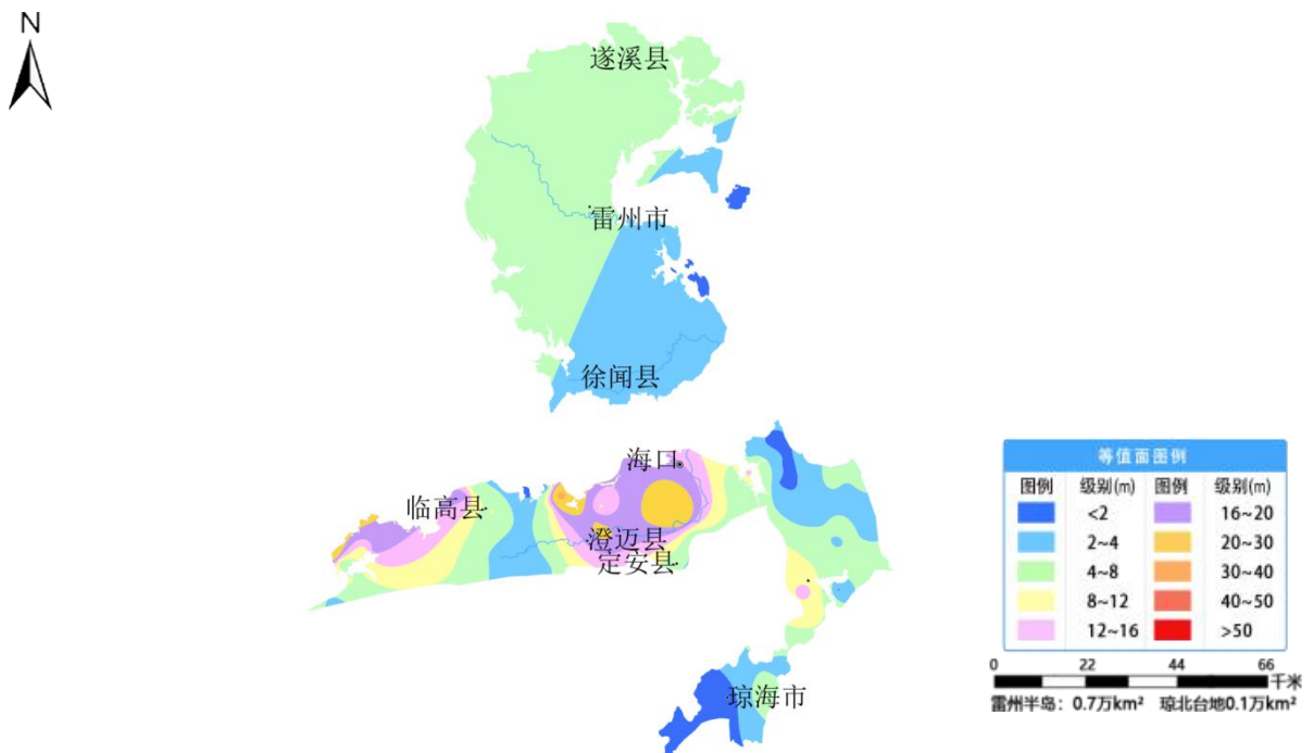
图 34 雷州半岛平原和琼北台地平原 12 月份地下水埋深等值面图
