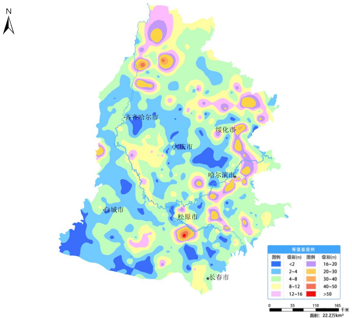
图 4 松嫩平原 12 月份地下水埋深等值面图
