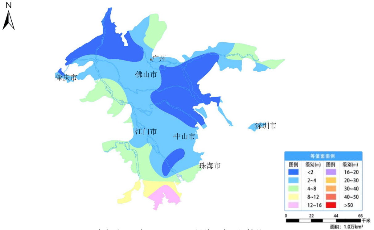
图 33 广东珠江三角洲平原 12 月份地下水埋深等值面图
