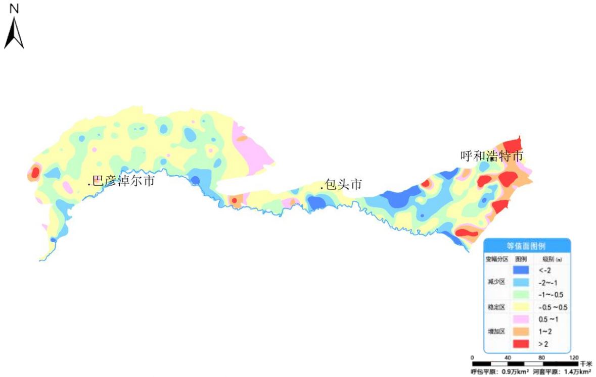
图 18 内蒙古呼包平原及河套平原 12 月份与去年同期相比地下水埋深变幅图
