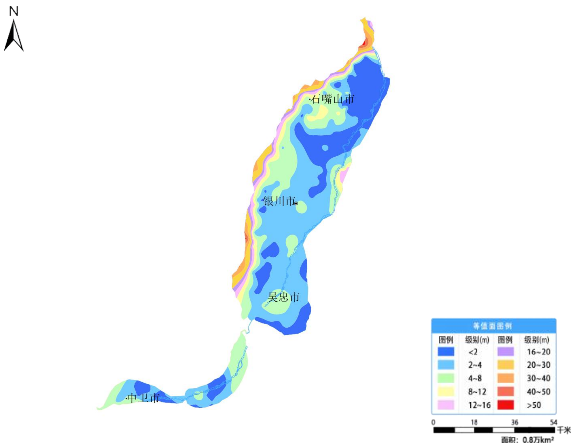
图 25 宁夏银川卫宁平原 12 月份地下水埋深等值面图
