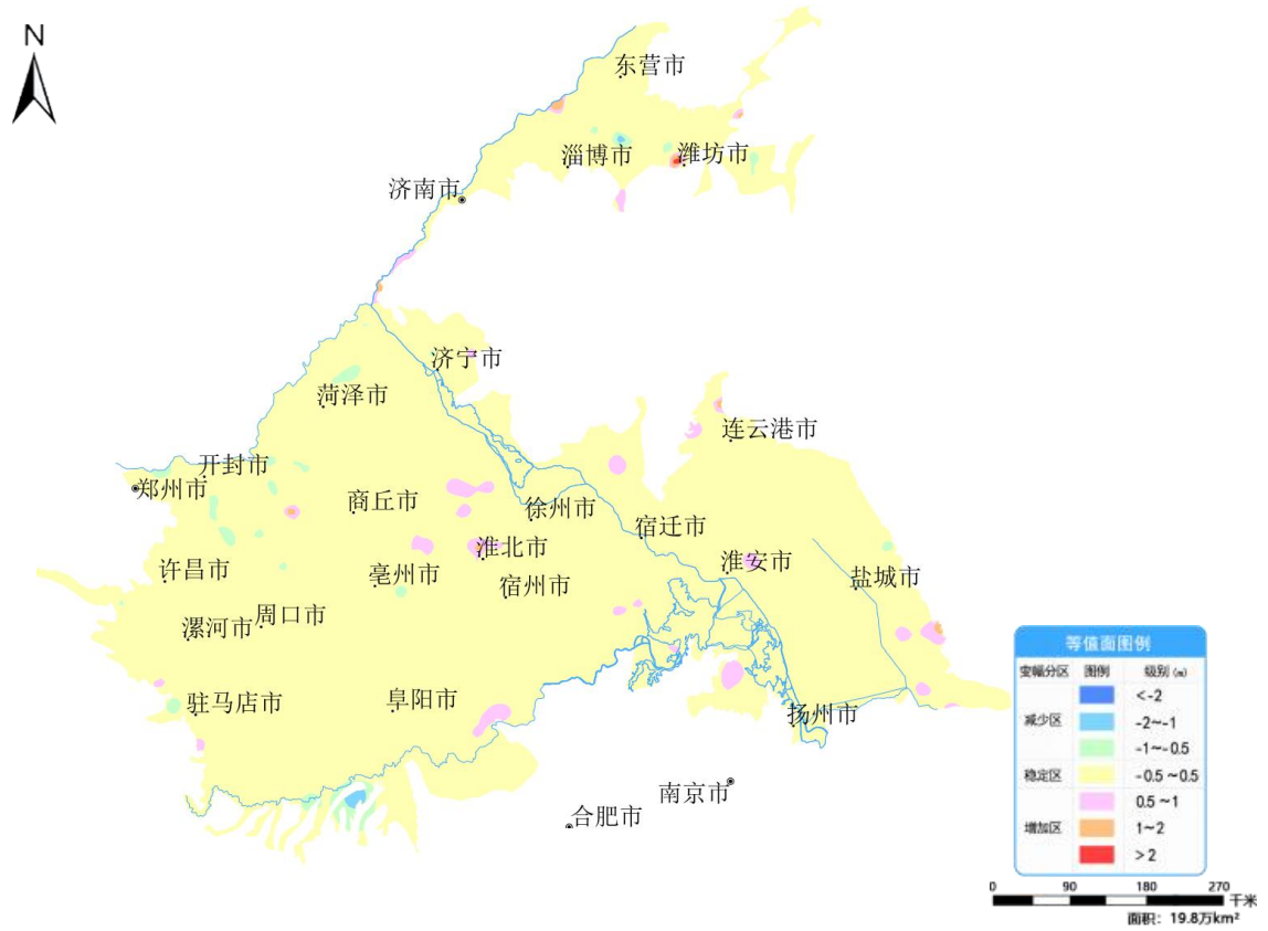
图 14 黄淮平原 12 月份与上月相比地下水埋深变幅图
