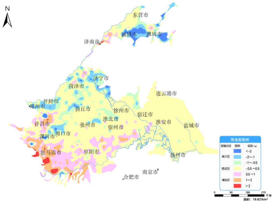
图 15 黄淮平原 12 月份与去年同期相比地下水埋深变幅图
