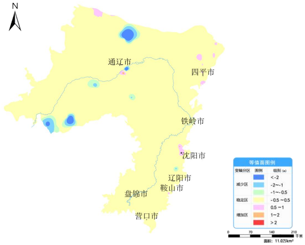
图 8 辽河平原 12 月份与上月相比地下水埋深变幅图
