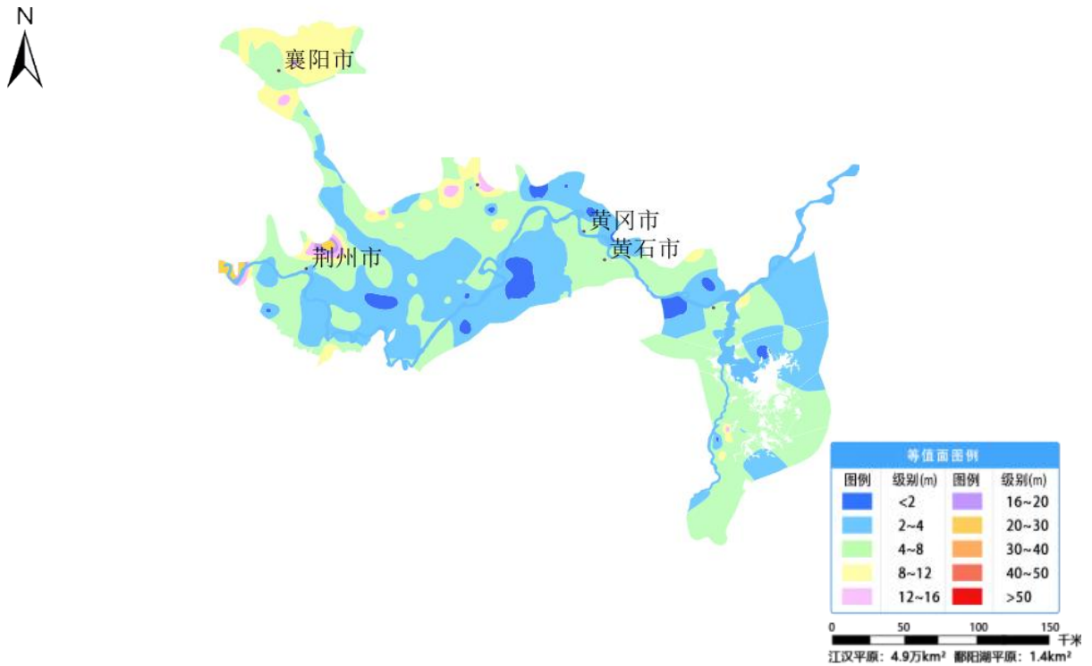
图 29 江汉平原和鄱阳湖平原 12 月份地下水埋深等值面图
