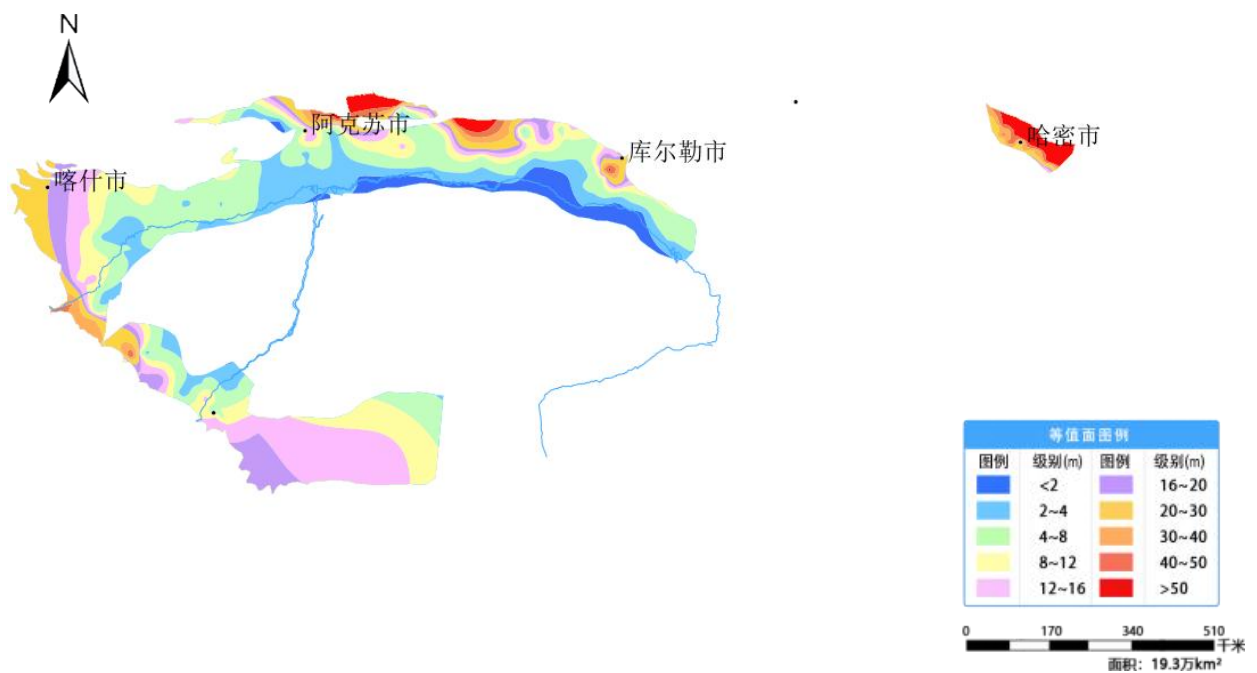
图 27 新疆塔里木盆地监控区 12 月份地下水埋深等值面图
