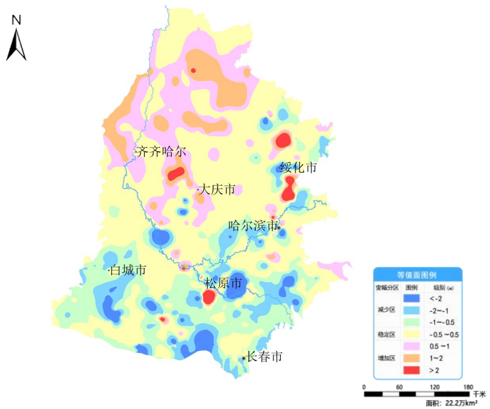
图 6 松嫩平原 12 月份与去年同期相比地下水埋深变幅图
