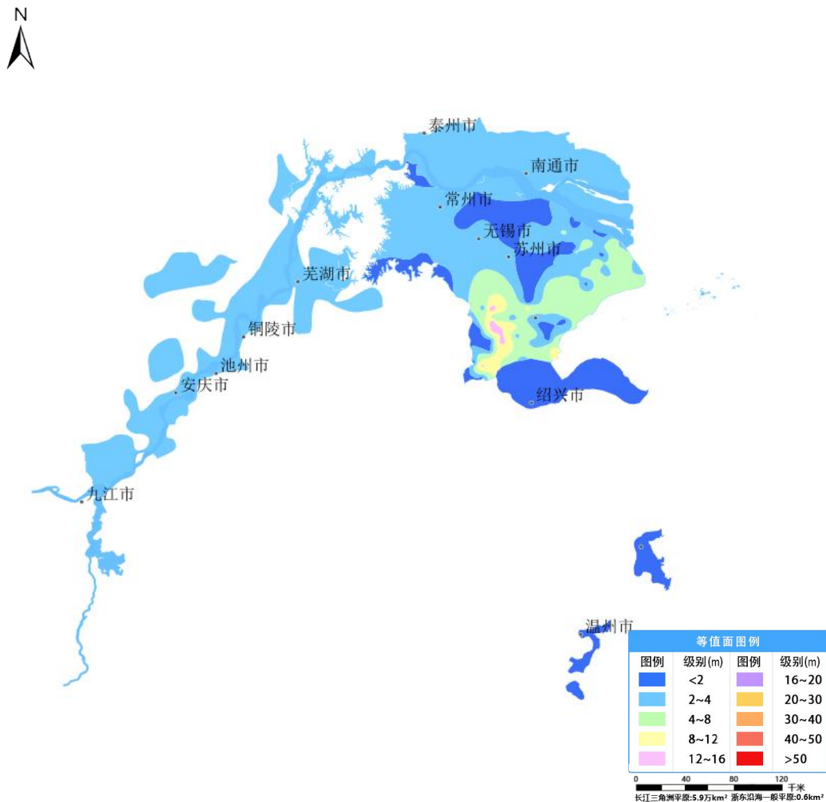
图 30 长江三角洲平原和浙东沿海平原 12 月份地下水埋深等值面图
