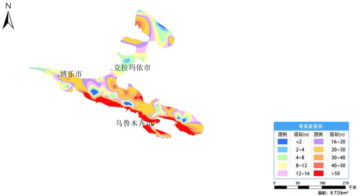
图 28 新疆准噶尔盆地监控区 12 月份地下水埋深等值面图
