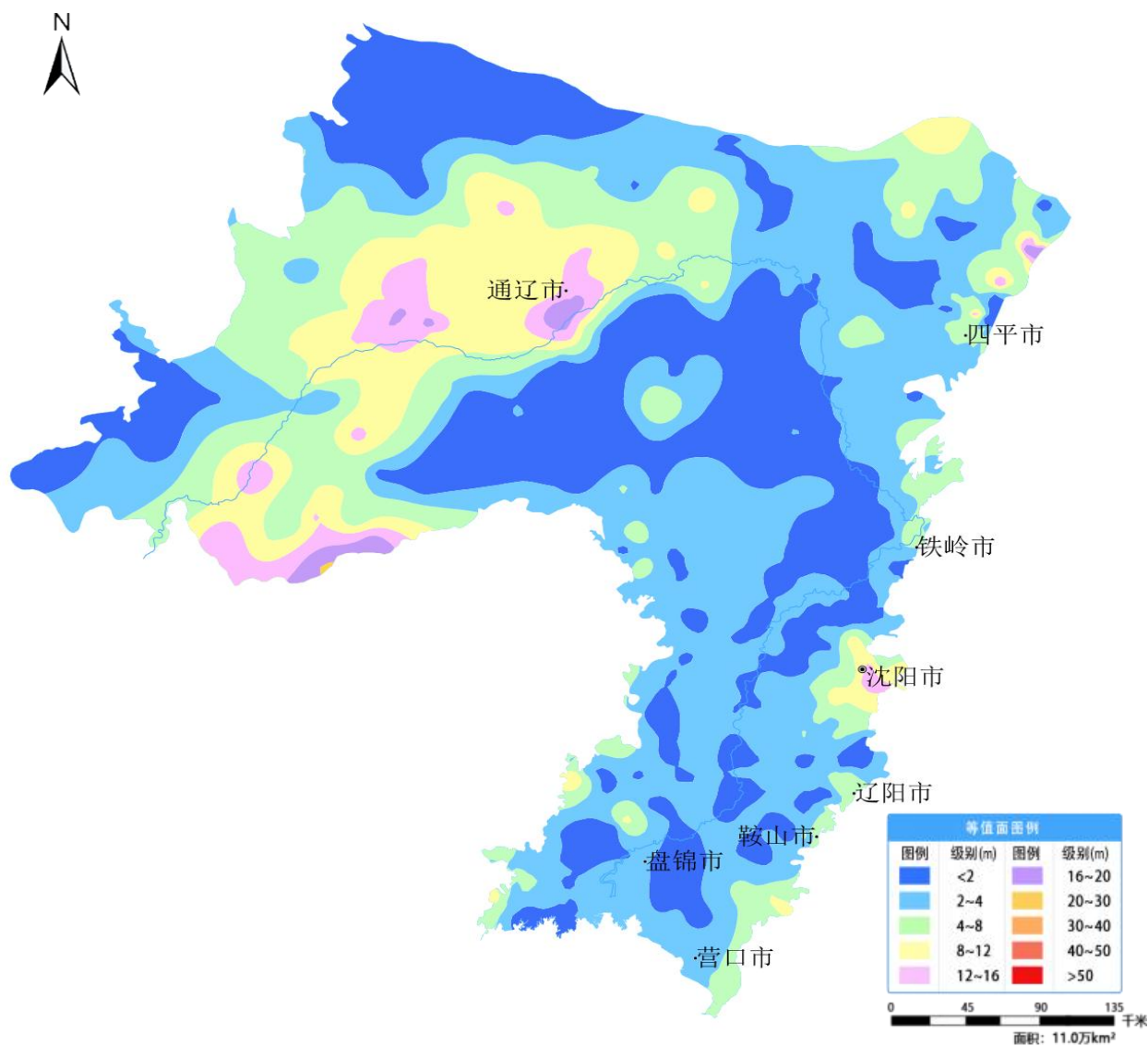
图 7 辽河平原 12 月份地下水埋深等值面图
