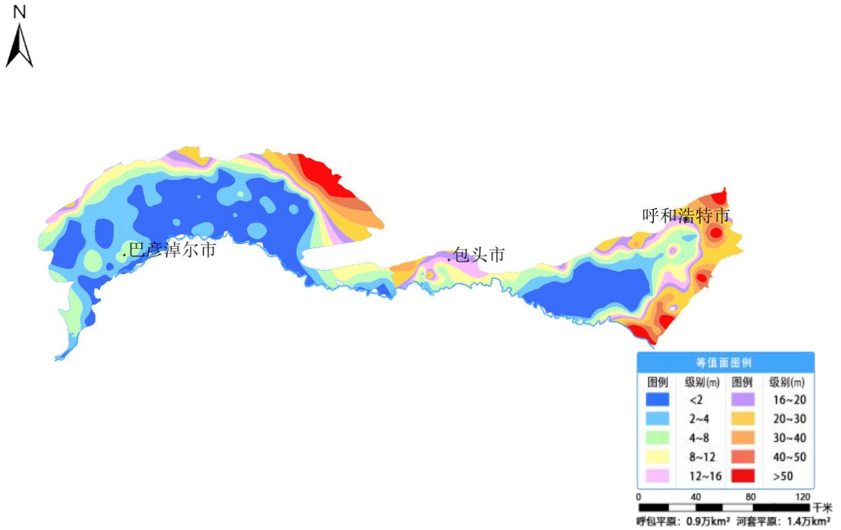
图 16 内蒙古呼包平原及河套平原 12 月份地下水埋深等值面图
